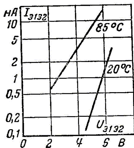
Зависимость динамического сопротивления от тока базы
