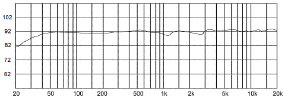
Амплитудно-частотная характеристика
