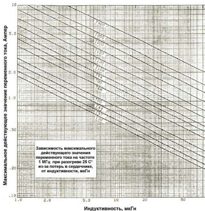
Рисунок 12. Зависимость действующего значения тока в обмотке от индуктивности при частоте 1 МГц и нагрее 25 С°
