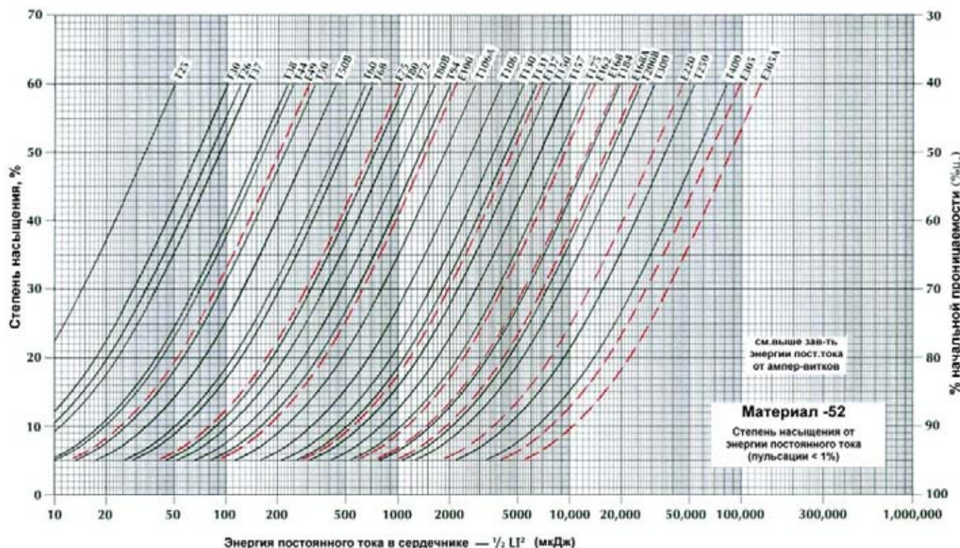
Понятие «степень насыщения» зачастую вызывает вопросы. Например, если проницаемость сердечника составляет 90% от начальной (индуктивность дросселя равна 90% от минимального значения
