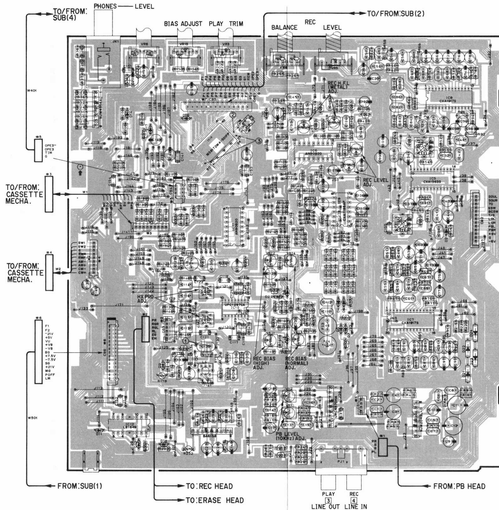
MAIN P. C. B. (1)
