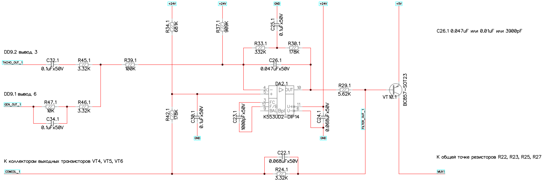
Фильтр (усилитель ошибки), схема вариант 1
