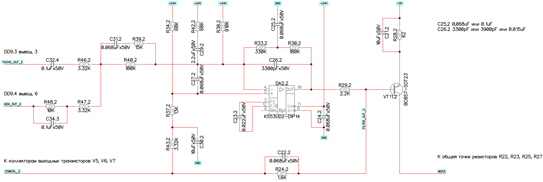
Фильтр (усилитель ошибки), схема вариант 2
