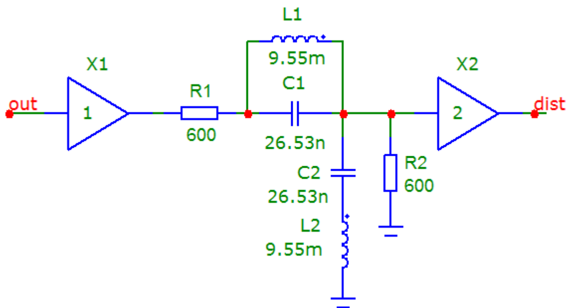
Рис. 3. Режекторный фильтр на частоту 10 кГц
