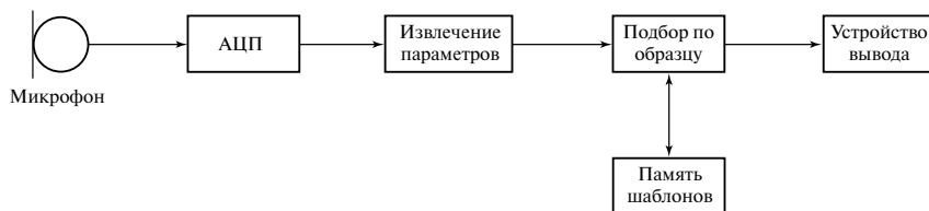
Рис. 1.11. Блок-схема системы распознавания речи
