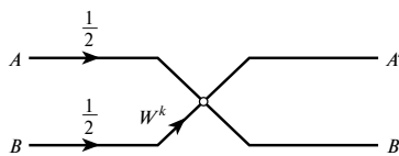
Рис. 13.30. Схема масштабирования для снижения переполнения в каждой “бабочке”
