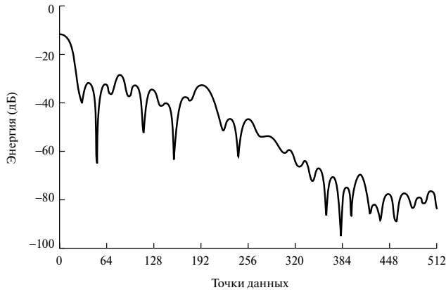
Рис. 11.6. Энергетический спектр при выборке с интервалом 1 с, весовая функция Кайзера–Бесселя, 64 информационные точки, 1024-точечное БПФ
