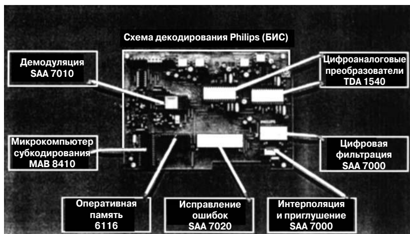
Рис. 1.15. Печатная плата декодирующей схемы проигрывателя компакт-дисков фирмы Philips. (Перепечатано с разрешения журнала Philips Technical Review , 40(6), 1982)
