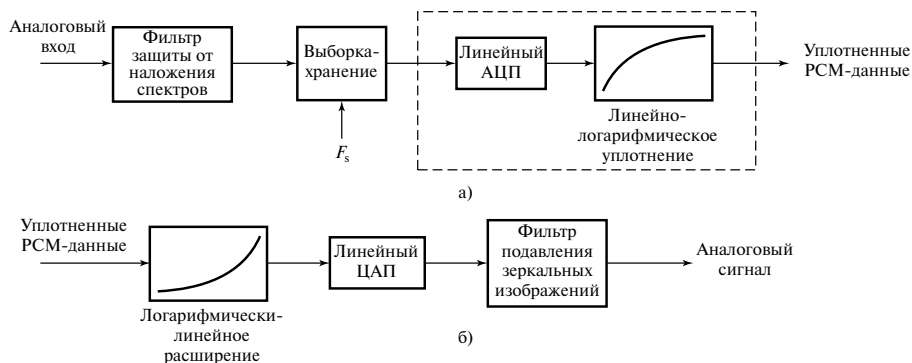
Рис. 2.26. Неоднородные аналого-цифровые и цифроаналоговые преобразования
