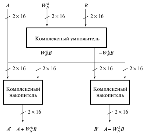
Рис. 12.40. Схема аппаратного процессора для вычисления "бабочки" с использованием отдельных блоков комплексной арифметики
