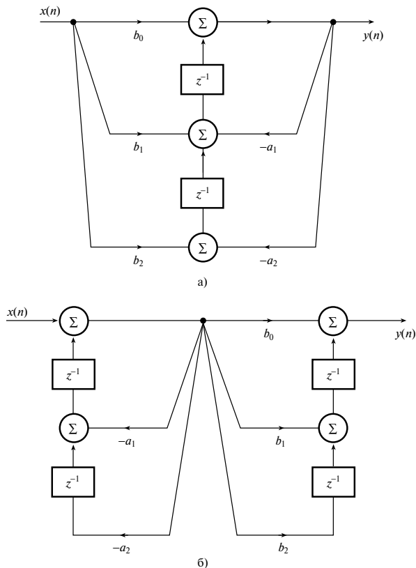
Рис. 8.26. Переупорядоченное каноническое звено второго порядка (панель а); переупорядоченное звено второго порядка в прямой реализации (панель б)
