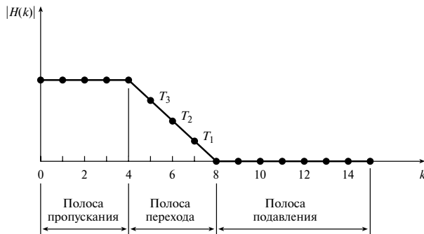
Рис. 7.19. Частотные выборки фильтра нижних частот, включая три выборки в полосе перехода. Примечание: поскольку амплитудная характеристика симметрична, показана только половина характеристики фильтра
