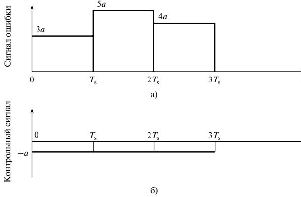
Рис. 5.34. Контроль за положением космического аппарата: а) сигнал ошибки; б) контрольный сигнал
