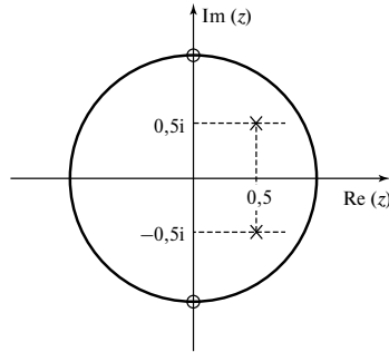
Рис. 4.7. Диаграмма нулей и полюсов для примера 4.10, п. 2
