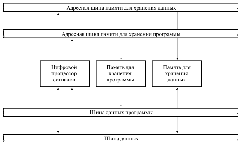
Рис. 12.4. Стандартная гарвардская архитектура с отдельными областями памяти для хранения данных и программы. Вызов команд данных и команд программы может выполняться одновременно, поскольку используются две независимые памяти
