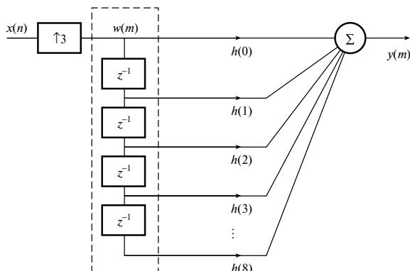
Рис. 9.20. Интерполятор 1:3 с 9-точечным КИХ-фильтром, реализованным в прямой форме
