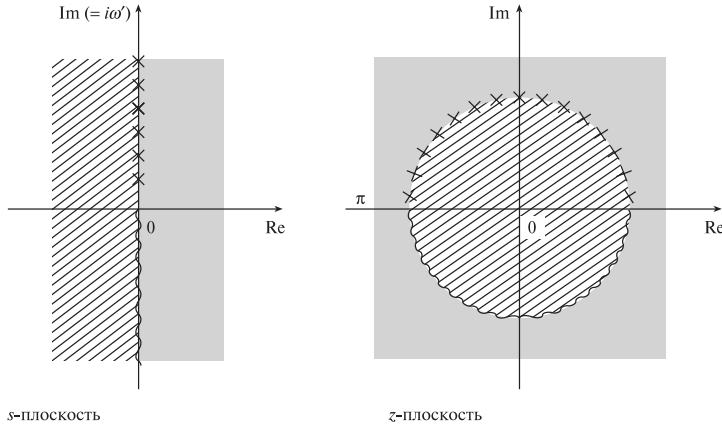
Рис. 8.9. Иллюстрация отображения с s -плоскости на комплексную ( z ) плоскость с использованием билинейного z -преобразования. Обратите внимание на то, что положительная часть оси i\omega' на s -плоскости (т.е. точки от s = 0 до s = i\infty ) отображается в верхнюю половину единичной окружности, а отрицательная часть оси i\omega' переводится в нижнюю половину
