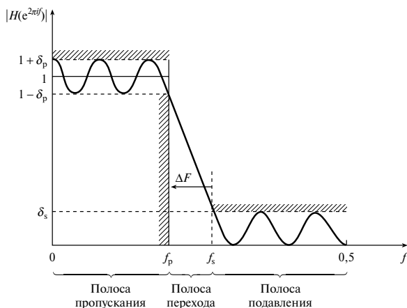
Рис. 7.3. Спецификация амплитудно-частотной характеристики фильтра нижних частот. Отклонения в полосах пропускания и подавления часто выражаются в децибелах: отклонение в полосе пропускания равно 20 \lg(1 + \delta_p) дБ; отклонение в полосе подавления равно -20 \lg(\delta_s) дБ
