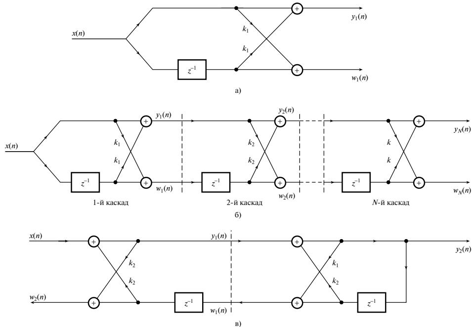
Рис. 6.8. Стандартная решетчатая структура (панель а). N -каскадный КИХ-фильтр с решетчатой структурой (панель б). Двухкаскадная решетчатая структура БИХ-фильтра с заданными всеми полюсами (панель в)
