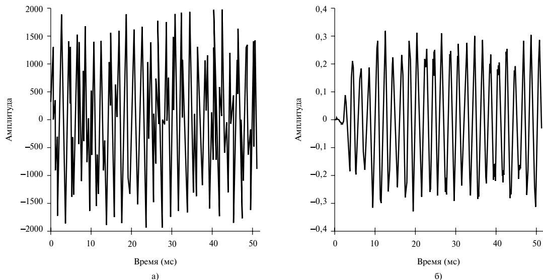
Рис. 10А.2. Адаптивное выделение узкополосного сигнала: а) зашумленный сигнал; б) выделенный сигнал
