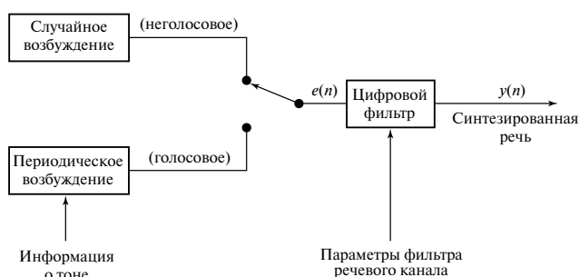
Рис. 1.9. Линейное кодирование речи с предсказанием
