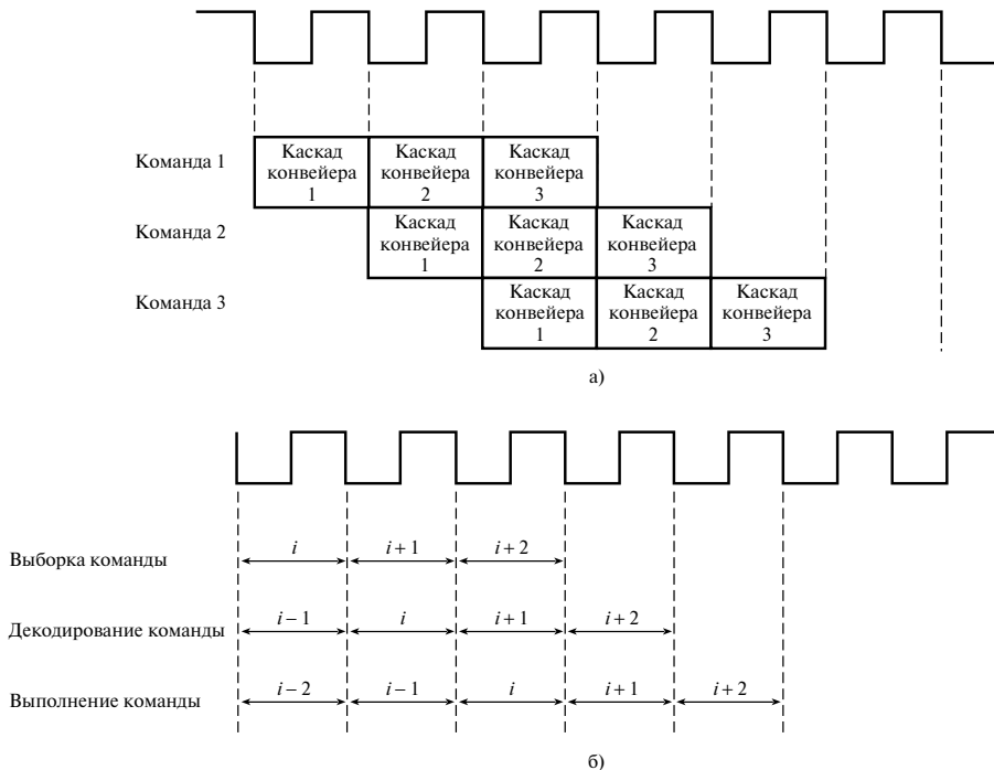
Рис. 12.6. Иллюстрация концепции конвейерной обработки
