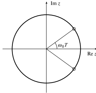
Рис. 7.39. Диаграмма нулей и полюсов для задачи 7.15; \omega_0 T = \pi/5 радиан
