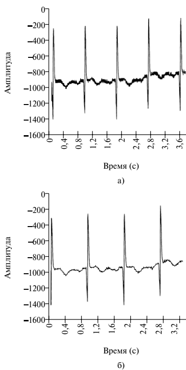
Рис. 9.36. Необработанные ЭКГ-данные (панель а ); ЭКГ-данные после децимации (выровнены с учетом задержки) (панель б )
