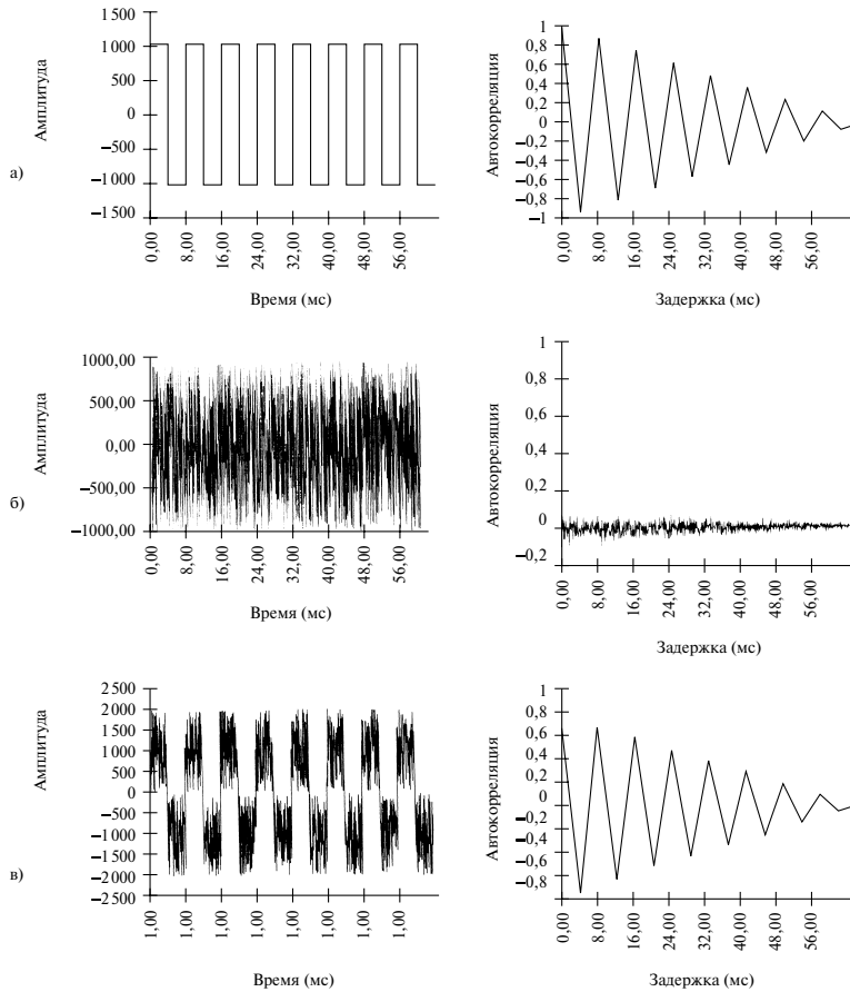
Рис. 1.2. Автокорреляция: а) периодического сигнала, б) шума; в) периодического сигнала с шумом. Обратите внимание на то, что на панели в периодический характер сигнала, скрытого за шумом, все еще заметен; по этой причине автокорреляцию часто используют для выявления скрытой периодичности
