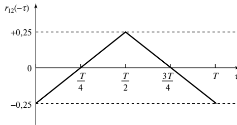
Рис. 5.9. Величина r_{12}(-\tau) как функция \tau
