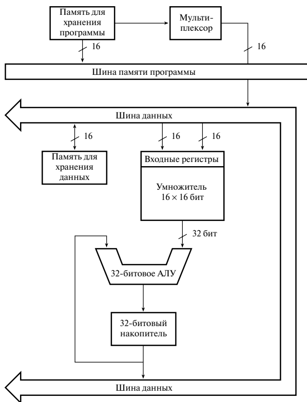
Рис. 12.15. Упрощенная архитектура процессора ЦОС с фиксированной запятой первого поколения (Texas Instruments TMS320C10)
