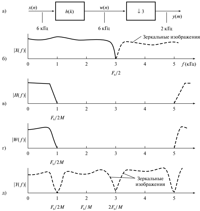
Рис. 9.2. Спектральная интерпретация децимации сигнала с частоты 6 до частоты 2 кГц. Если бы не цифровой фильтр, на сигнал наложился бы зеркальные компоненты
