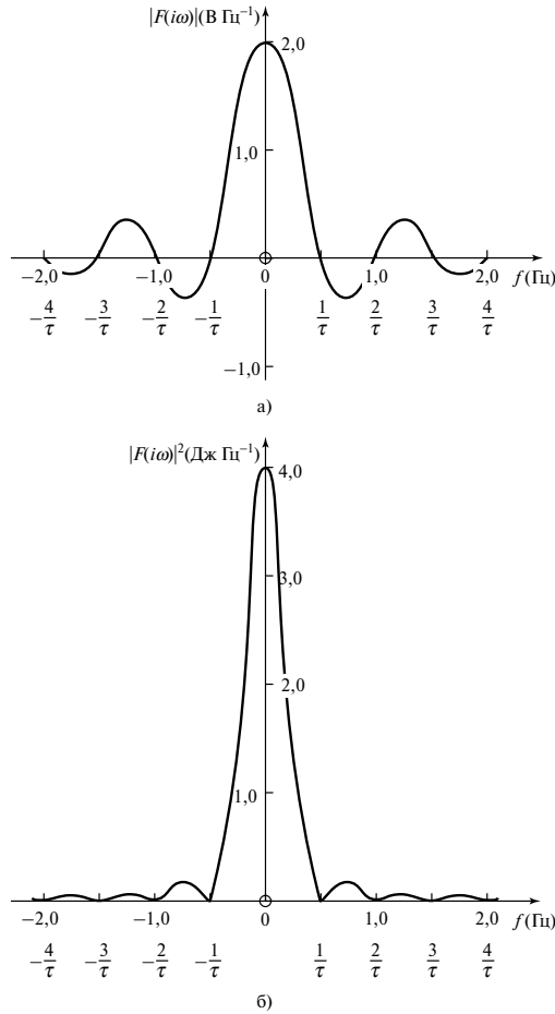
Рис. 3.2. Импульс 2 В: а) амплитудный спектр; б) энергетический спектр
