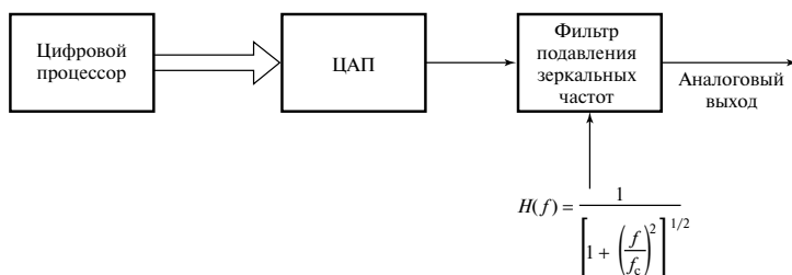
Рис. 2.58. Выходной каскад системы ЦОС реального времени
