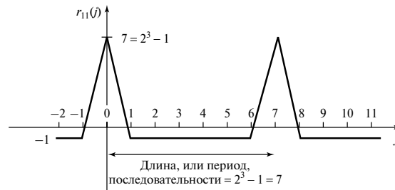
Рис. 5.16. Автокорреляционная функция биполярного сигнала трехкаскадного генератора псевдослучайной последовательности
