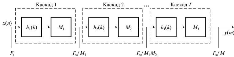
Рис. 9.8. Процесс многокаскадной децимации
