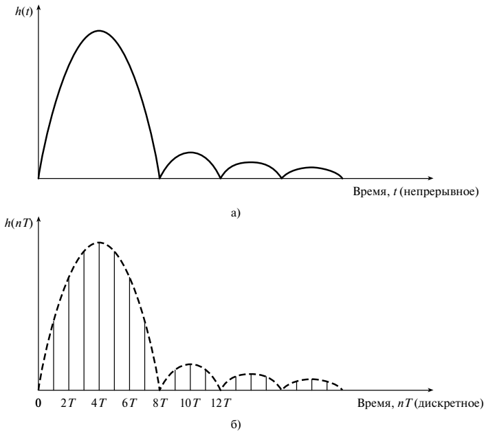
Рис. 8.7. Сравнение импульсной характеристики а) аналогового фильтра h(t) и б) эквивалентного цифрового фильтра h(nT) . В методе инвариантного преобразования импульсной характеристики две характеристики идентичны в моменты взятия выборок
