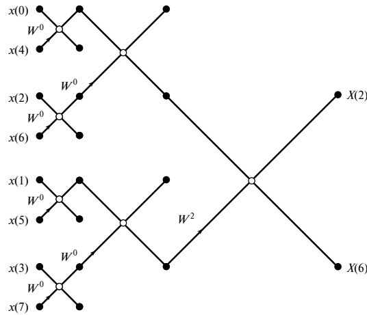
Рис. 13.29. Граф-схема, на которой показаны “бабочки”, вносящие вклад в шум округления, присутствующий в выходах X(2) и X(6)
