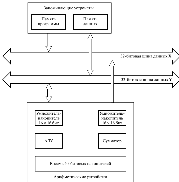
Рис. 12.22. Упрощенная архитектура процессора ЦОС с фиксированной запятой третьего поколения (Lucent Technologies DSP16000)
