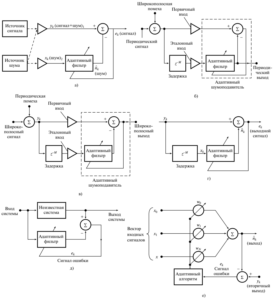
Рис. 10.3. Некоторые конфигурации адаптивного фильтра (согласно [10]): а) адаптивный шумоподавитель; б) адаптивный самонастраивающийся фильтр; в) подавление периодической помехи без внешнего эталонного источника; г) адаптивный селективный фильтр; д) моделирование системы; е) подбор линейной комбинации
