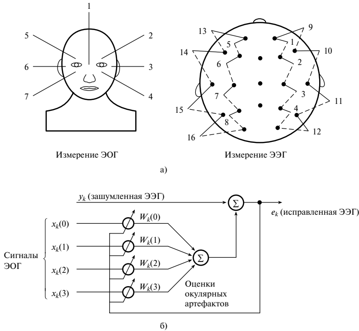
Рис. 10.17. Метод адаптивного устранения окулярных артефактов: а) возможные положения электродов при снятии электроокулограммы и электроэнцефалограммы; б) адаптивный фильтр окулярных артефактов
