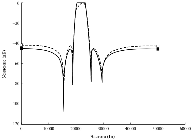
Рис. 13.6. Практическое влияние квантования коэффициентов на частотную характеристику: ■ — неквантованные коэффициенты; □ — коэффициенты квантованы до 5 бит
