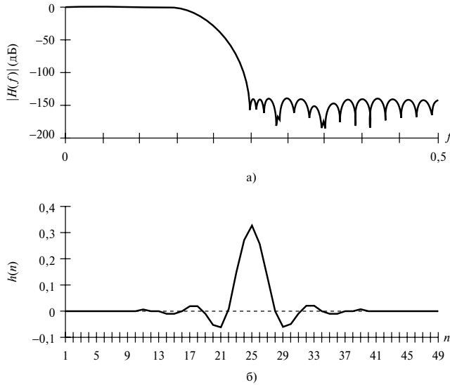
Рис. 7.21. Интерполированная частотная характеристика (панель а); коэффициенты фильтра (панель б). Неравномерность в полосе пропускания — 0,046 дБ; затухание в полосе подавления — 139,64 дБ; ширина полосы пропускания — 0,15; пять выборок в полосе перехода; 49 коэффициентов фильтра. Значения выборок в полосе перехода — 0,855456; 0,485507; 0,148961; 0,019693; 0,000644
