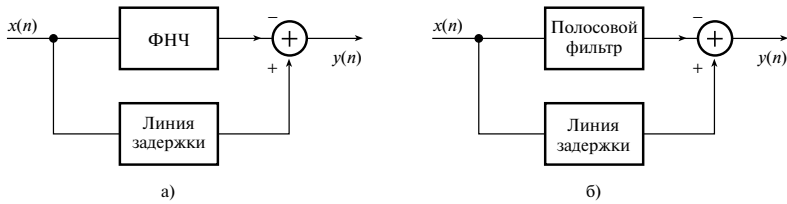
Рис. 9.34. Реализация с обработкой при нескольких скоростях фильтра нижних частот и режекторного фильтра как дуальных к фильтру нижних частот и полосовому фильтру: а) фильтр верхних частот; б) режекторный фильтр
