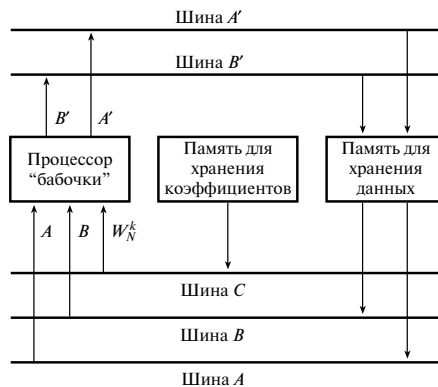
Рис. 12.41. Упрощенная архитектура аппаратного процессора БПФ. Контроллер и генератор адресов не показаны
