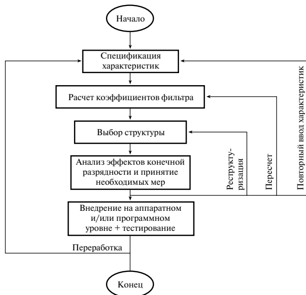
Рис. 8.1. Этапы разработки цифровых фильтров
