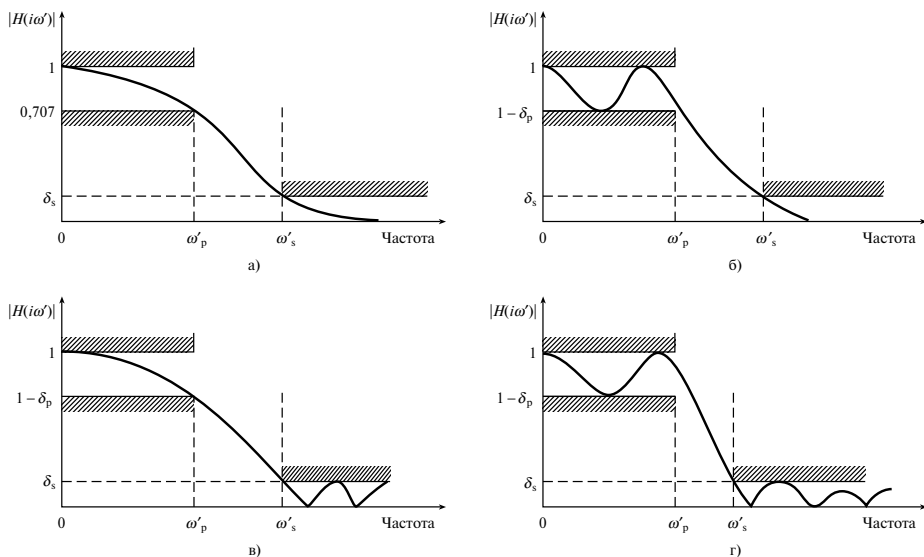
Рис. 8.12. Схематические частотные характеристики некоторых классических аналоговых фильтров: а) фильтр Баттерворта; б) фильтр Чебышева I типа; в) фильтр Чебышева II типа; г) эллиптический фильтр
