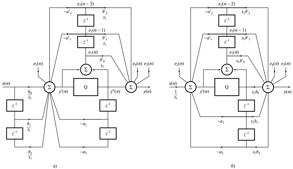
Рис. 13.24. Обобщенные схемы снижения шума: a — фильтр, реализованный в прямой форме; б — канонический фильтр
