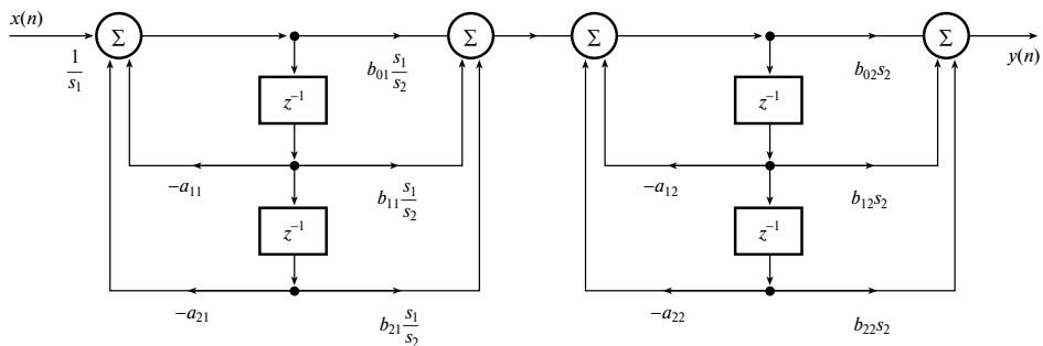
Рис. 8.31. Диаграмма реализации фильтра из раздела 8.16
