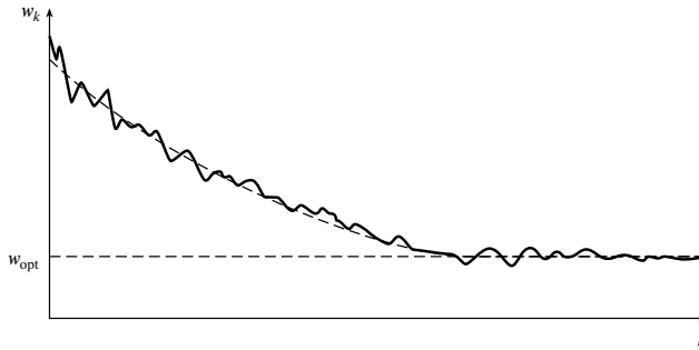
Рис. 10.7. Изменение весовых коэффициентов фильтра
