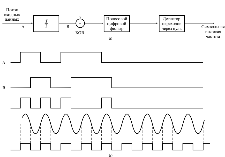
Рис. 8.41. Иллюстрация принципов восстановления символьной тактовой частоты в сфере передачи данных
