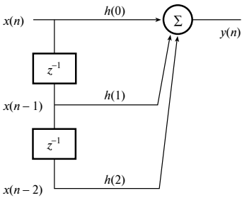
Рис. 14.23. Простой трехточечный КИХ-фильтр
