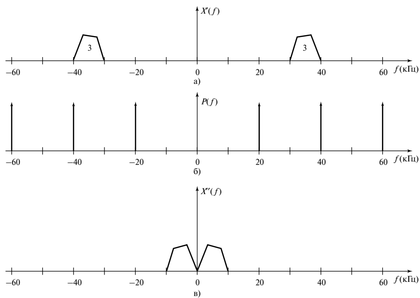
Рис. 2.20. Выход полосового фильтра (панель а ); функция дискретизации (панель б ); выход устройства дискретизации для канала 3 (панель в ) (пример 2.6)
