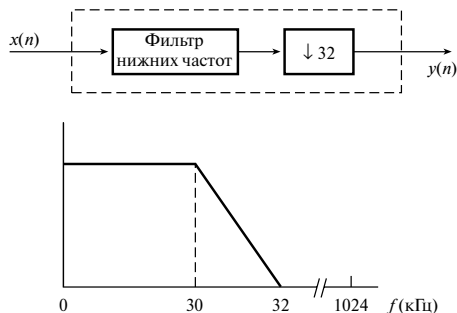
Рис. 9.7. Однокаскадный дециматор из примера 9.1
