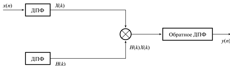
Рис. 7.30. Иллюстрация быстрой свертки
