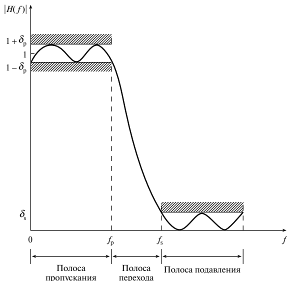
Рис. 6.4. Схема допусков для фильтра нижних частот
