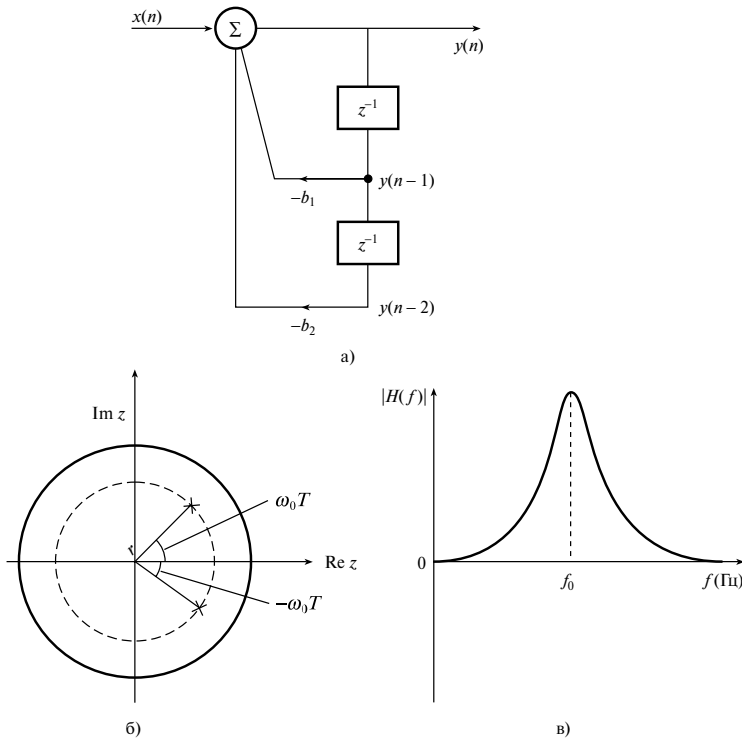
Рис. 8.42. Структура БИХ-фильтра для восстановления символьной тактовой частоты (панель а); диаграмма полюсов (панель б); спектр фильтра (панель в)
