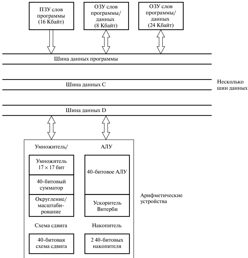
Рис. 12.20. Упрощенная архитектура процессора ЦОС с фиксированной запятой третьего поколения (Texas Instruments TMS320C54x)
