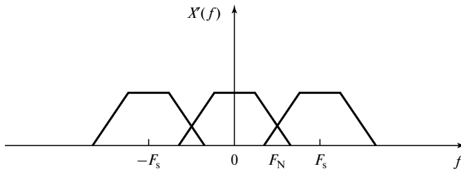
Рис. 2.6. Спектр сигнала, прошедшего процесс дискретизации, на котором показано наложение. Сигналы в области наложения не поддаются восстановлению. F_N равно половине частоты дискретизации и обычно называется частотой Найквиста . Чтобы восстановить все компоненты сигнала, нужно провести выборку с частотой, превышающей удвоенную частоту самого высокочастотного компонента (или равной ей)
