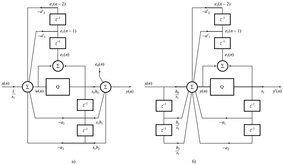
Рис. 13.25. Две различные структуры реализации БИХ-фильтра второго порядка
