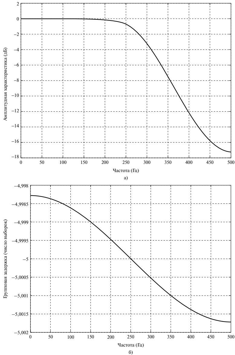
Рис. 8.19. Амплитудно-частотная характеристика инвариантного преобразования импульсной характеристики (панель а ); групповая задержка фильтра, полученного методом инвариантного преобразования импульсной характеристики (панель б )
