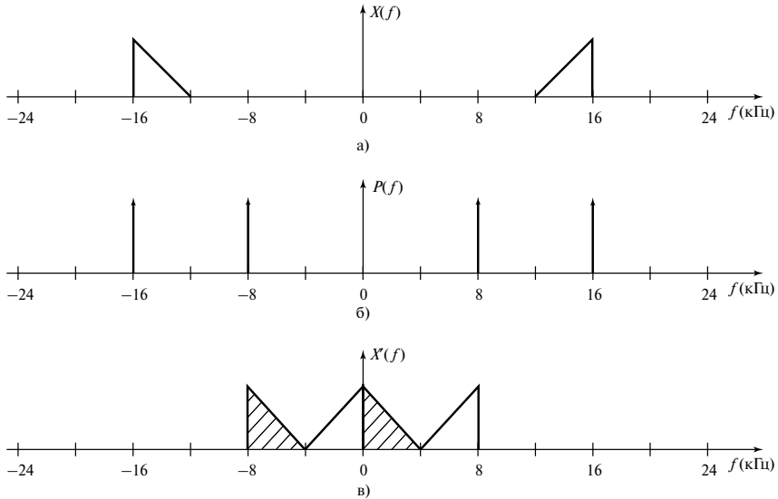
Рис. 2.22. Спектр дискретного сигнала для четных целых n ( n = f_H/B = 4 ) (пример 2.7, вариант 1)
