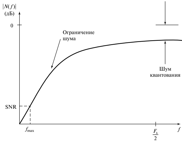
Рис. 2.34. Влияние схемы формирования спектра шума на шум квантования
