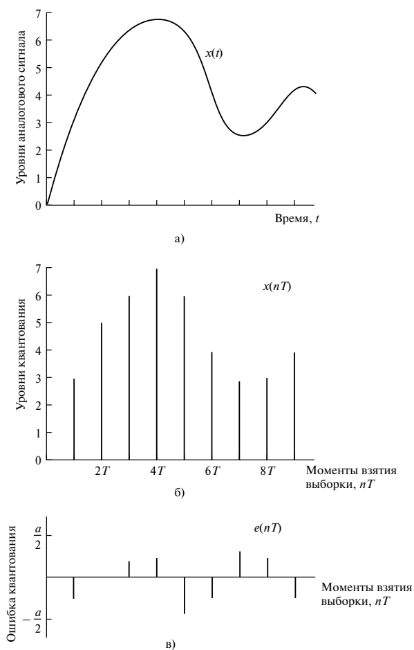
Рис. 2.25. Квантование выборок аналогового сигнала. Для нахождения ошибок квантования на панели в из квантованных выборок (3-битовое устройство квантования; панель б ) сигнала вычитаются выборки сигнала (панель а )
