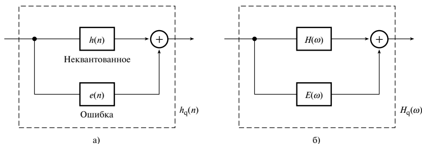
Рис. 7.32. Квантование коэффициентов: а) влияние на коэффициенты импульсной характеристики; б) влияние на частотную характеристику фильтра
