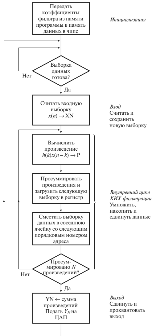
Рис. 12.25. Функциональная схема КИХ-фильтра. Внутренний цикл КИХ-фильтра вычисляет сверточную сумму, представленную в уравнении (12.25)
