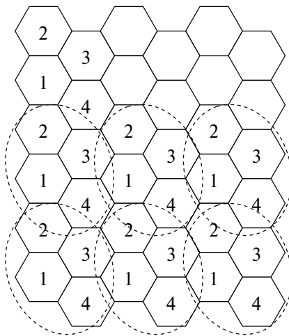
Рис. 1.16. Сотовый принцип, иллюстрирующий схему повторяющихся ячеек, возникающую из-за многократного использования частоты
