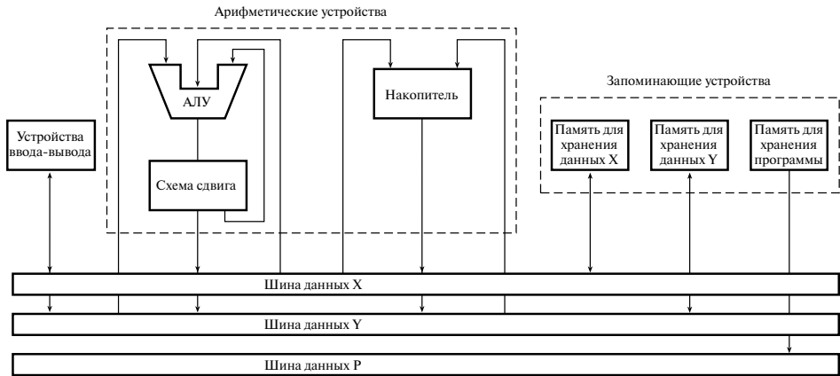
Рис. 12.2. Стандартная универсальная аппаратная архитектура обработки сигналов
