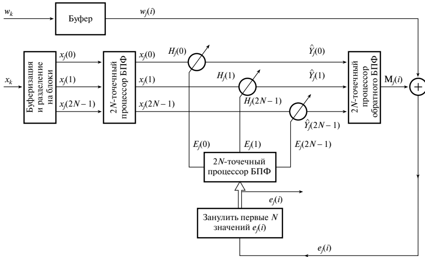
Рис. 10.14. Упрощенная блок-схема фильтра, построенного на основе схемы наименьших квадратов
