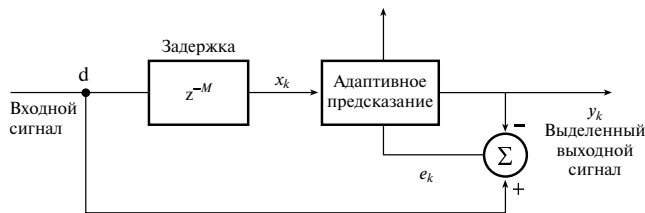
Рис. 10А.1. Адаптивное выделение сигнала
