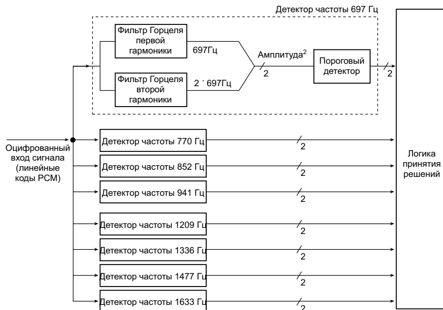
Рис. 8.39. Принципы декодирования ДТМЧ с использованием фильтров Горцеля (согласно [17])
