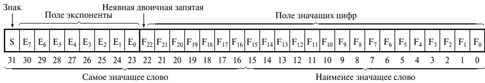
Рис. 13.1. Представление с плавающей запятой (формат IEEE обычной точности)
