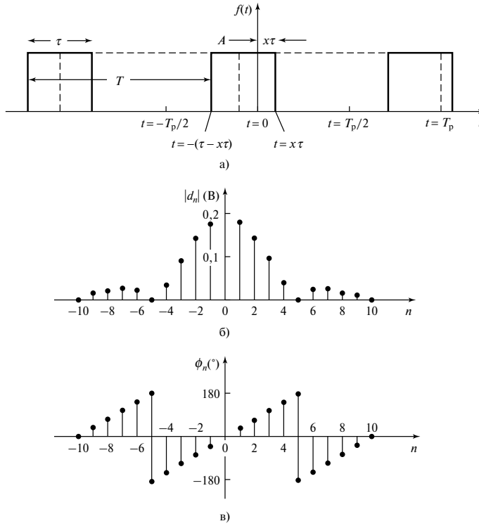
Рис. 3.1. Сигнал f(t) (панель а); амплитудный спектр |d_n| (панель б); фазовый спектр \phi_n (панель в)
