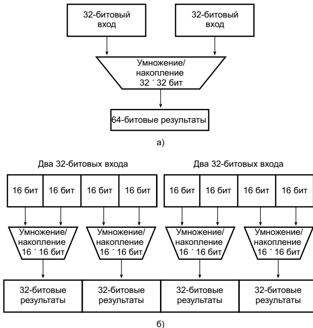
Рис. 12.12. Иллюстрация использования обработки по схеме SIMD и поддержки данных нескольких размеров для увеличения в процессоре TigerSHARC числа умножителей-накопителей с одного до четырех
