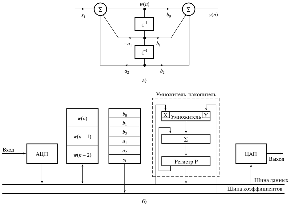
Рис. 12.39. БИХ-фильтр: а) структура; б) гарвардская архитектура биквадратного звена
