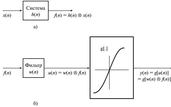
Рис. 5.23. Слепое обращение свертки
