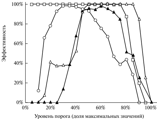
Рис. 14.10. Эффективность метода согласованной фильтрации для данных класса 1 и 2 и шаблонов длины 11 и 31: □ — класс 1, длина 11; △ — класс 1, длина 31; ○ — класс 2, длина 11; ▲ — класс 2, длина 31
