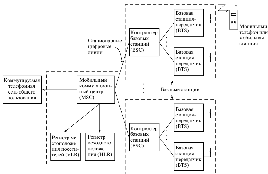
Рис. 1.17. Упрощенная блок-схема мобильной сотовой телефонной системы
