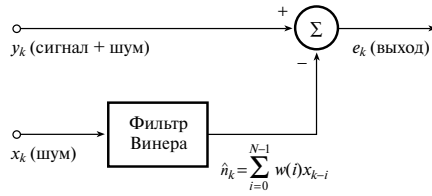
Рис. 10.5. Фильтр Винера (стандартная форма)
