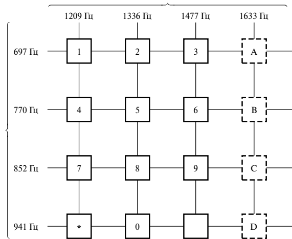
Рис. 8.37. Упрощенная схема клавишного поля 4 \times 4 кнопочного телефона. Кнопки, изображенные пунктиром, недоступны. При нажатии кнопки генерируется пара тонов — один из низкочастотной группы, другой из высокочастотной. Например, при нажатии кнопки 9 генерируются тоны 825 и 1477 Гц (согласно [17])
