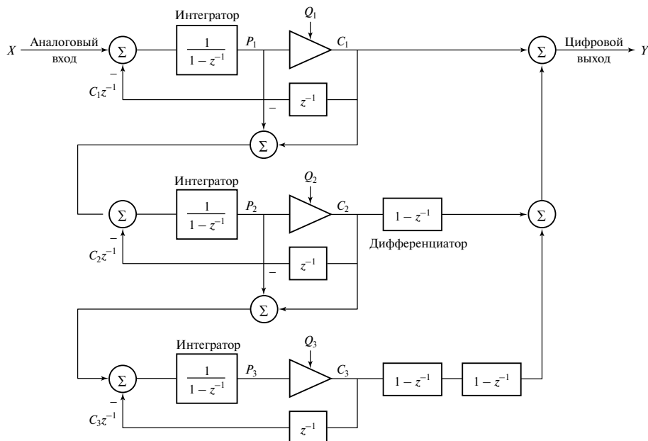
Рис. 2.36. Упрощенный однобитовый АЦП
