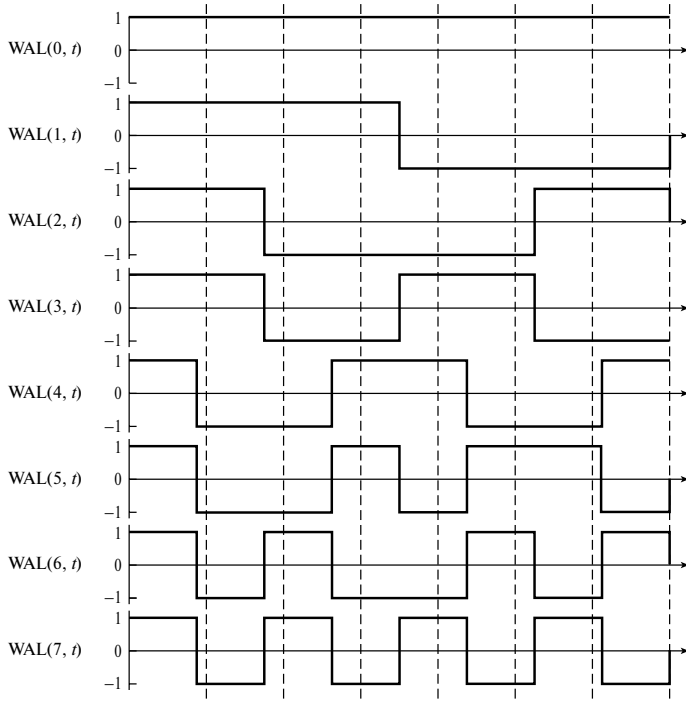
Рис. 3.6. Упорядоченные по возрастанию функции Уолша до n = 7 , которые показывают времена дискретизации для матрицы преобразования Уолша порядка 8 \times 8
