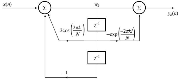
Рис. 8.40. Структура фильтра Горцеля второго порядка
