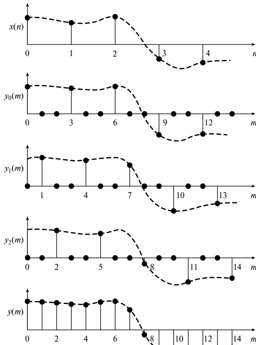
Рис. 9.22. Реализация интерполяции 1:3 на базе многофазных фильтров
