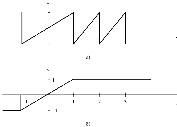
Рис. 13.14. Переполнение: a — характеристика переполнения; б — арифметика насыщения
