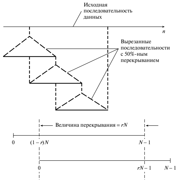
Рис. 11.4. Разбиение данных перед обработкой с избыточностью
