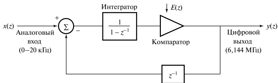
Рис. 2.55. Модель сигма-дельта-модулятора на z -плоскости
