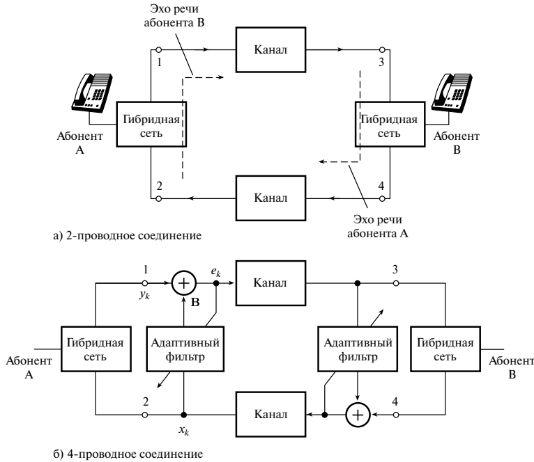
Рис. 10.18. Упрощенная схема междугородного телефонного канала (панель а); эхоподавление в голосовой междугородной телефонной связи (панель б)
