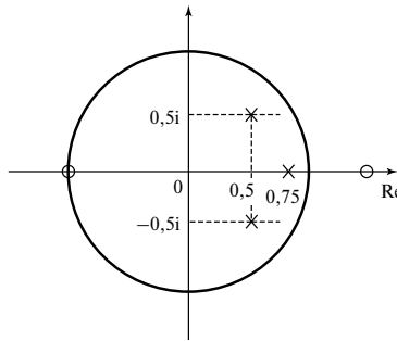
Рис. 4.8. Диаграмма нулей и полюсов для примера 4.10
