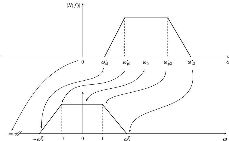
Рис. 8.15. Отображение ФНЧ-прототипа в полосовой фильтр
