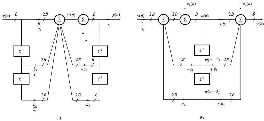
Рис. 13.20. Модели шума для звеньев БИХ-фильтров в современной системе ЦОС. Показаны длины слов в различных точках фильтра. Предполагается, что входные данные и коэффициенты имеют размер по B бит
