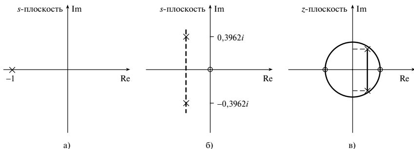
Рис. 8.11. Диаграмма нулей и полюсов для а) фильтра-прототипа нижних частот, б) промежуточного аналогового полосового фильтра и в) дискретного полосового фильтра, полученного путем преобразования полосы
