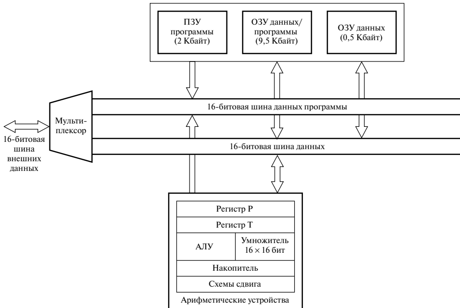
Рис. 12.16. Упрощенная архитектура процессора ЦОС с фиксированной запятой второго поколения (Texas Instruments TMS320C50)
