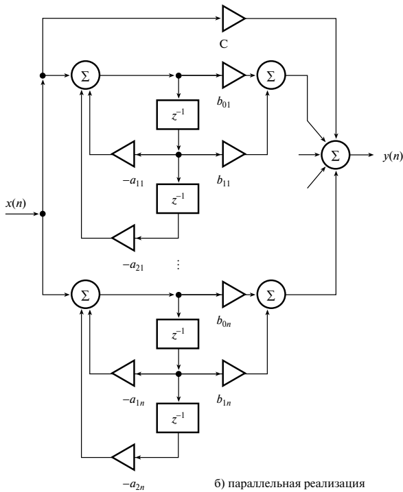
б) параллельная реализация
