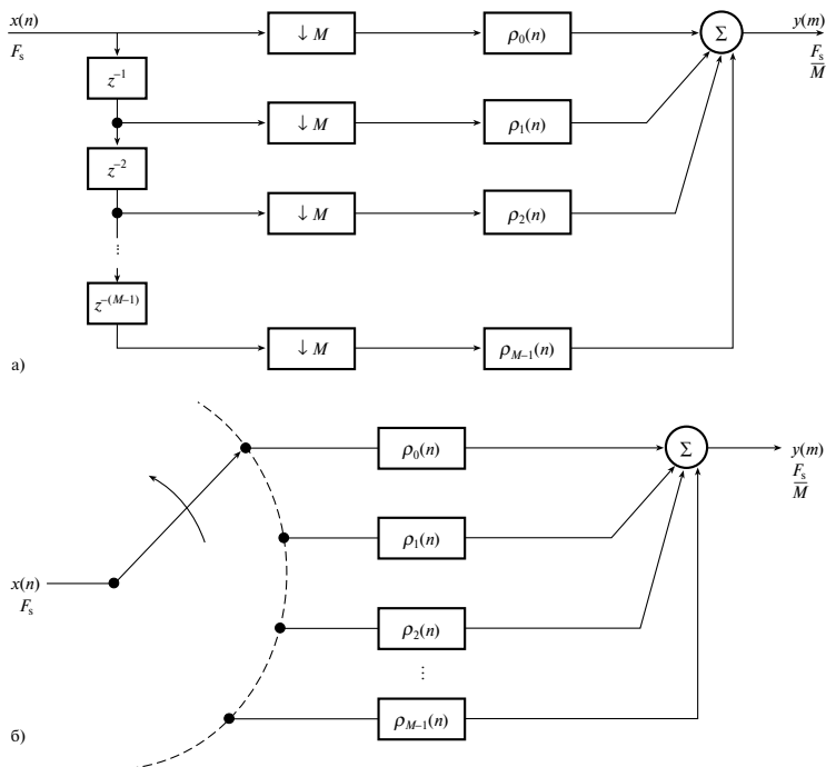
Рис. 9.24. Общая модель децимации на базе многофазных фильтров (панель а). Коммутативная модель реализации (панель б)
