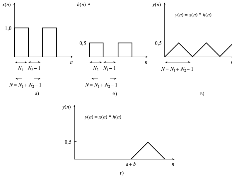
Рис. 5.26. Свертка двух сигналов, изображенных на рис. 5.25, для получения которой x(n) и h(n) транслировались в начало координат. Прибавление к x(n) N_2 - 1 дополняющих нулей (панель а). Прибавление к h(n) N_1 - 1 дополняющих нулей (панель б). Свертка y(n) = x(n) \otimes h(n) (панель в). Правильная линейная свертка получается заменой y(n) вдоль оси n функцией, начинающейся в точке n = a + b (панель з)
