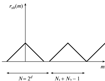
Рис. 5.28. Неверная взаимная корреляция, полученная при трансляции x(n) и h(n) в начало координат
