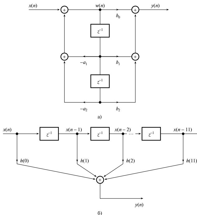
Рис. 6.3. Блок-схема БИХ-фильтра из примера 6.1 (панель а); блок-схема КИХ-фильтра из примера 6.1 (панель б)
