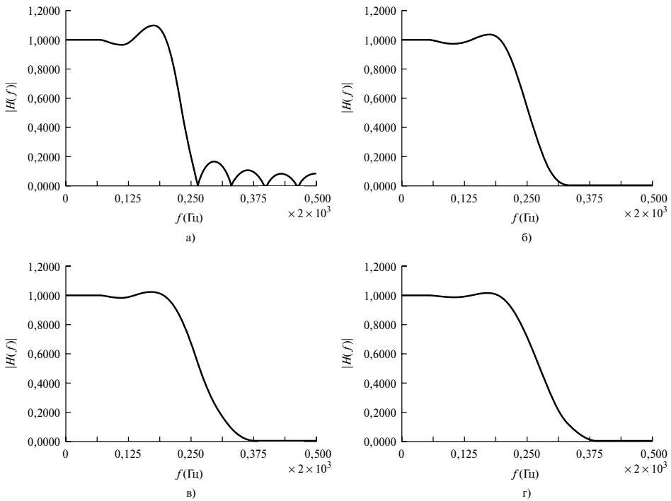
Рис. 7.20. Частотная характеристика фильтра частотной выборки при следующих условиях: а) в полосе перехода нет частотных выборок; б) одна выборка в полосе перехода; в) две выборки в полосе перехода; г) три выборки в полосе перехода
