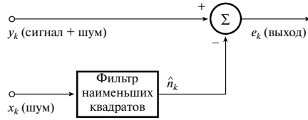
Рис. 10.15. Иллюстрация основной идеи метода наименьших квадратов
