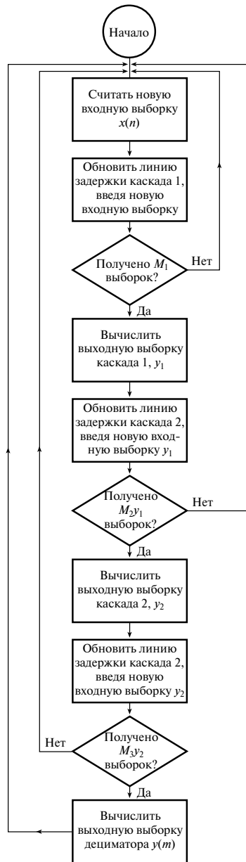
Рис. 9.15. Функциональная схема трехкаскадного дециматора
