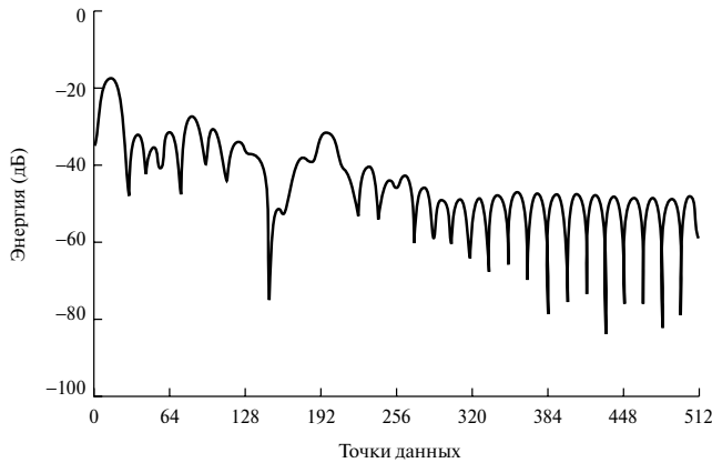
Рис. 11.7. Энергетический спектр при выборке с интервалом 1 с, весовая функция Кайзера-Бесселя, 64 информационные точки, 1024-точечное БПФ. Средний уровень взвешенных данных удален путем вычитания среднего из данных
