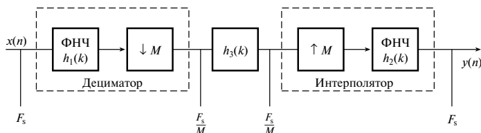
Рис. 9.32. Узкополосная фильтрация с обработкой при нескольких скоростях
