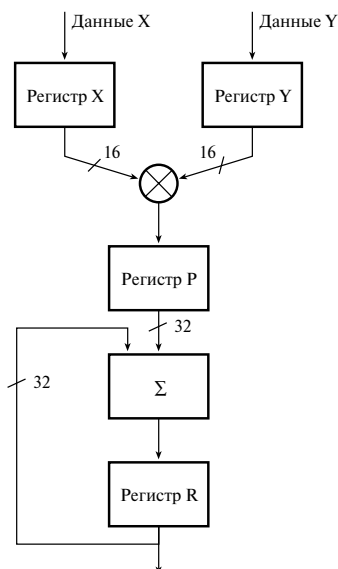
Рис. 12.10. Типичная для ЦОС конфигурация умножителя-накопителя
