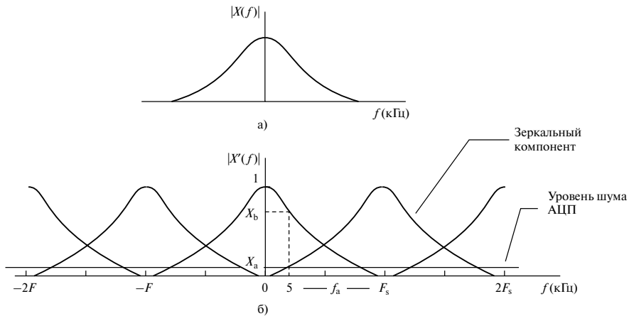
Рис. 2.9. Спектр дискретного сигнала, на котором показано искажение, вызванное наложением и шумом квантования АЦП
