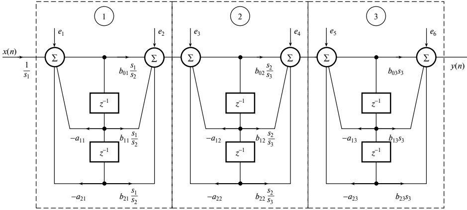
Рис. 13.18. Шумовая модель каскадной реализации БИХ-фильтра шестого порядка
