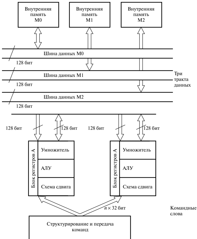
Рис. 12.14. Принципы суперскалярной архитектуры и схема потока данных в процессоре ЦОС TigerSHARC
