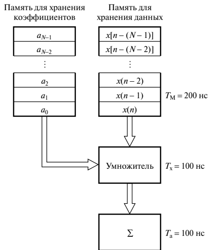
Рис. 12.7. Конфигурация умножителя-накопителя без конвейерной обработки. Произведения подаются в накопитель каждые 400 нс
