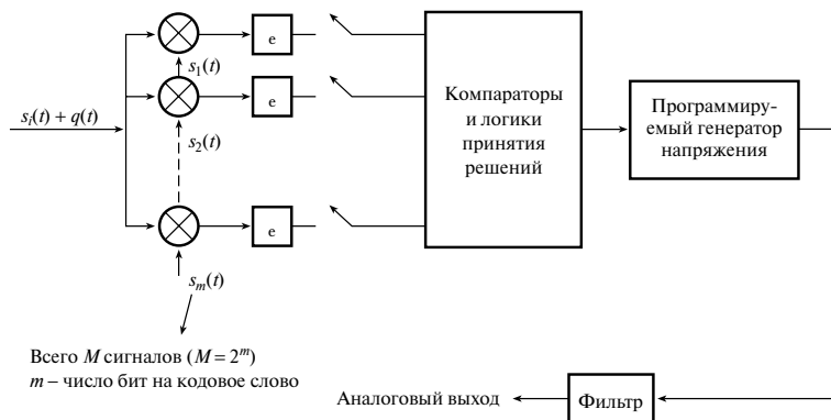
Рис. 5.14. Детектор кодовых слов PCM, основанный на корреляционном детекторе
