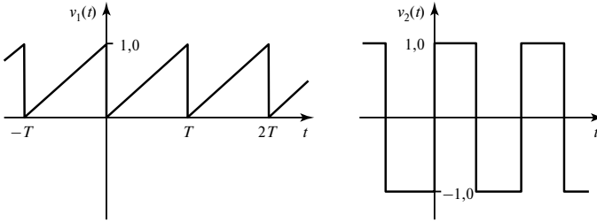
Рис. 5.6. Сигналы v_1(t) и v_2(t) (пример 5.3)
