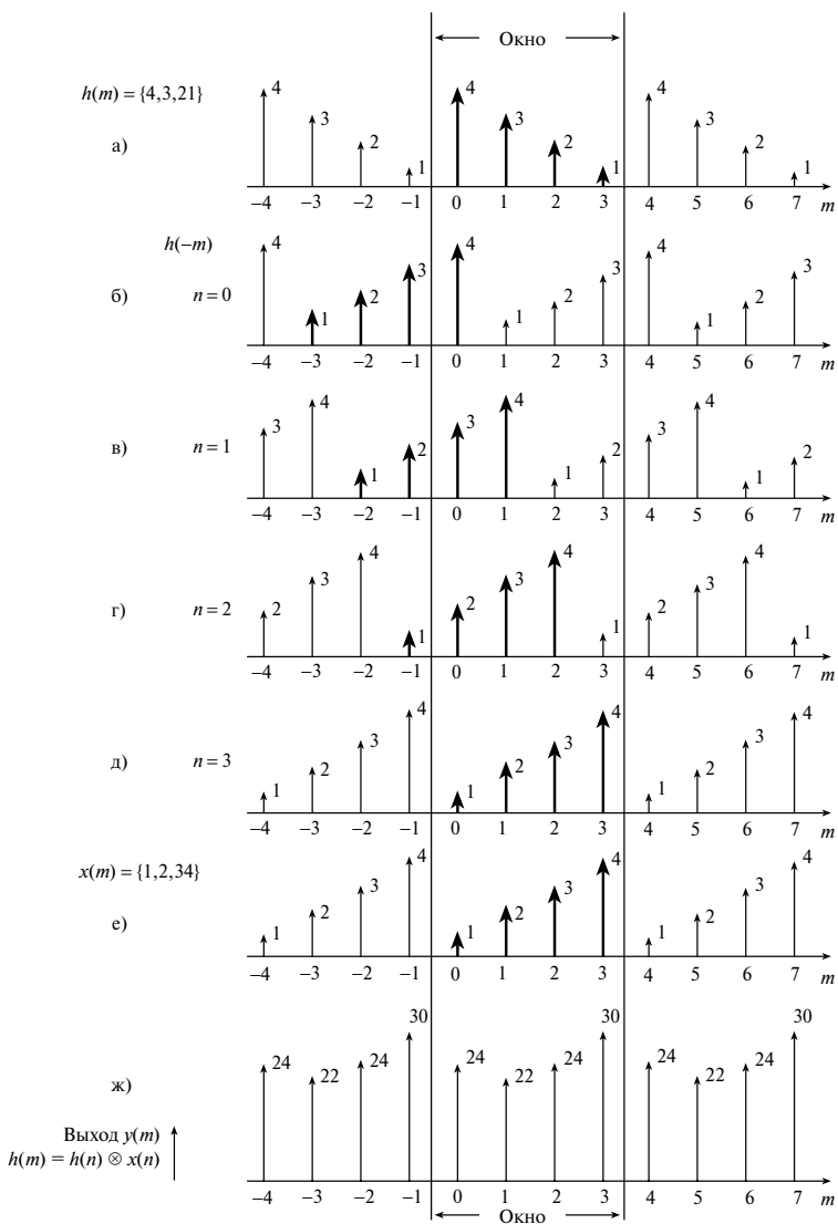
Рис. 5.20. Свертка y(m) последовательностей h(n) и x(n) : а) периодическая последовательность h(m) ; б) обращенная во времени последовательность h(-m) ; в)–д) копии h(-m) , последовательно смещаемые вправо; е) последовательность x(m) ; ж) выходная последовательность y(m) = h(n) \otimes x(n)
