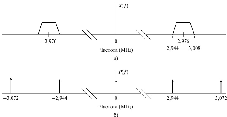
Рис. 2.52. Спектр сигнала на втором промежуточном этапе (панель а); спектр выборочной функции (панель б)
