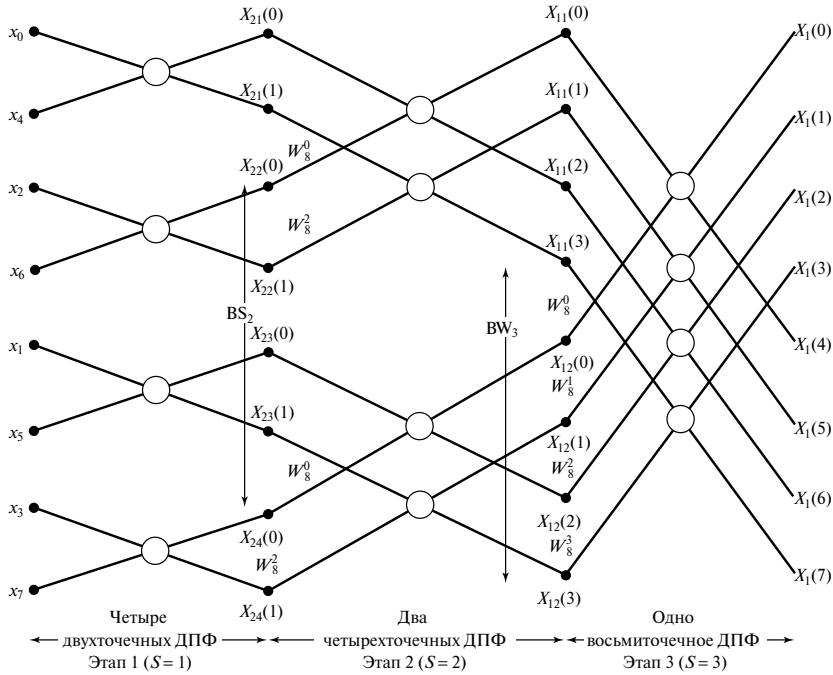
Рис. 3.5. “Бабочки” восьмиточечного ДПФ: BW_3 — память, выделенная точкам, дающим вклад в самую большую “бабочку” этапа 3; BS_2 — память, выделенная верхним точкам “бабочки” этапа 2 с одинаковыми весовыми коэффициентами
