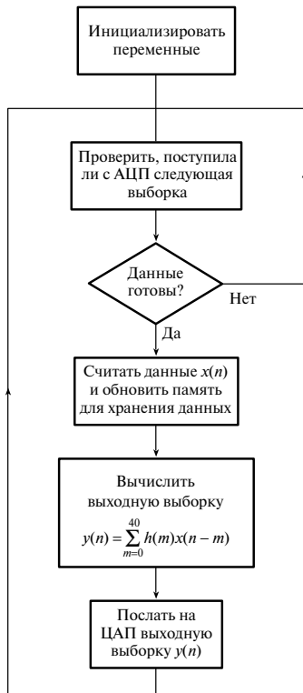
Рис. 7.35. Упрощенная функциональная схема трансверсального КИХ-фильтра реального времени
