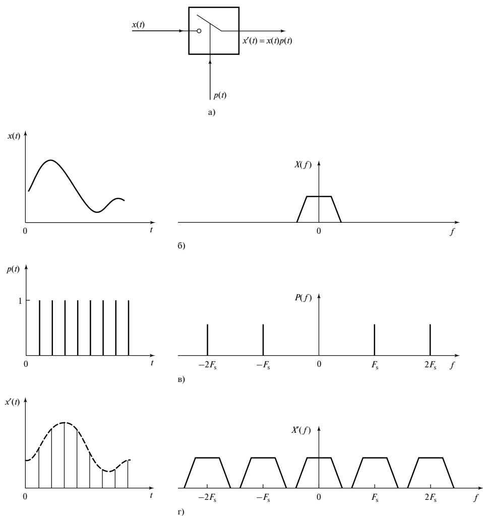
Рис. 2.5. Описание процесса дискретизации во временной и частотной областях. Сравните спектры сигнала до (б) и после (г) дискретизации. Обратите внимание на изменения в дискретном сигнале и, в частности, на то, что спектр дискретного сигнала повторяется в точках, кратных частоте дискретизации F_s
