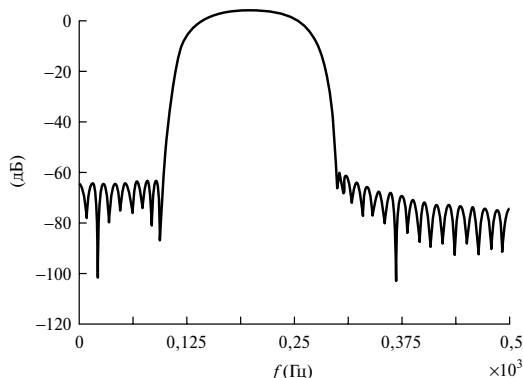
Рис. 7.8. Спектр фильтра (пример 7.4)
