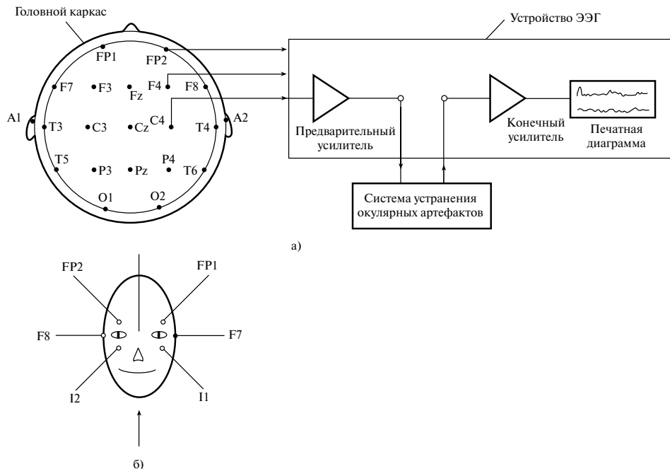
Рис. 14.15. Используемая экспериментальная установка: а) соединение с аппаратом ЭЭГ; б) размещение электродов для снятия ЭОГ
