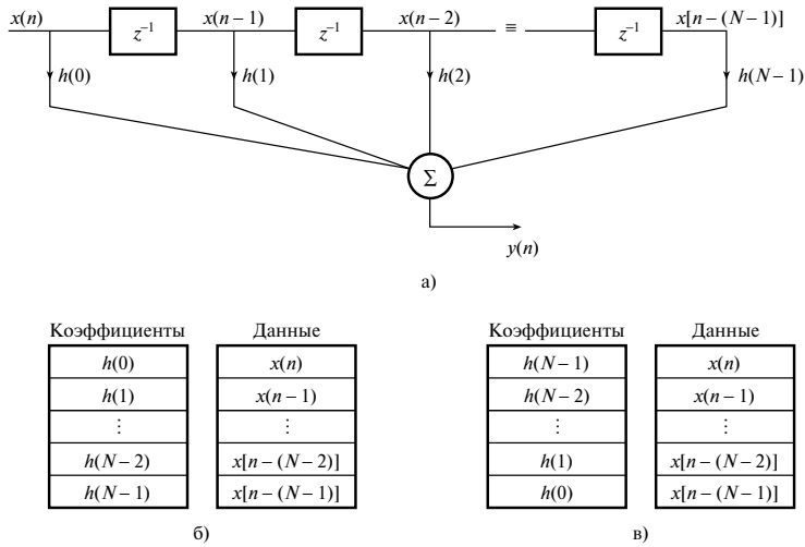
Рис. 12.24. Реализация КИХ-фильтра: а) структура фильтра; б) карты памяти коэффициентов и данных; в) альтернативная карта памяти
