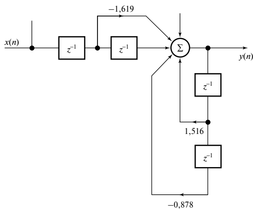
Рис. 4.17. Блок-схема системы дискретного времени из задачи 4.11
