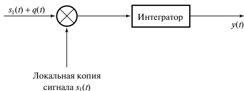
Рис. 5.13. Схематическое изображение корреляционного детектора
