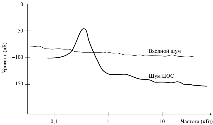
Рис. 13.2. Иллюстрация влияния шума округления в обработке сигналов на уровень собственных шумов системы
