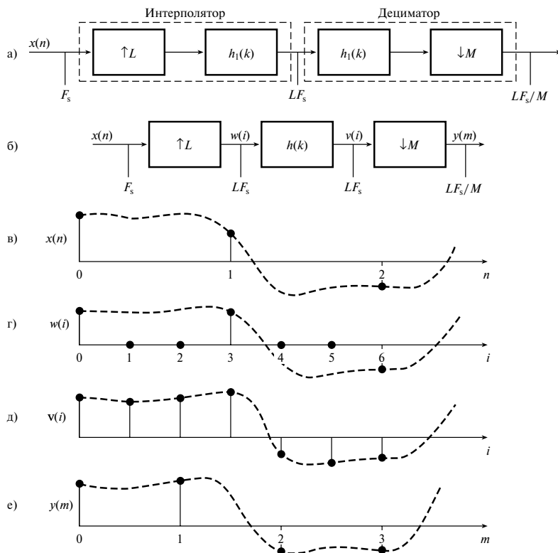
Рис. 9.5. Иллюстрация интерполяции с рациональным шагом ( L = 3 , M = 2 )
