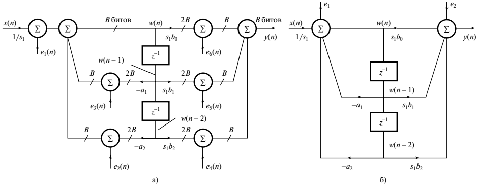
Рис. 13.17. Модель шума квантования произведения для канонического фильтрующего звена. Все источники шума, выход которых на панели a поступает в одну точку, на панели б объединены
