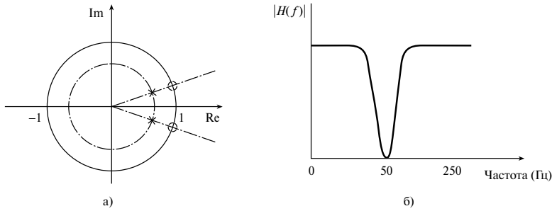
Рис. 8.5. Диаграмма нулей и полюсов фильтра из примера 8.2 (панель а); соответствующая частотная характеристика (панель б)
