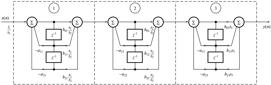
Рис. 13.12. Масштабирование в каскадной реализации БИХ-фильтра шестого порядка (масштабные коэффициенты внесены в числитель, т.е. представлены коэффициенты прямой связи)
