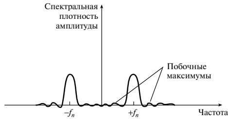
Рис. 11.2. Спектральная плотность амплитуды синусоидального сигнала, свернутого с дискретизирующей функцией
