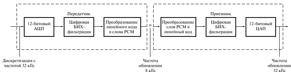
Рис. 8.36. Канал РСМ, демонстрирующий возможное использование БИХ-фильтров как фильтров защиты от наложения спектров (передатчик) и фильтров подавления зеркальных частот (приемник)
