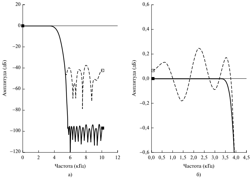
Рис. 7.31. Влияние квантования коэффициентов (пример 7.18) (панель а). Полоса пропускания (■ — неквантованная характеристика, □ — квантованная) (панель б)
