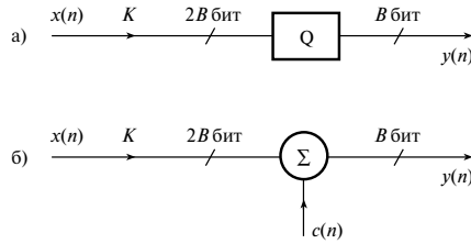
Рис. 13.15. Представление ошибки квантования произведения: а — блок-схема процесса квантования; б — линейная модель процесса квантования
