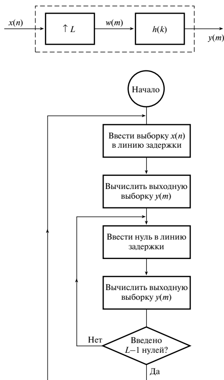
Рис. 9.18. Функциональная схема процесса интерполяции
