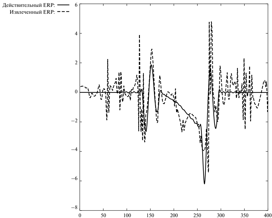
Рис. 3.15. Потенциал ERP, очищенный методом определения сингулярностей, и реальный потенциал ERP (белый шум, отношение сигнал-шум -5, 67 дБ)
