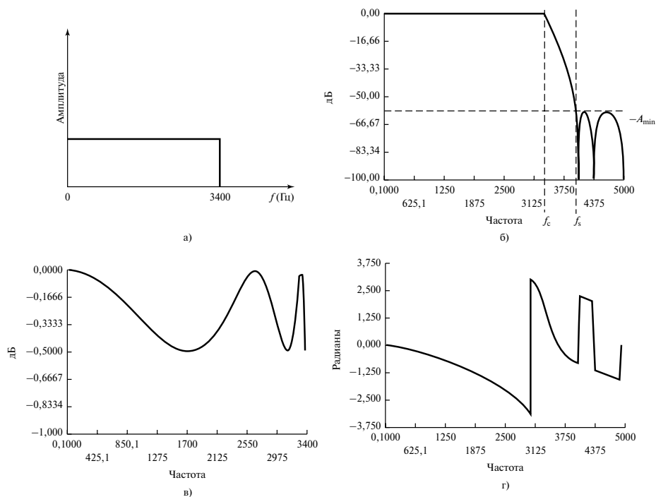
Рис. 2.7. Идеальная и реальные частотные характеристики фильтров защиты от наложения спектров, показывающие ошибки, которые дают реальные фильтры: а) идеальная характеристика; б) реальная амплитудная характеристика; в) реальная полосовая амплитудная характеристика; г) реальная фазовая характеристика. Сравним, к примеру, плоскую полосовую характеристику на панели а и реальную полосовую характеристику на панели в: неравномерность реальной характеристики приводит к амплитудному искажению внутриполосных компонентов сигнала
