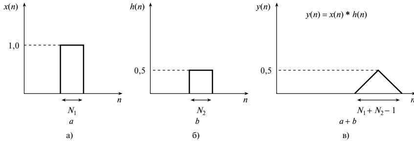
Рис. 5.25. Свертка y(n) = x(n) \otimes h(n) двух сигналов x(n) и h(n) , не выходящих из начала координат
