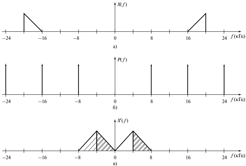
Рис. 2.23. Спектр дискретного сигнала для нечетных целых n ( n = f_H/B = 5 ) (пример 2.7, вариант 2)
