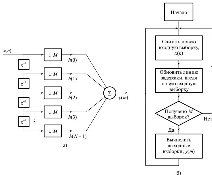
Рис. 9.14. Более эффективная диаграмма прохождения сигнала через дециматор (панель а); функциональная схема процесса децимации (панель б)
