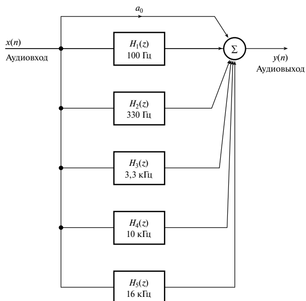
Рис. 8.33. Упрощенная диаграмма полностью цифрового графического эквалайзера. Основной компонент — блок параллельных БИХ-фильтров с различными центральными частотами. Усиление каждого фильтра можно регулировать независимо, например, с помощью скользящего потенциометра, скажем, в диапазоне \pm 10 дБ
