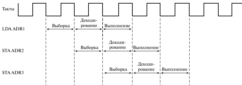
Рис. 12.5. Иллюстрация совмещения команд, возможного при использовании гарвардской архитектуры
