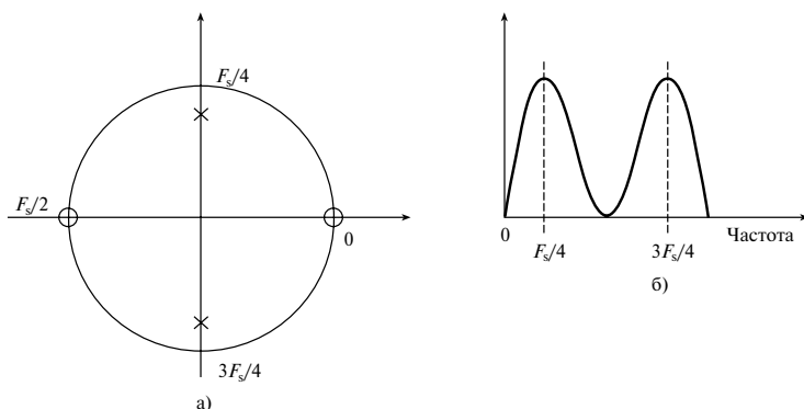
Рис. 8.3. Диаграмма нулей и полюсов простого фильтра (панель а); схематическое изображение частотной характеристики этого фильтра (панель б)
