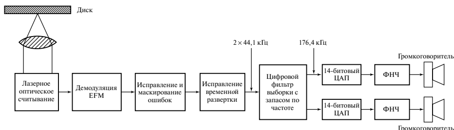
Рис. 1.14. Воспроизведение звукового сигнала с компакт-диска
