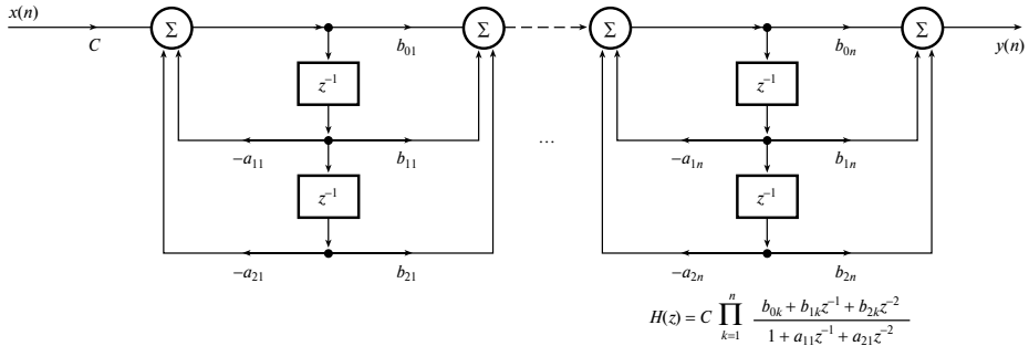
Рис. 8.27. Каскадная реализация
