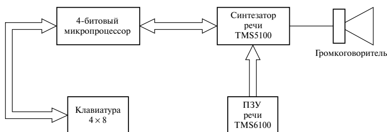
Рис. 1.10. Структура пособия Speak and Spell
