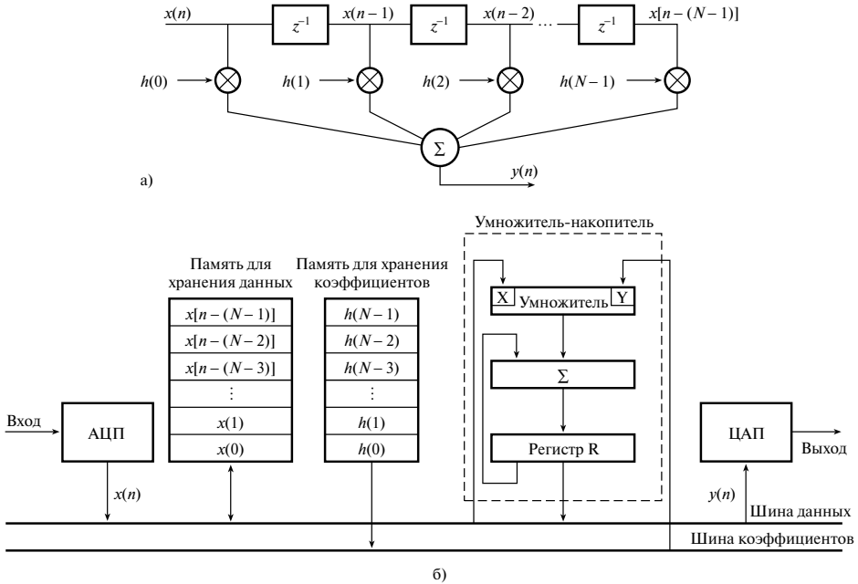
Рис. 12.38. Архитектура аппаратного цифрового КИХ-фильтра
