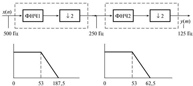
Рис. 9.35. Дециматор для уменьшения частоты ЭКГ-данных
