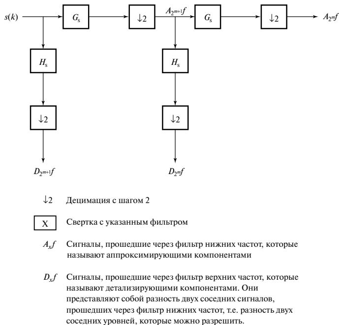
Рис. 3.10. Разложение сигнала для КА вейвлетным методом
