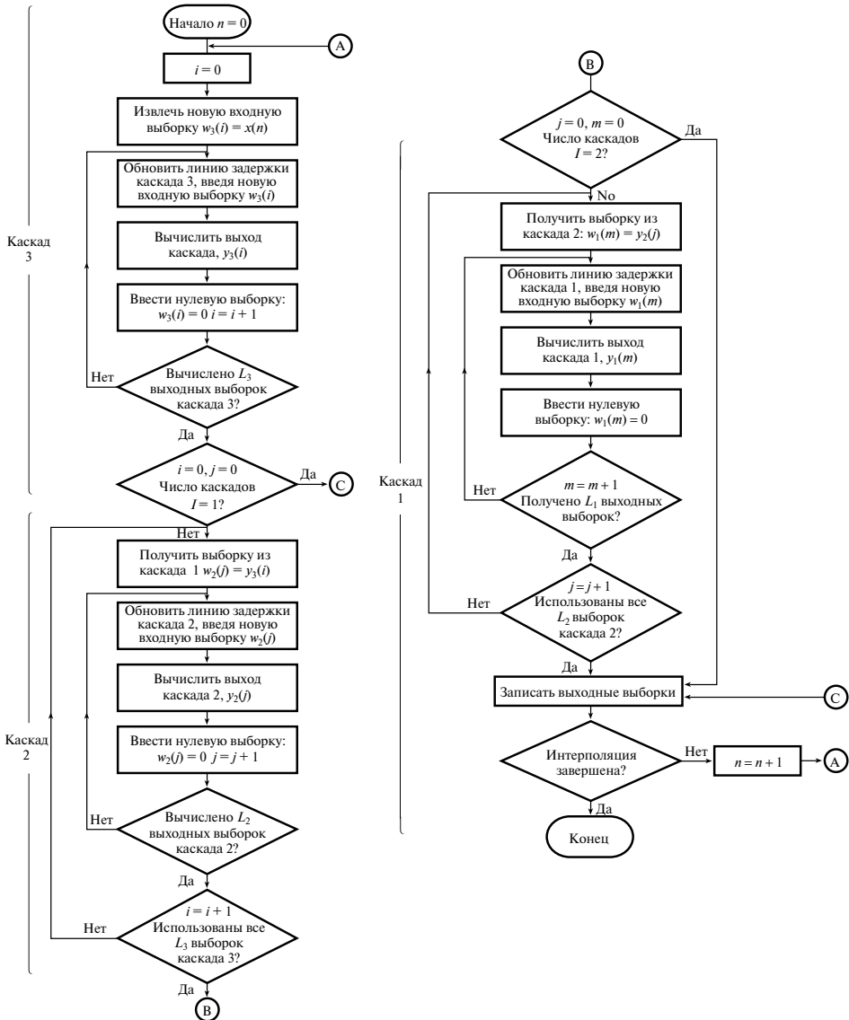
Рис. 9.19. Интерполяция с использованием до трех каскадов. Если, например, I = 1 , то выполняются только блоки с меткой “каскад 3”
