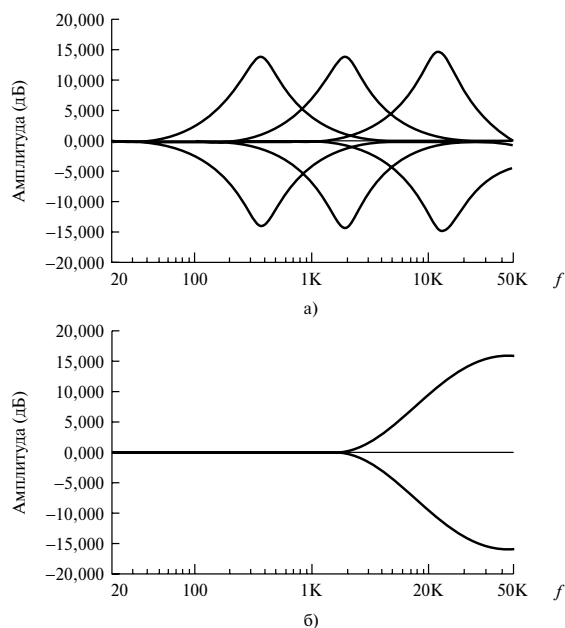
Рис. 14.18. Амплитудная характеристика звонкового фильтра для различных центральных частот и шириин полос (панель а ). Амплитудная характеристика полочного фильтра (панель б )
