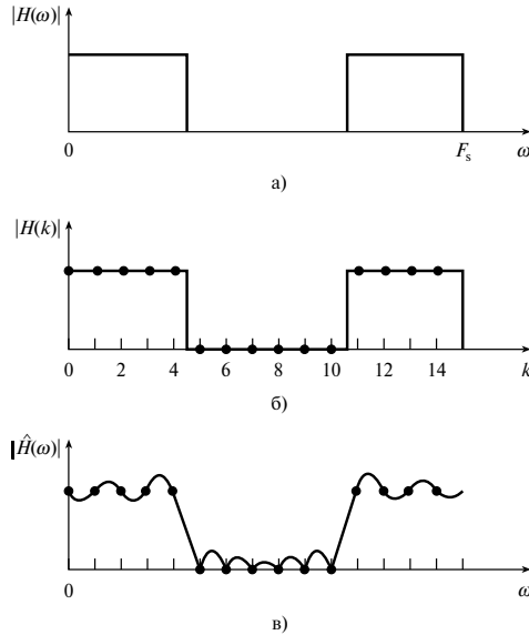
Рис. 7.16. Понятие частотной выборки: а) частотная характеристика идеального фильтра нижних частот; б) выборки идеального фильтра нижних частот; в) частотная характеристика фильтра нижних частот, выведенная из частотных выборок панели б
