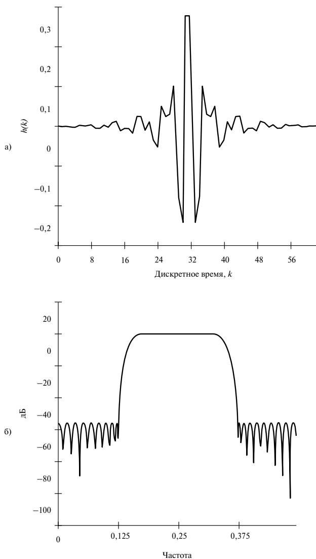
Рис. 1.5. Описание цифрового фильтра во временных и частотных координатах: а) импульсная характеристика; б) спектр фильтра. Спектр фильтра был получен с помощью дискретного преобразования h(n) , что иллюстрирует одно из возможных применений ДПФ
