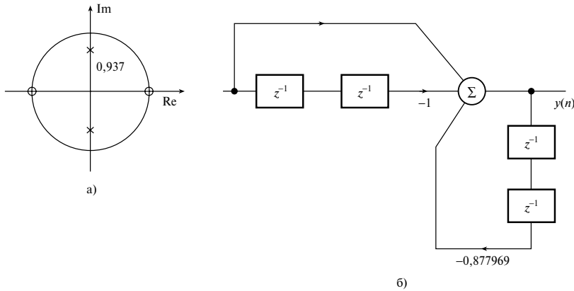
Рис. 8.4. Диаграмма нулей и полюсов (панель а). Блок-схема фильтра (панель б)
