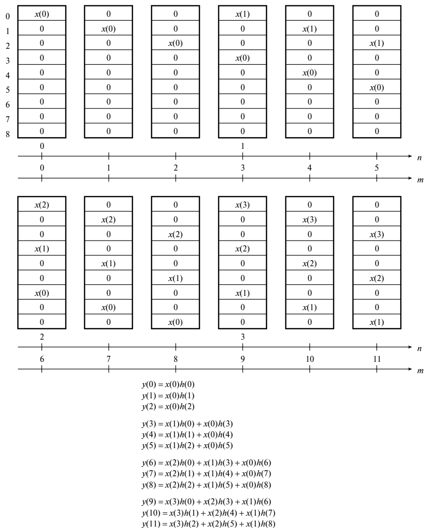
Рис. 9.21. Интерполяция 1:3 с использованием многофазных фильтров: а) содержимое линии задержки в два различных момента взятия выборки n и m ; б) выходные выборки многофазных фильтров
