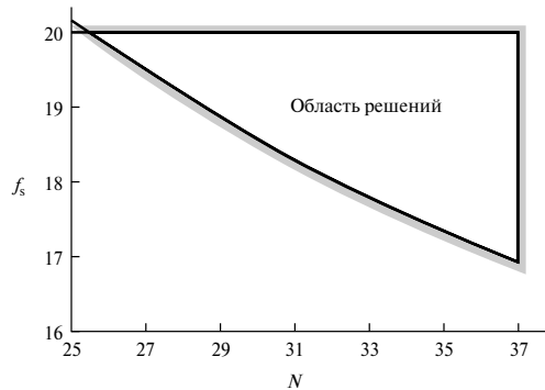
Рис. 7.15. Зависимость положения края полосы подавления от длины фильтра с указанным диапазоном возможных решений
