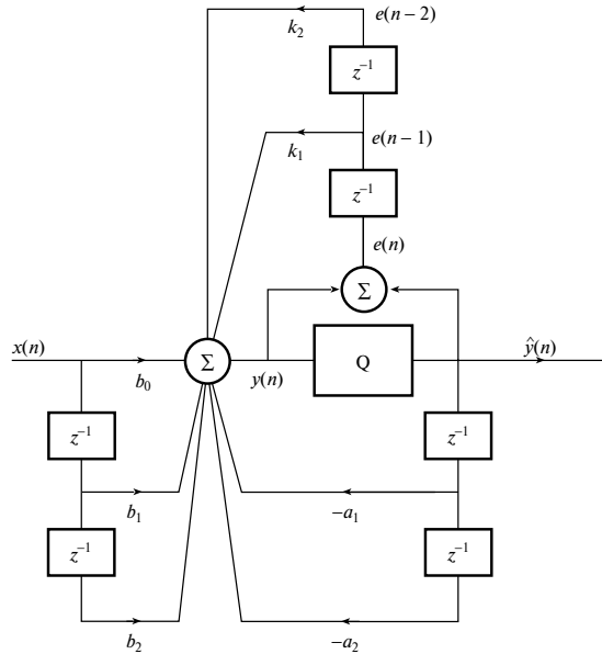
Рис. 14.20. Схема снижения шума второго порядка
