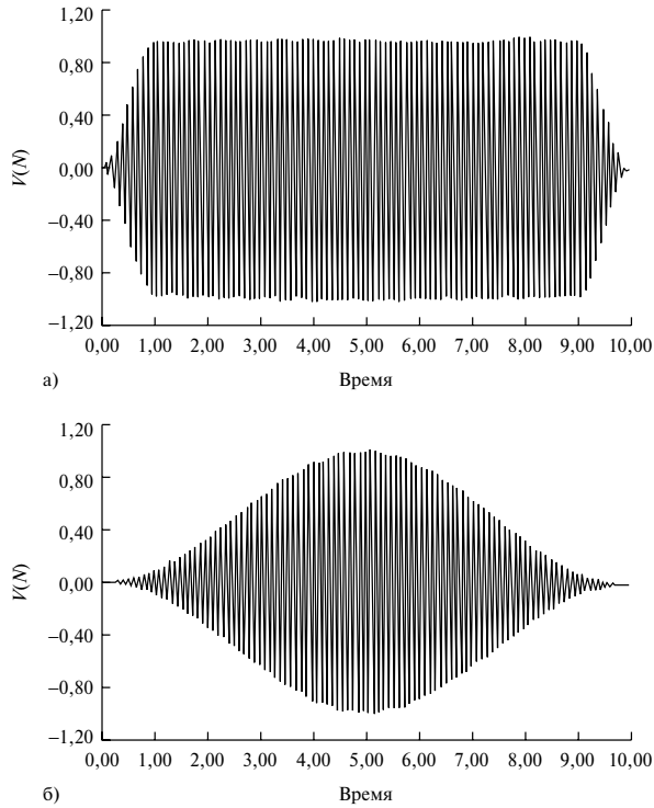
Рис. 11.10. Весовая функция Тьюки: а) \alpha = 0, 1 ; б) \alpha = 0, 5
