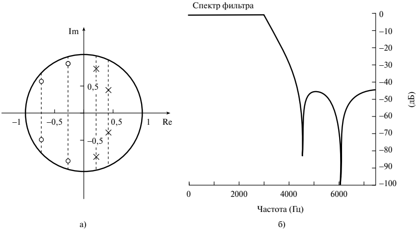
Рис. 8.32. Диаграмма нулей и полюсов (панель а) и частотная характеристика фильтра из раздела 8.16 (панель б)
