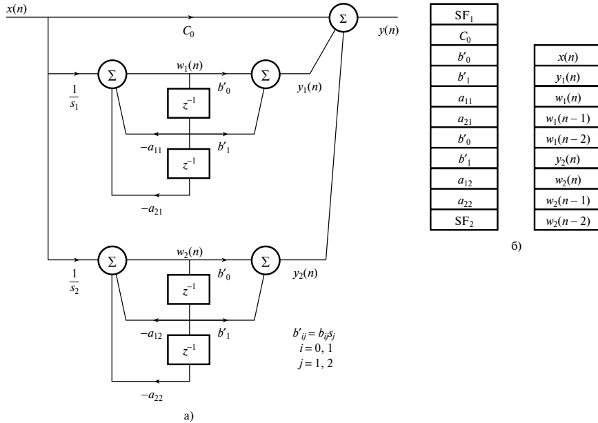
Рис. 12.30. Реализация БИХ-фильтра четвертого порядка: а) диаграмма реализации; б) схема памяти для хранения данных и коэффициентов
