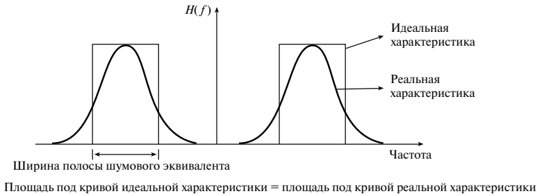
Рис. 11.3. Ширина полосы шумового эквивалента
