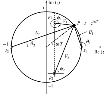
Рис. 4.9. Геометрическая оценка частотной характеристики по диаграмме нулей и полюсов
