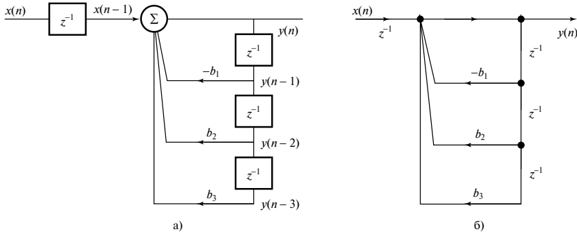
Рис. 4.14. Диаграммы реализации разностного уравнения: a — в виде блок-схемы; b — в виде функциональной схемы
