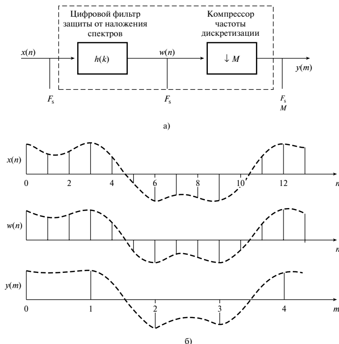
Рис. 9.1. Блок-схема децимации с шагом M (панель а ). Иллюстрация децимации с шагом M = 3 (панель б ). Обратите внимание на то, что на выход поступает только одна из каждых трех выборок w(n)
