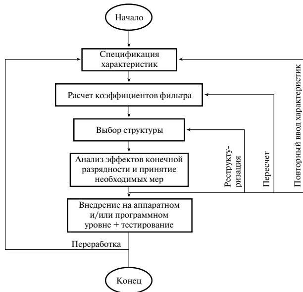
Рис. 7.2. Этапы разработки цифровых фильтров
