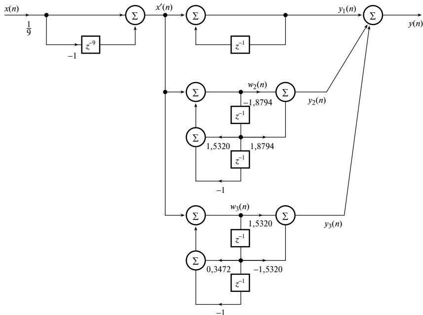
Рис. 7.23. Диаграмма реализации для фильтра частотной выборки из примера 7.12
