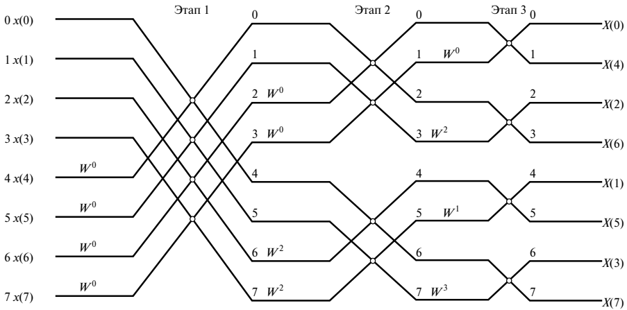
Рис. 12.32. Диаграмма прохождения сигнала по БПФ с децимацией во времени с замещением, где вход идет в естественном порядке, а выход записан в порядке, определяемом обращенными битами
