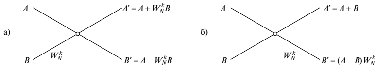
Рис. 12.31. Два типа “бабочек”, используемых в алгоритмах двоичного БПФ: а) “бабочка” для двоичного БПФ с децимацией во времени; б) “бабочка” для двоичного БПФ с децимацией по частоте
