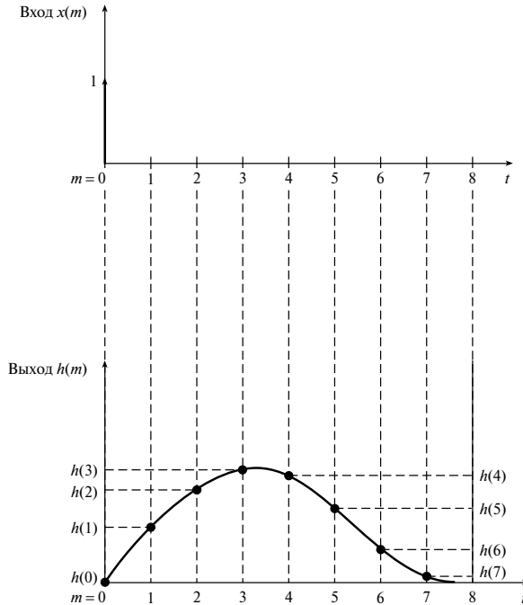
Рис. 5.18. Входной импульс и соответствующая импульсная характеристика системы
