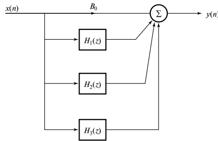
Рис. 4.16. Общая схема параллельной реализации
