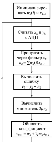
Рис. 10.8. Функциональная схема адаптивной фильтрации по схеме наименьших квадратов
