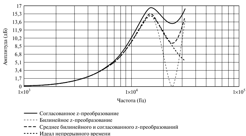
Рис. 8.21. Амплитудная характеристика фильтров, полученных методами согласованного z -преобразования, билинейного z -преобразования, усредненного согласованного/билинейного z -преобразования и аналогового эталона, 15 кГц, Q = 2 , усиление 15 дБ
