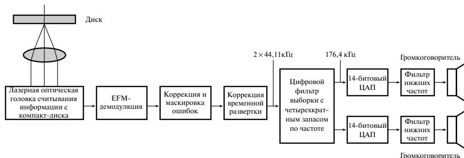
Рис. 9.26. Воспроизведение аудиосигнала в проигрывателе компакт-дисков
