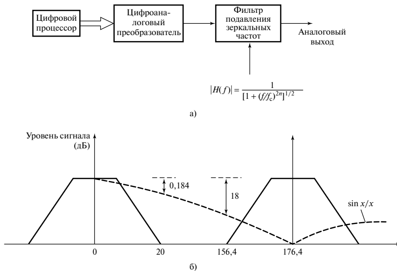
Рис. 2.44. Устройство предварительной обработки данных системы ЦОС реального времени (панель а). Спектр на выходе ЦАП (панель б)
