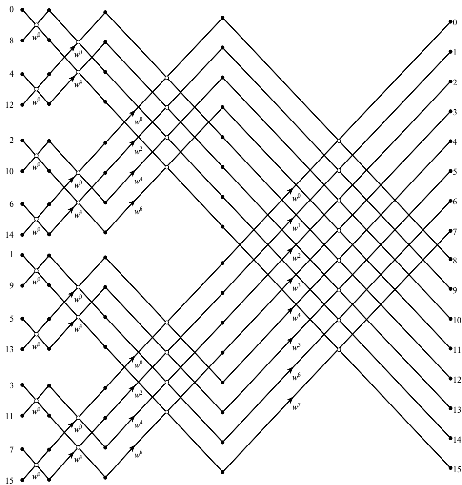
Рис. 12.43. Схема прохождения сигнала 16-точечного двоичного БПФ с децимацией по времени
