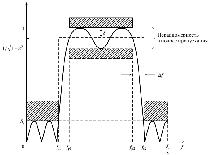
Рис. 8.2. Схема допусков для полосового БИХ-фильтра
