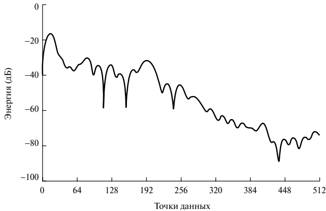
Рис. 11.8. Энергетический спектр при выборке с интервалом 1 с, весовая функция Кайзера–Бесселя, 64 информационные точки, 1024-точечное БПФ. Данные прошли предварительную обработку с целью удаления среднего уровня взвешенных данных и сохранения средней мощности
