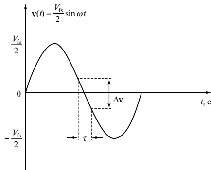
Рис. 2.16. Синусоидальный сигнал (пример 2.5)
