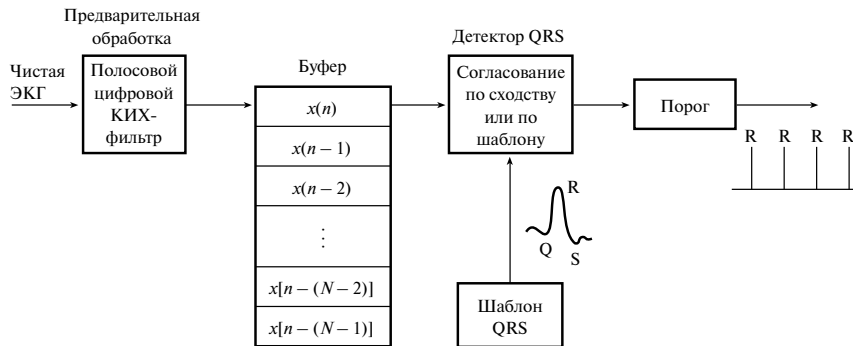
Рис. 14.8. Концепции детектирования комплексов QRS по необработанной ЭКГ
