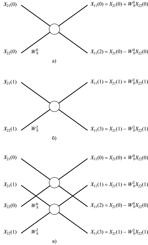
Рис. 3.4. “Бабочки” БПФ
