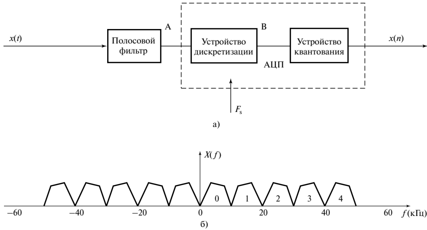
Рис. 2.18. Устройство для предварительной обработки данных системы (панель а); спектр принятого сигнала (панель б) (пример 2.6)
