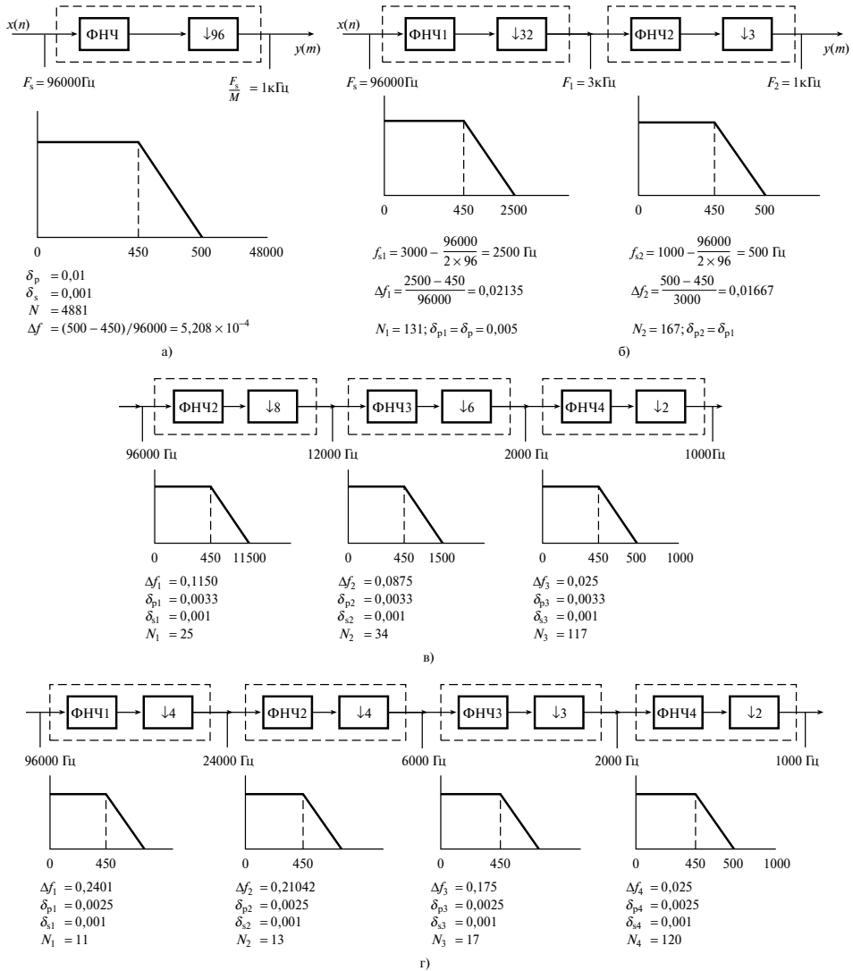
Рис. 9.11. Однокаскадный дециматор (панель а); двухкаскадный дециматор (панель б); трехкаскадный дециматор (панель в); четырехкаскадный дециматор (панель г) (пример 9.3)
