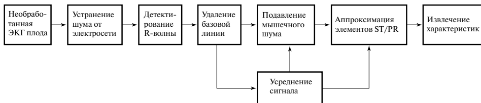
Рис. 1.23. Схема обработки сигнала ЭКГ плода
