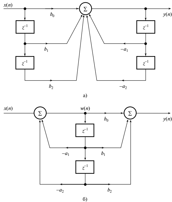
Рис. 13.3. Стандартные блоки БИХ-фильтров: а) звено второго порядка, реализованное в прямой форме I; б) каноническое звено второго порядка
