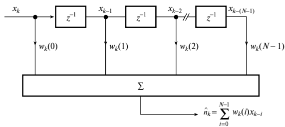
Рис. 10.4. Структура фильтра с конечной импульсной характеристикой
