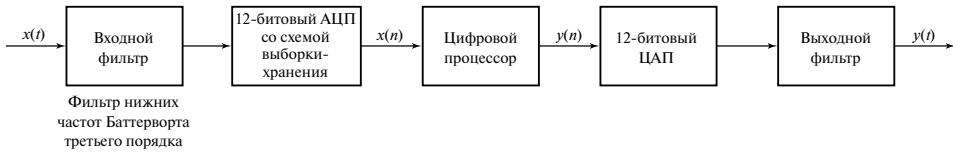
Рис. 2.12. Система цифровой обработки сигналов реального времени
