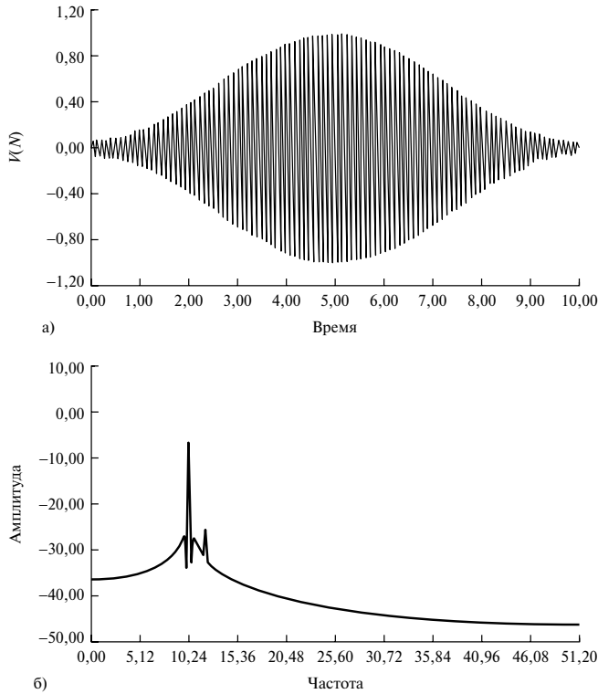
Рис. 11.12. Весовая функция Хэмминга (панель a ); соответствующий амплитудный спектр двух синусоид (панель б )
