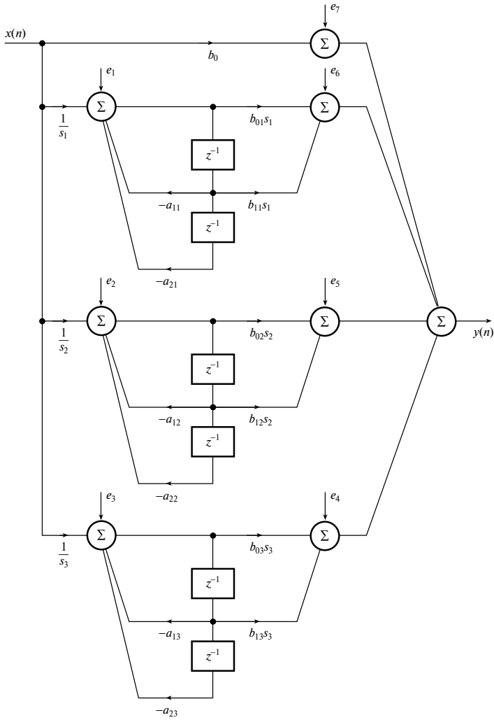
Рис. 13.19. Шумовая модель каскадной реализации БИХ-фильтра шестого порядка
