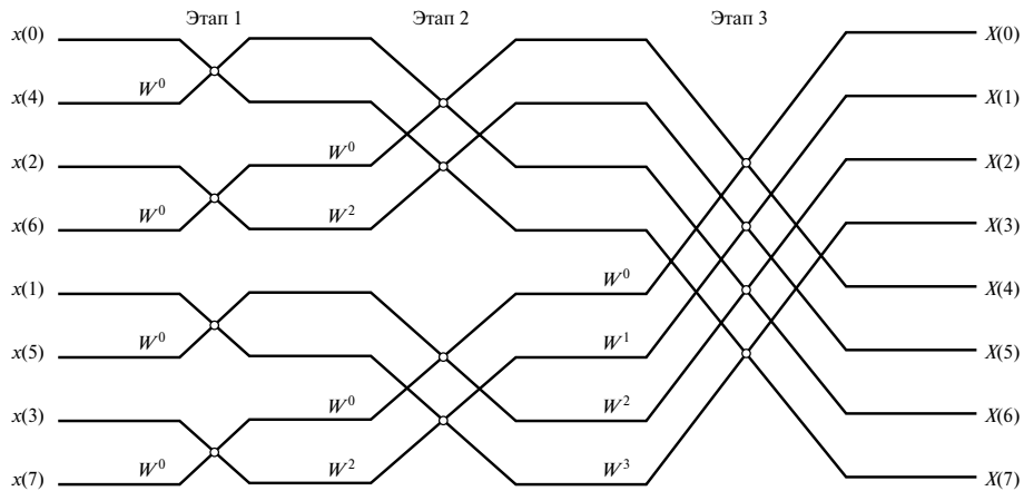
Рис. 12.34. Диаграмма прохождения сигнала для БПФ с децимацией во времени и замещением ячеек памяти; вход представлен в порядке, определяемом обращенными битами, а выход идет в естественном порядке
