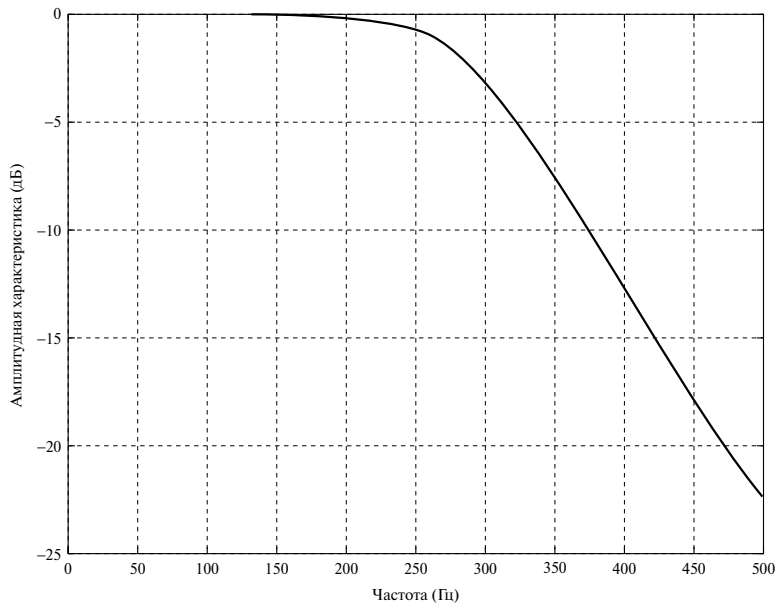
Рис. 8.18. Амплитудная характеристика аналогового фильтра
