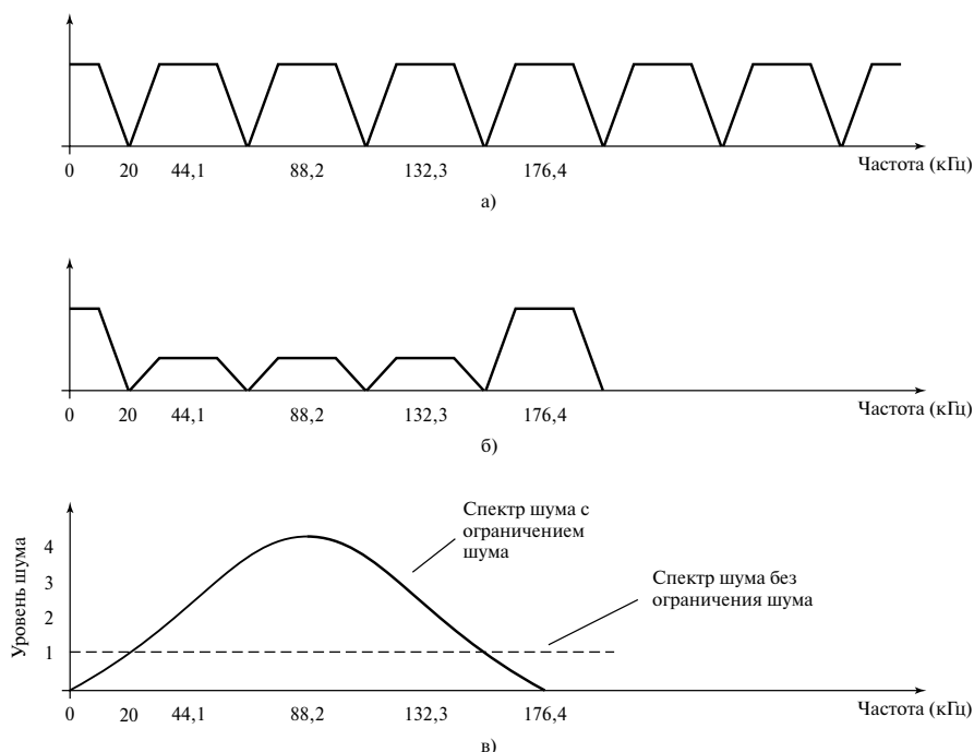
Рис. 2.43. Спектр выборок звукового сигнала с частотой 44,1 кГц (панель а); спектр сигнала с четырехкратной переборкой, на котором показаны значительно уменьшенные зеркальные компоненты (панель б); действие схемы ограничения шума на спектр шума (панель в). Обратите внимание на то, что в полосе звуковых частот (0–20 кГц) уровень шума значительно меньше, чем в области высоких частот, и сравним со спектром шумов, если бы не было ограничения шума (показанного пунктирной линией)
