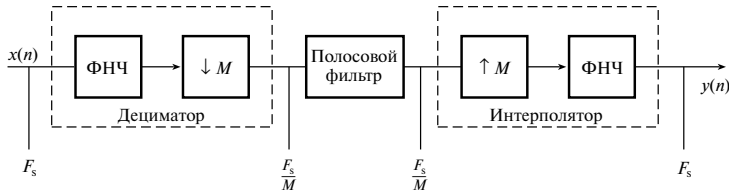
Рис. 9.33. Узкополосная полосовая фильтрация с обработкой при нескольких скоростях
