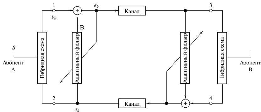
Рис. 1.20. Эхоподавление в междугородной телефонной связи
