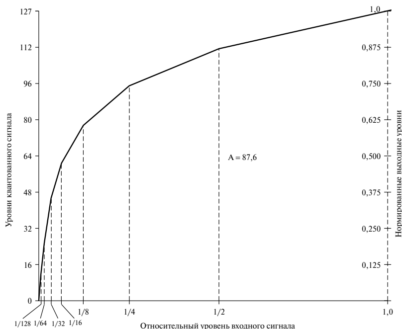
Рис. 2.28. Характеристики компрессирования для А-характеристики ( A = 255 ) [ITU, 1998]. Характеристики подчиняются уравнению F(x) = \text{sgn}(x) \frac{A|x|}{1+\ln(A)} , 0 \leq |x| < 1/A ; F(x) = \text{sgn}(x) \frac{1+\ln(A|x|)}{1+\ln(A)} , 1/A \leq |x| < 1 , где A = 87,6 , x — нормированный входной сигнал, \text{sgn} — его знак, а F(x) — сжатый выходной сигнал
