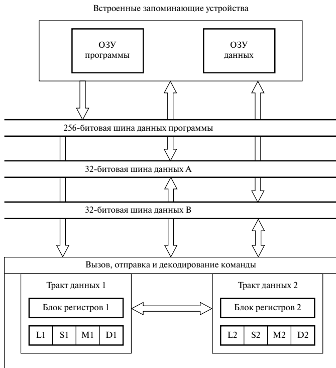
Рис. 12.23. Упрощенная архитектура процессора ЦОС с фиксированной запятой четвертого поколения (Texas Instruments TMS320C62x). Обратите внимание на два независимых арифметических тракта передачи данных, каждый из которых имеет четыре операционных блока — L1, S1, M1 и D1; L2, S2, M2 и D2
