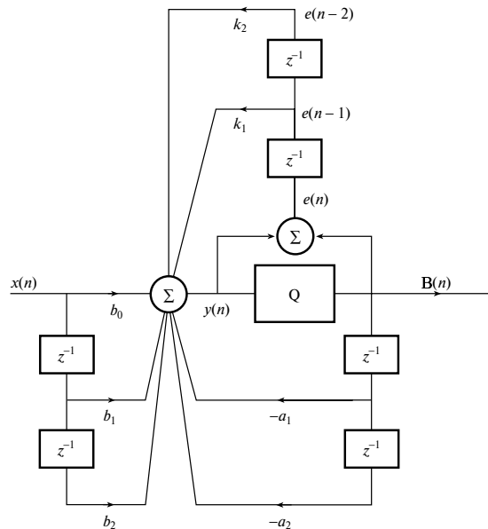
Рис. 13.26. Схема снижения шума второго порядка — выбор коэффициентов обратной связи по ошибке
