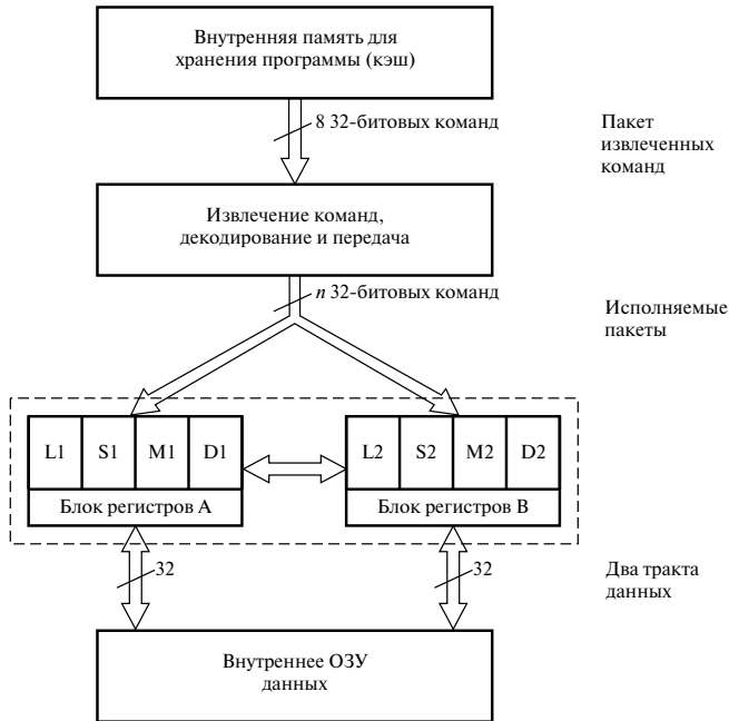
Рис. 12.13. Принципы архитектуры с командными словами сверхбольшой длины (Very Long Instruction Word — VLIW) и схема потока данных в процессорах TMS320C62x. Примечание: L1, L2 — логические элементы; S1, S2 — схемы сдвига/логические элементы; M1, M2 — умножители; D1, D2 — адресные элементы
