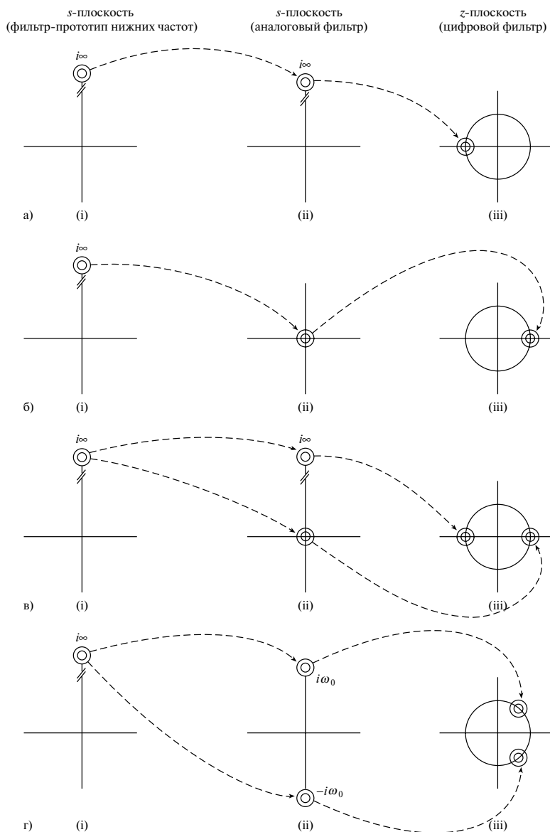
Рис. 8.17. Отображение нулей фильтра-прототипа нижних частот второго порядка в нули а) фильтра нижних частот; б) фильтра верхних частот; в) полосового фильтра; г) режекторного фильтра
