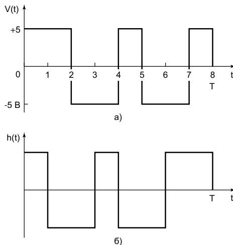
Рис. 5.12. Сигнал — 8-битовое кодовое слово PCM (панель а ). Импульсная характеристика соответствующего согласованного фильтра (панель б )
