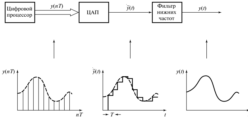
Рис. 2.39. Процесс цифроаналогового преобразования, который используется для восстановления аналогового сигнала после цифровой обработки. Заметим, что вход ЦАП — это серия импульсов, тогда как выход ЦАП имеет форму лесенки, поскольку каждый импульс не изменяется на протяжении времени T (s)
