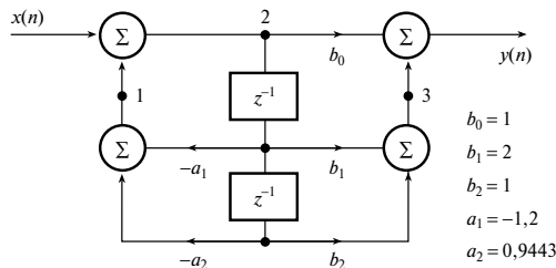
Рис. 13.31. Стандартное звено второго порядка (задача 13.1)
