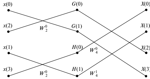
Рис. 3.18. Функциональная схема БПФ (пример 3.8)
