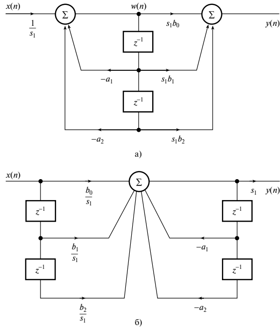
Рис. 13.9. Принципы масштабирования в звеньях второго порядка: а) каноническое звено; б) реализация в прямой форме
