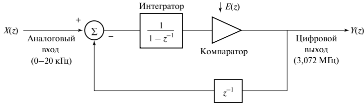
Рис. 2.33. Модель сигма-дельта-модулятора первого порядка на z -плоскости
