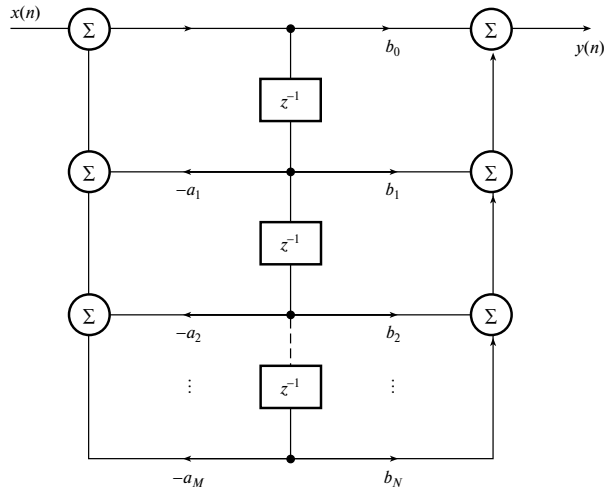
Рис. 8.24. Реализация БИХ-фильтра в прямой форме
