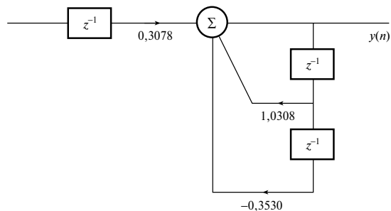
Рис. 8.6. Блок-схема фильтра из примера 8.4
