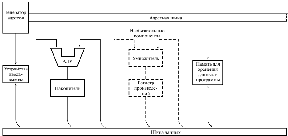
Рис. 12.1. Упрощенная архитектура стандартных микропроцессоров
