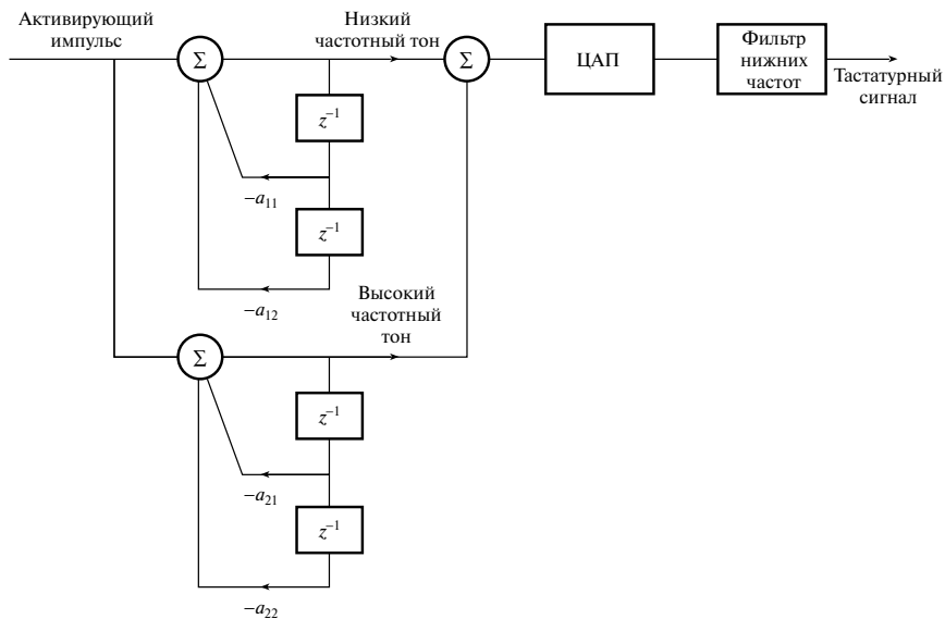
Рис. 8.38. Кнопочный генератор (согласно [17]). Код набранной цифры используется для выбора коэффициентов фильтра и начальных условий, а следовательно, частоты осциллятора
