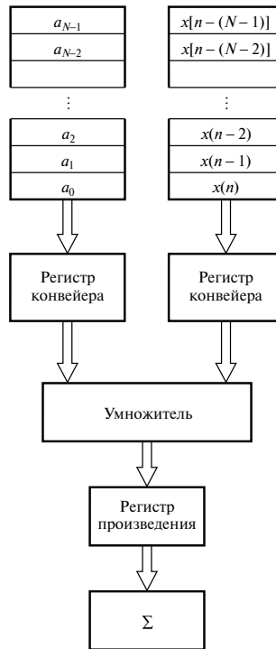
Рис. 12.8. Конфигурация умножителя-накопителя с конвейерной обработкой. Регистры конвейера используются как временное хранилище для коэффициентов и пар выборок данных. Регистр произведения также служит временным хранилищем произведения
