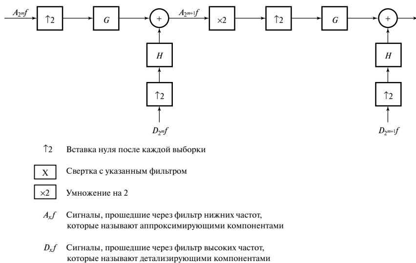
Рис. 3.11. Восстановление сигнала с помощью вейвлетного КА
