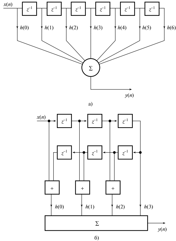
Рис. 7.29. Трансверсальная структура (панель а ); структура с линейной фазовой характеристикой фильтра из примера 7.17 (панель б )
