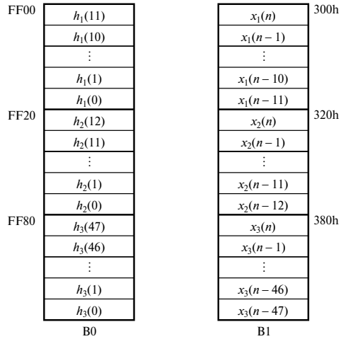
Рис. 12.36. Схемы хранения коэффициентов и данных трехкаскадного дециматора
