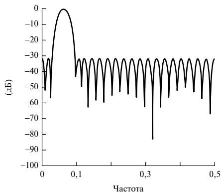
Рис. 7.13. Частотная характеристика фильтра (нормированная шкала частот)
