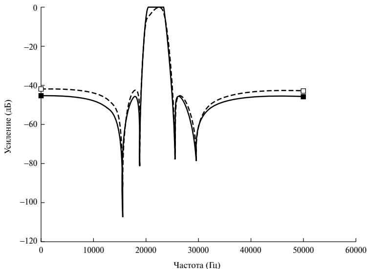
Рис. 8.30. Практическое влияние квантования коэффициентов на частотную характеристику: ■ — неквантованная характеристика; □ — квантованная характеристика (5 бит)
