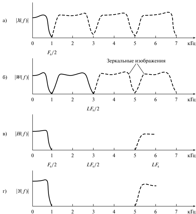
Рис. 9.4. Спектральная интерпретация интерполяции сигнала с 2 до 6 кГц
