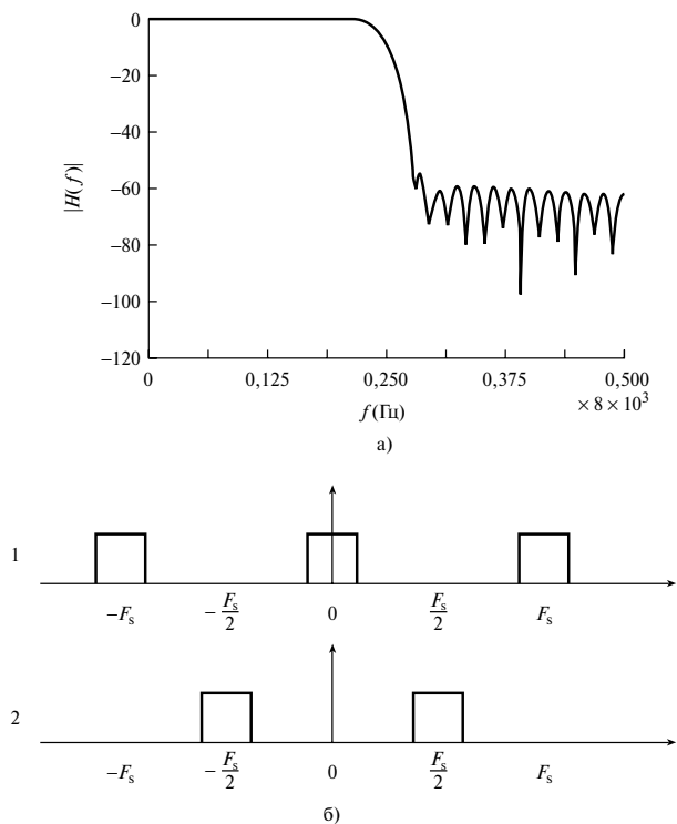
Рис. 7.26. Частотная характеристика полуполосного фильтра нижних частот (панель а). Частотная характеристика 1) идеального фильтра нижних частот; 2) эквивалентного идеального фильтра верхних частот (панель б)
