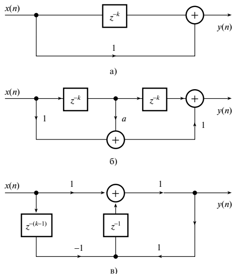
Рис. 7.27. Примеры примитивных блоков КИХ-фильтров: а) схема суммирования ( H(z) = 1 + z^{-k} ); б) схема двойного суммирования ( H(z) = az^{-k} + z^{-2k} ); чтобы избежать прямого умножения a = \pm 2^n , n — целое; умножение на целое число можно реализовать с помощью сдвигов); в) блок рекурсивной текущей суммы ( H(z) = (1 - z^{-k})/(1 - z^{-1}) = 1 + z^{-1} + z^{-2} + \dots + z^{-(k-1)} ).
