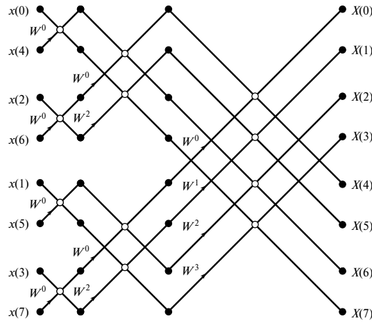
Рис. 13.28. Граф-схема 8-точечного двоичного алгоритма БПФ с децимацией во времени
