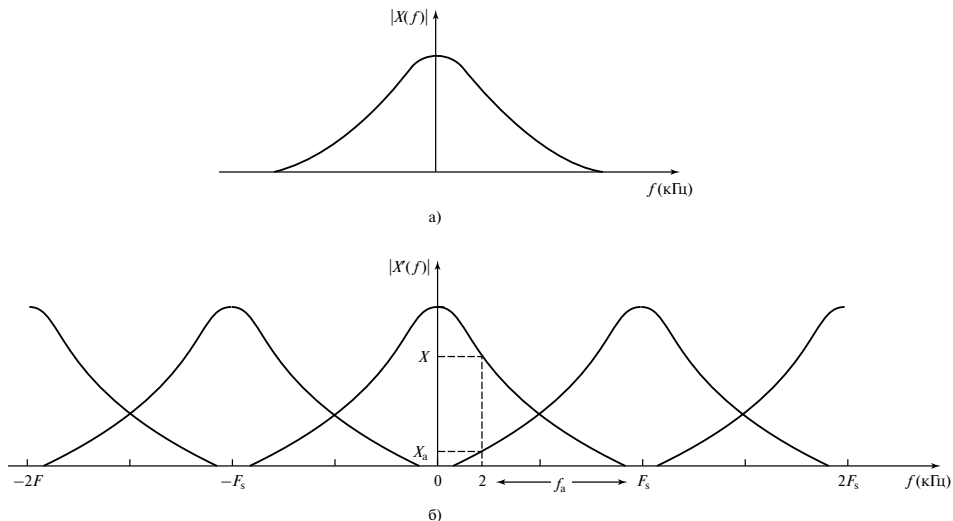
Рис. 2.11. Спектр сигнала а) на выходе аналогового фильтра и б) после дискретизации (пример 2.2)
