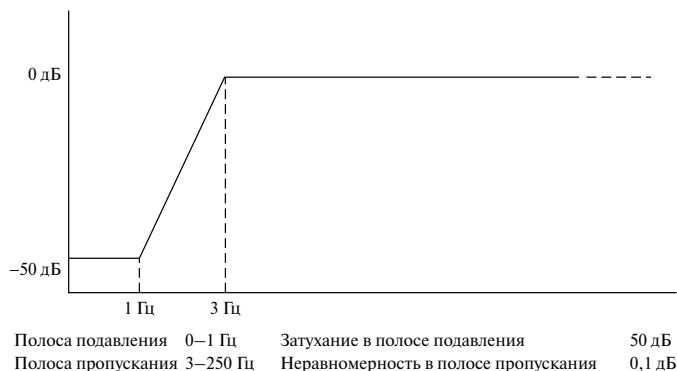
Рис. 14.22. Спецификация фильтра для устранения смещений базовой линии
