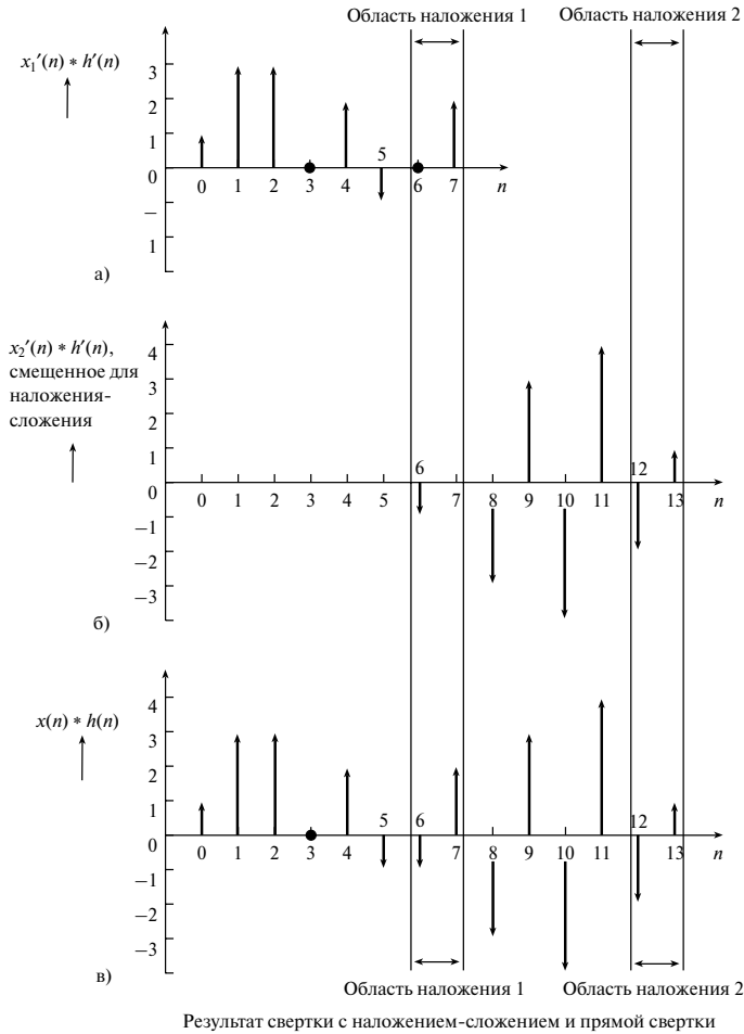
Рис. 5.31. Эквивалентность метода наложения-сложения и прямой свертки
