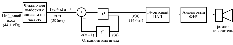
Рис. 2.59. Упрощенная блок-схема воспроизведения звукового сигнала проигрывателем компакт-дисков с четырехкратной выборкой с запасом по частоте и ограничением формы шума
