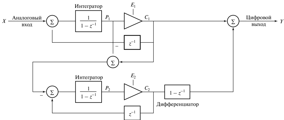
Рис. 2.37. Модель сигма-дельта-модулятора второго порядка на z -плоскости (пример 2.12)
