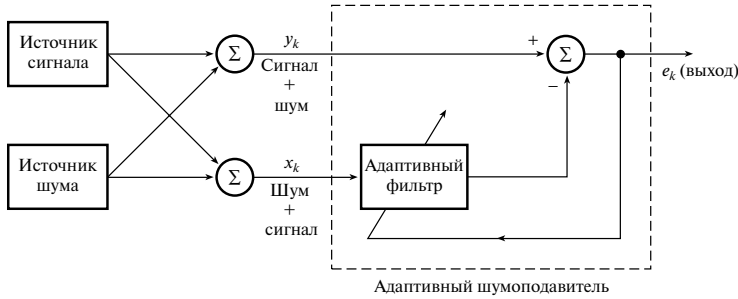
Рис. 10.13. Адаптивное шумоподавление при наличии компонентов сигнала в канале помехи и канале полезного сигнала
