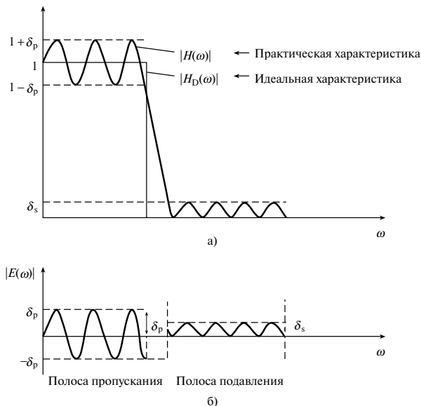
Рис. 7.11. Частотная характеристика оптимального фильтра нижних частот (панель а ). Характеристика ошибки между идеальной и практической характеристиками ( \delta_p = 2\delta_s ) (панель б )
