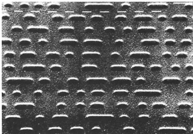
Рис. 1.12. Выжженные лазером впадины на компакт-диске. Ширина каждой впадины — 0,5 мкм, длина — 0,8–3,5 мкм, а глубина — 0,11 мкм. Расстояние между дорожками составляет 1,6 мкм. (Перепечатано с разрешения журнала Philips Technical Review , 40(6), 1982)
