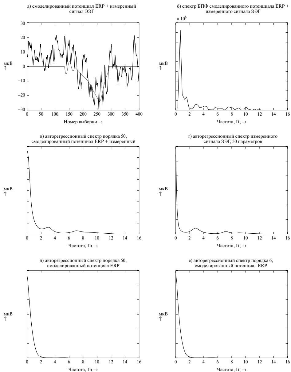
Рис. 11.21. Иллюстрация получения спектра авторегрессионным методом
