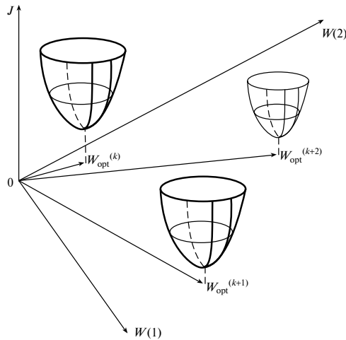
Рис. 10.11. Нестационарная поверхность производительности
