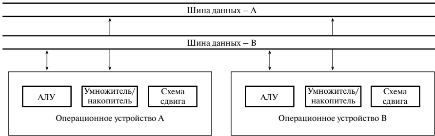
Рис. 12.11. Двойные арифметические устройства и двойные тракты передачи данных для обработки по схеме SIMD
