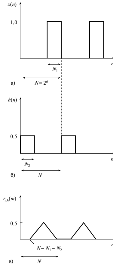
Рис. 5.29. Метод получения правильной взаимной корреляции двух последовательностей x(n) и h(n) : а) x(n) смещается в N - N_1 + 1 ; б) h(n) смещается в начало координат; в) получающийся правильный периодический коэффициент взаимной корреляции r_{xh}(m)
