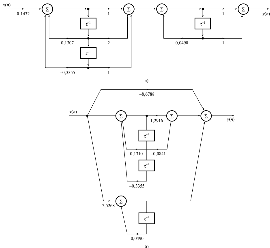
Рис. 8.29. Реализации фильтра из примера 8.20: а) каскадная; б) параллельная
