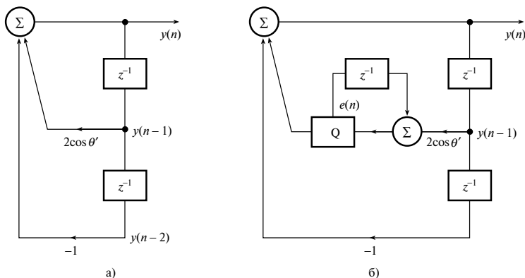
Рис. 8.35. Простой цифровой осциллятор (панель а); простой цифровой осциллятор со схемой формирования формы ошибки первого порядка (панель б)
