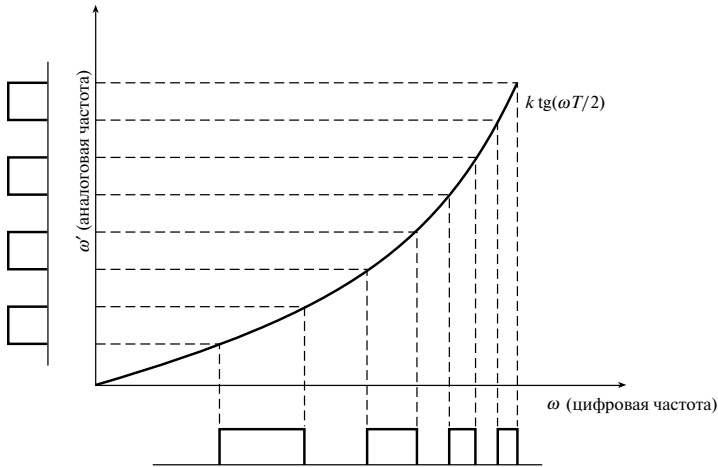
Рис. 8.10. Связь между аналоговыми и цифровыми частотами, демонстрирующая эффект деформации. Обратите внимание на то, что равноотстоящие аналоговые полосы после преобразования в цифровую область на высоких частотах сжимаются и располагаются плотнее
