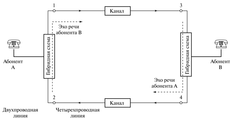
Рис. 1.19. Упрощенная схема телефонной цепи для больших расстояний
