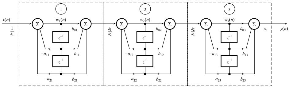
Рис. 13.11. Масштабирование в каскадной реализации БИХ-фильтра шестого порядка
