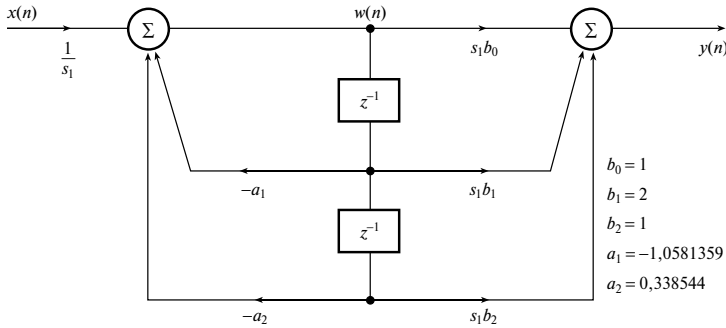
Рис. 13.10. Блок-схема фильтра (пример 13.9)
