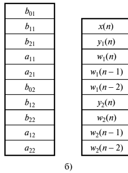
Рис. 12.29. Каскадная реализация БИХ-фильтра: а) диаграмма реализации; б) память для хранения данных и коэффициентов
