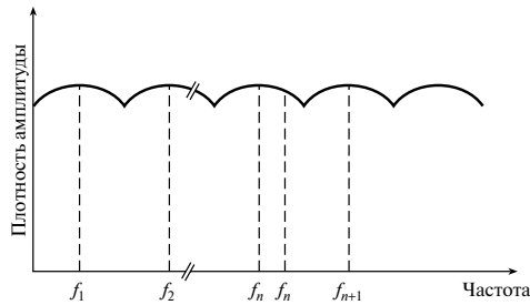
Рис. 11.1. Спектральная плотность амплитуды сигнала с равномерной спектральной плотностью
