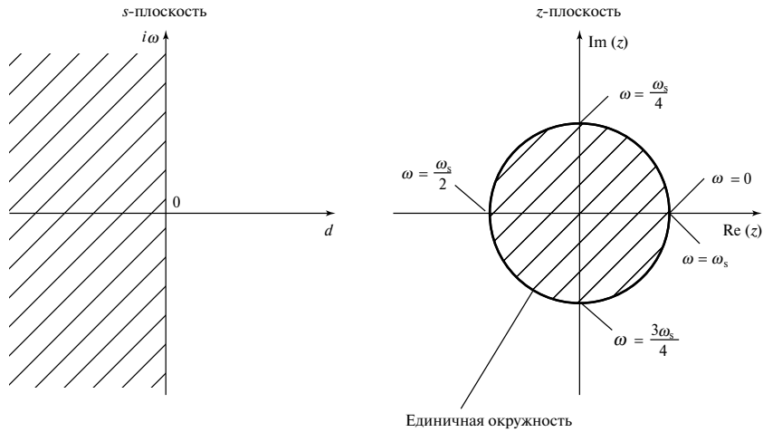
Рис. 4.5. Отображение s -плоскости в z -плоскость. Левая сторона s -плоскости отображается на внутреннюю часть z -плоскости, правая сторона отображается на внешнюю часть, а ось i\omega отображается на единичную окружность
