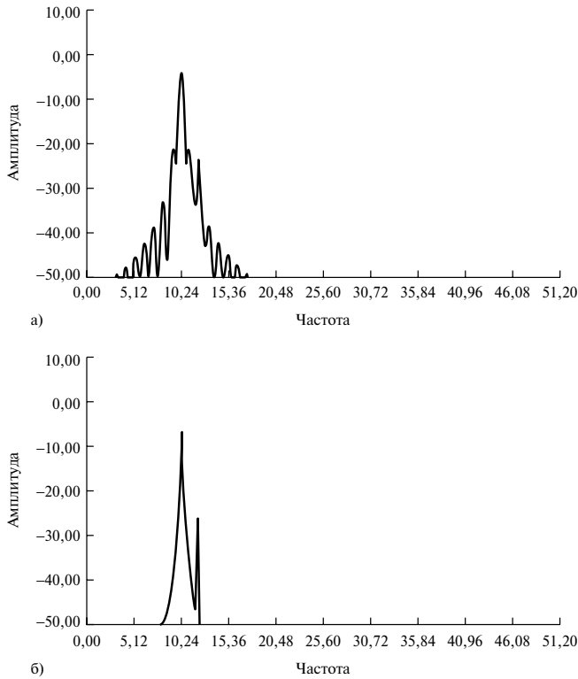
Рис. 11.11. Амплитудный спектр двух синусоид, умноженных на весовую функцию — конический косинус
