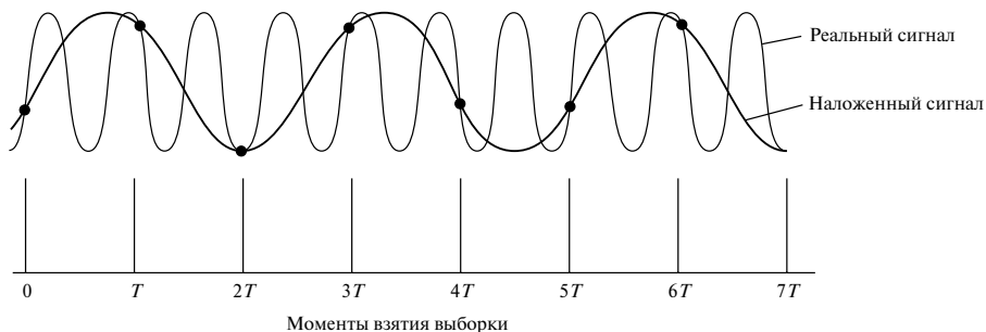
Рис. 2.4. Пример наложения во временных координатах. Обратите внимание на то, что оба сигнала имеют одинаковые значения в одних и тех же точках, хотя их частоты различны
