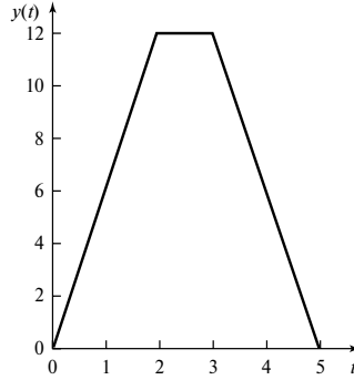
Рис. 5.22. Зависимость свертки y(t) = x(t) \otimes h(t) от t
