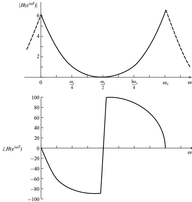
Рис. 4.11. Схематическое изображение частотной характеристики системы дискретного времени из примера 4.11
