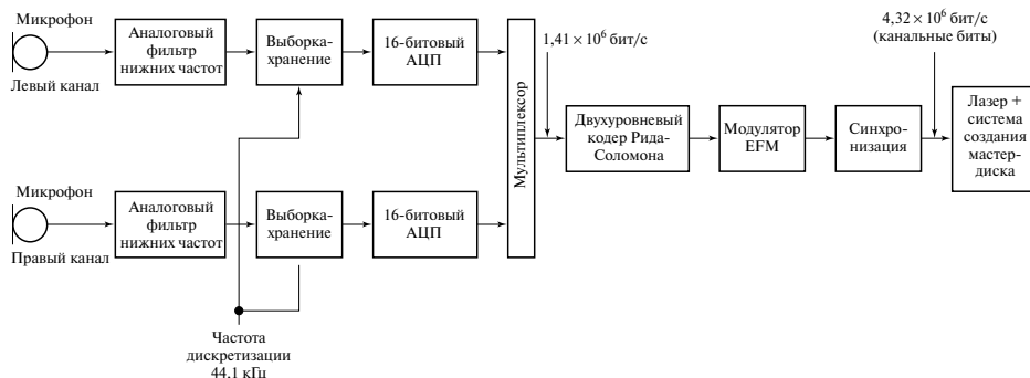
Рис. 1.13. Упрощенная блок-схема обработки аудиосигнала и записи его на компакт-диск
