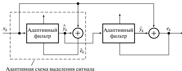
Рис. 10.21. Подавление помехи в приемнике DS/SS
