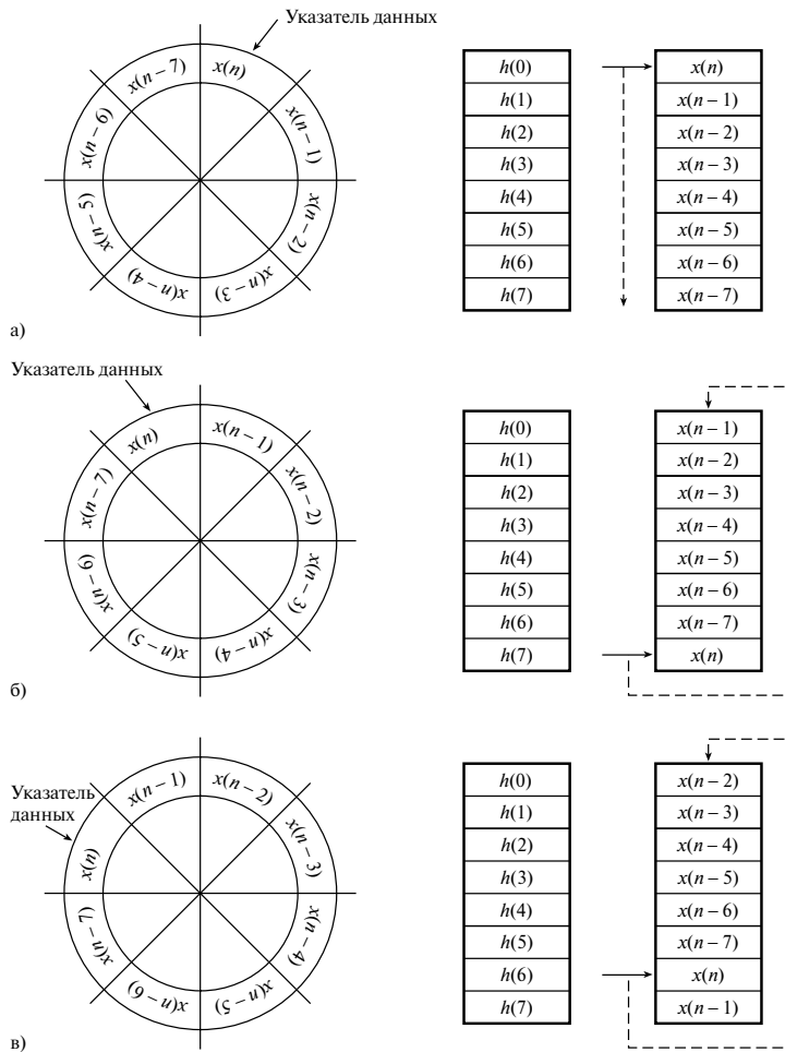
Рис. 12.26. Иллюстрация принципов реализации КИХ-фильтра на основе кругового буфера
