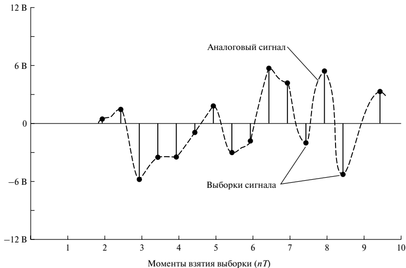
Рис. 2.3. Пример дискретного сигнала (идеальная дискретизация). Дискретные значения сигнала равны значениям исходного аналогового сигнала в эти моменты времени
