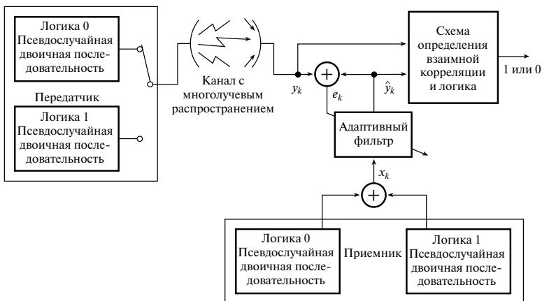
Рис. 10.20. Адаптивная система связи расширенного спектра с компенсацией многолучевого распространения
