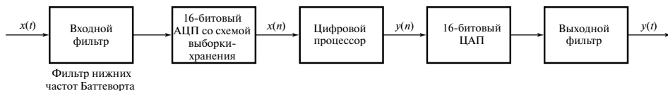
Рис. 2.47. Система цифровой обработки сигналов реального времени
