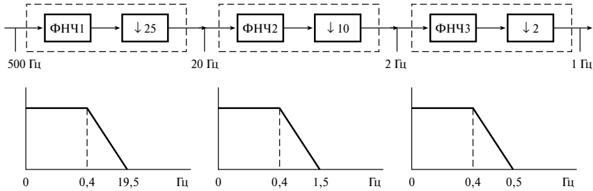
Рис. 9.37. Трехкаскадный дециматор из примера 9.9
