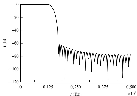
Рис. 7.9. Спектр фильтра, полученного с помощью функции Кайзера (пример 7.5)
