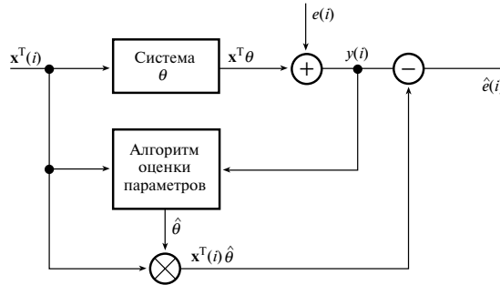
Рис. 14.11. Блок-схема устранения окулярных артефактов
