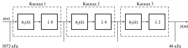
Рис. 9.10. Блок-схема дециматора из примера 9.2
