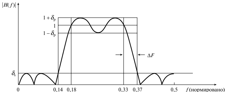
Рис. 6.5. Схема допусков для полосового фильтра из примера 6.2
