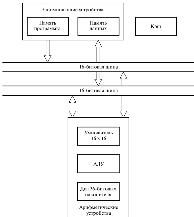
Рис. 12.19. Упрощенная архитектура процессора ЦОС с фиксированной запятой DSP16xx (Lucent Technologies)
