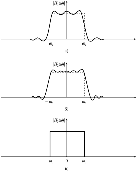
Рис. 7.5. Влияние на частотную характеристику округления идеальной импульсной характеристики до а) 13 коэффициентов; б) 25 коэффициентов; в) бесконечного числа коэффициентов
