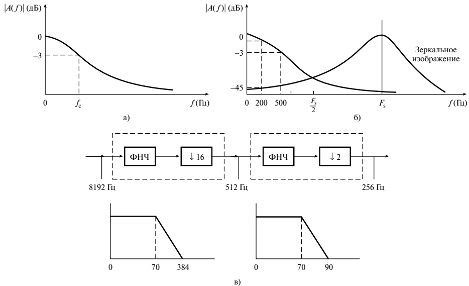
Рис. 9.29. Характеристика фильтра Баттерворта второго порядка (панель а). Спектр широкополосного сигнала после ограничения полосы и дискретизации (панель б). Двухкаскадный дециматор из примера 9.6 (панель в)
