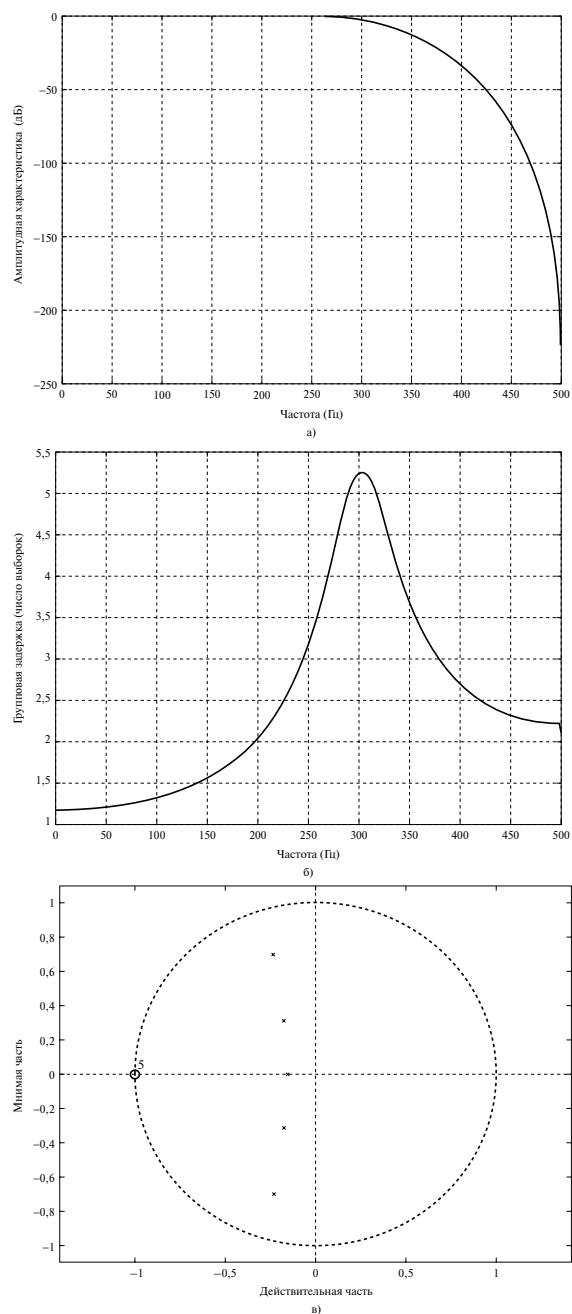
Рис. 8.20. Амплитудно-частотная характеристика билинейного z -преобразования (панель а); групповая задержка фильтра, полученного методом билинейного z -преобразования (панель б); диаграмма нулей и полюсов фильтра, полученного методом билинейного z -преобразования (панель в)
