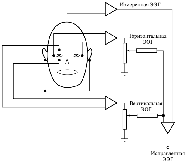
Рис. 14.12. Типичный пример автономных методов устранения артефактов [13]
