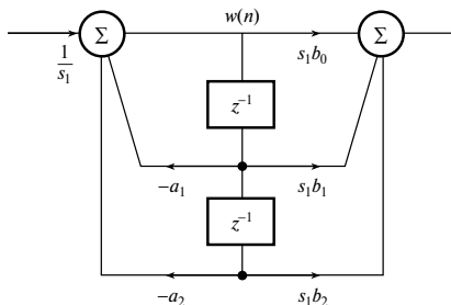
Рис. 13Б.1. Стандартное каноническое звено фильтра
