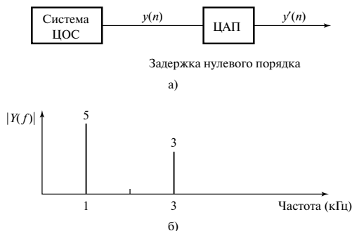
Рис. 2.56. Система ЦОС реального времени с аналоговым выходом (панель а); спектр сигнала, который подается на ЦАП (панель б)
