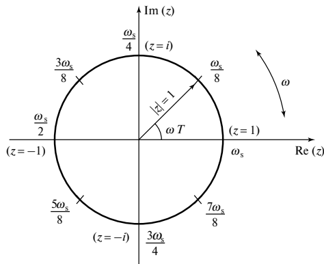
Рис. 4.12. Единичная окружность z -плоскости, на которой показаны критические точки частоты
