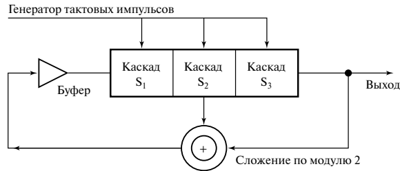
Рис. 5.15. Трехкаскадный генератор псевдослучайной последовательности
