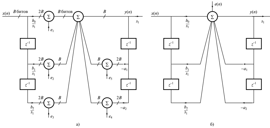
Рис. 13.16. Модель шума квантования произведения для фильтрующего звена, реализованного в прямой форме. Все источники шума, представленные на панели а , на панели б объединены, поскольку выход с них поступает в одну точку
