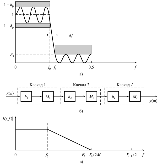
Рис. 9.9. Схема допусков фильтра нижних частот с равными колебаниями характеристики (панель а); многокаскадная структура (панель б); спецификации фильтра i -го каскада, i = 1, 2, \dots, I (панель в)
