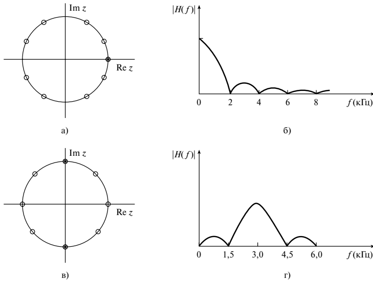
Рис. 7.24. Диаграмма нулей и полюсов (панель а ). Схематическое изображение амплитудной характеристики рекурсивного КИХ-фильтра с целыми коэффициентами (панель б ). Диаграмма нулей и полюсов для простого полосового фильтра с целыми коэффициентами (панель в ). Соответствующая амплитудная характеристика (панель г )
