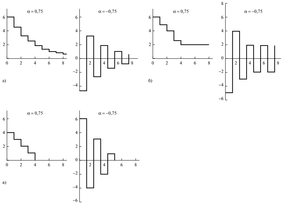
Рис. 13.27. Иллюстрация низкоуровневого граничного цикла, порожденного квантованием произведений БИХ-фильтра первого порядка: а — бесконечная точность; б — квантование через округление; в — квантование через усечение
