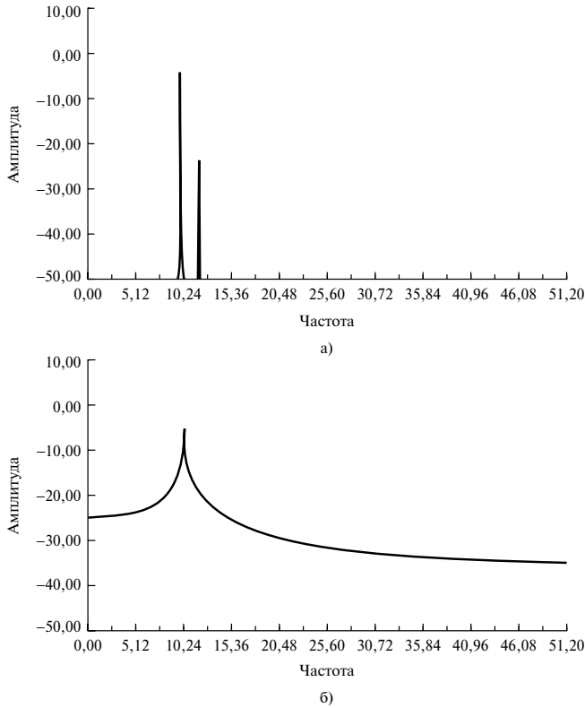
Рис. 11.9. Амплитудный спектр двух синусоид, отличающихся по амплитуде на 40 дБ: а) длина окна кратна обоим периодам; б) длина окна не кратна одному из периодов (большему)
