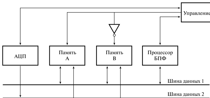
Рис. 12.42. Двойная буферизация в БПФ реального времени
