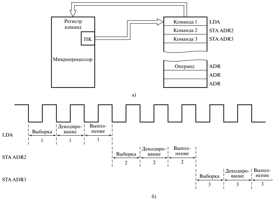
Рис. 12.3. Иллюстрация выборки, декодирования и выполнения команды в негарвардской архитектуре с единой областью памяти: а) вызов команды из памяти; б) временная диаграмма процесса
