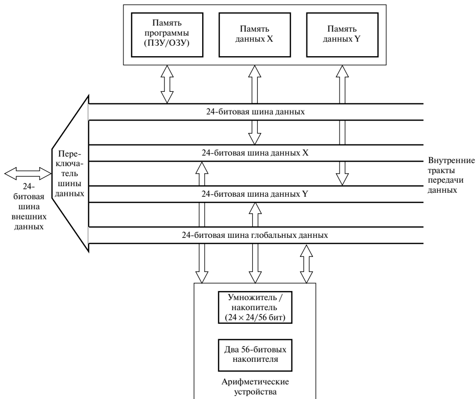
Рис. 12.17. Упрощенная архитектура процессора ЦОС с фиксированной запятой второго поколения (Motorola DSP56002)
