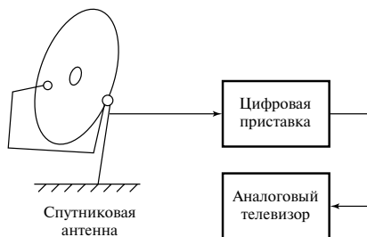
Рис. 1.18. Использование цифровой приставки для приема сигнала цифрового телевидения
