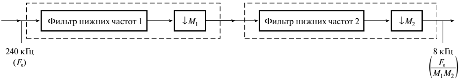
Рис. 9.12. Двухкаскадный дециматор
