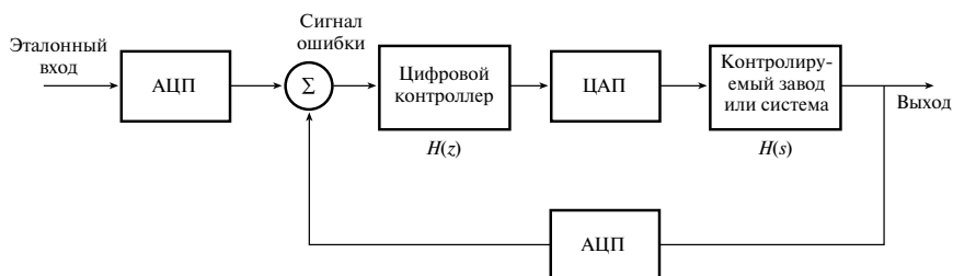
Рис. 8.34. Принципы цифрового управления аналоговым оборудованием
