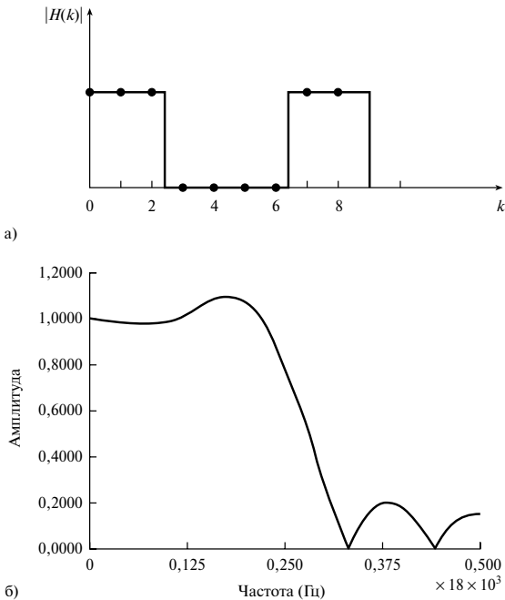
Рис. 7.18. Идеальная частотная характеристика, на которой показаны точки выборки (панель а). Частотная характеристика фильтра, построенного по принципу частотной выборки (панель б)
