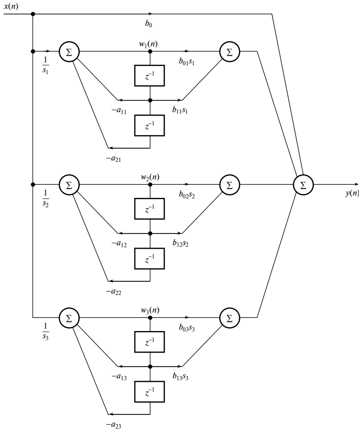
Рис. 13.13. Масштабирование в параллельной реализации БИХ-фильтра шестого порядка
