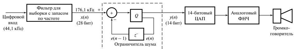
Рис. 2.42. Упрощенная блок-схема воспроизведения аудиосигнала в проигрывателе компакт-дисков с четырехкратной перевыборкой и формированием спектра шума
