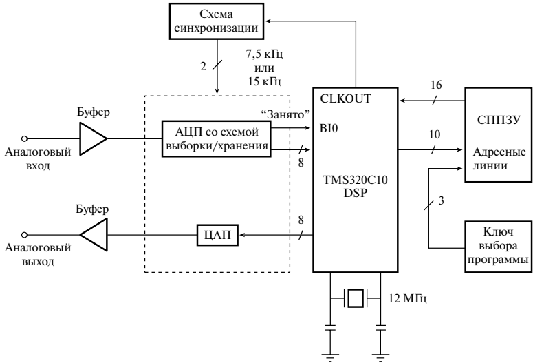
Рис. 14.1. Простая блок-схема целевой платы TMS320C10
