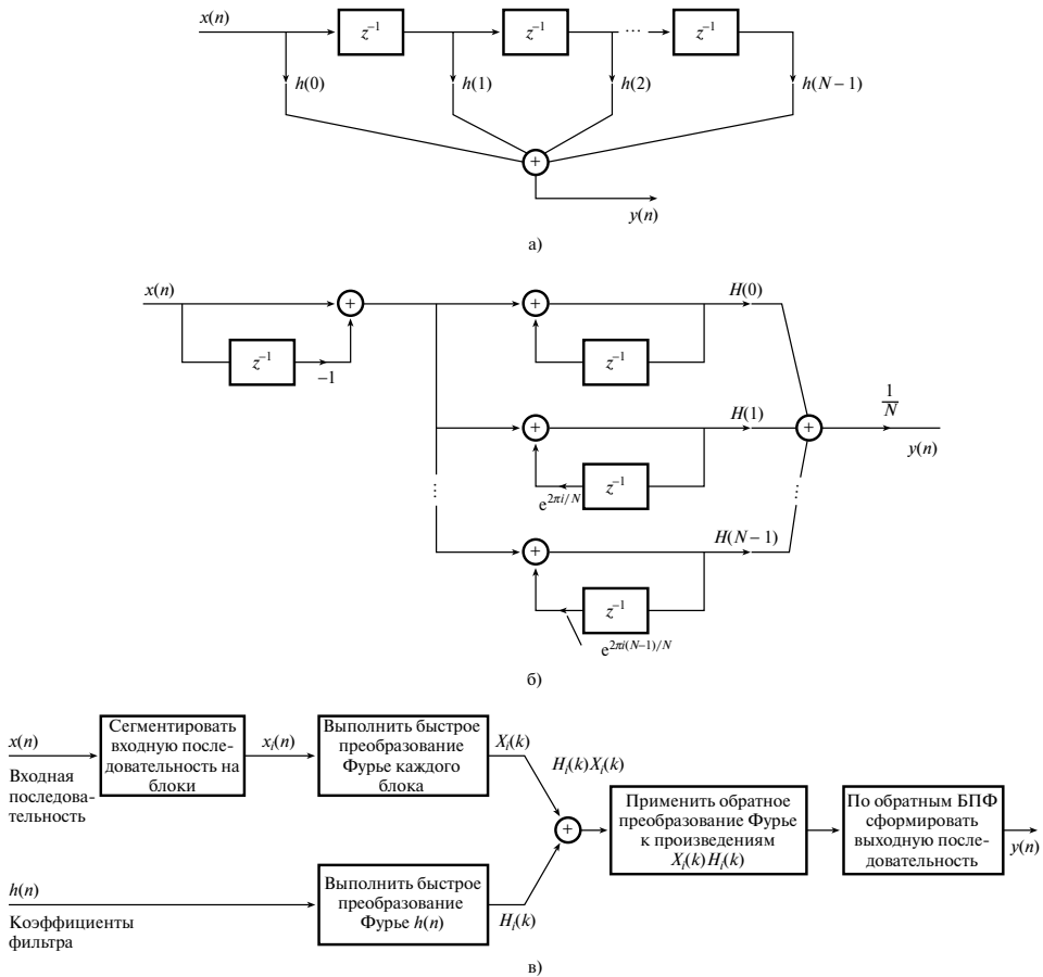
Рис. 6.7. Структуры реализации КИХ-фильтров: а) трансверсальный фильтр (прямая структура); б) реализация частотной выборки; в) схема быстрой свертки
