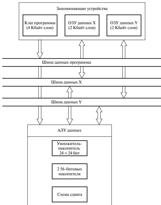
Рис. 12.21. Упрощенная архитектура процессора ЦОС с фиксированной запятой третьего поколения (Motorola DSP56300)
