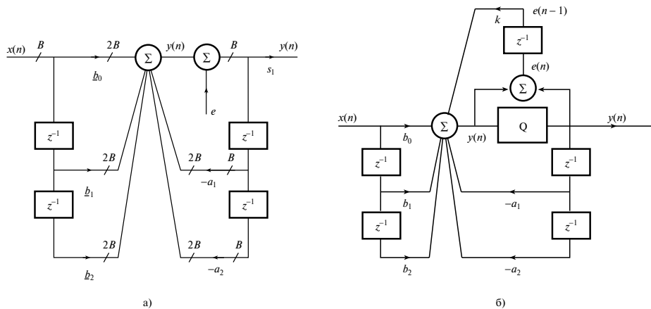
Рис. 13.21. Шум округления в звене второго порядка прямой формы I: a — длины слов в различных точках фильтра; б — схема снижения шума первого порядка
