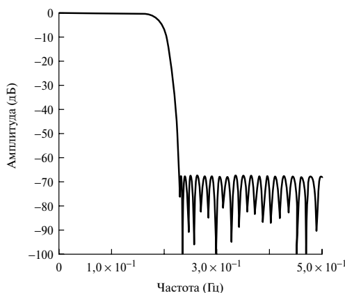
Рис. 7.33. Спектр фильтра до квантования (пример 7.19)
