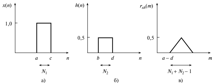
Рис. 5.27. Взаимная корреляция r(m) двух сигналов x(n) и h(n) , которые начинаются не в начале координат: а) x(n) ; б) h(n) ; в) r_{xh}(m)
