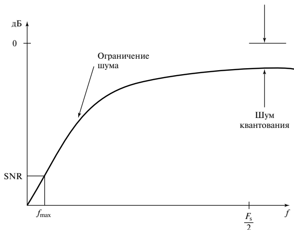
Рис. 2.38. Влияние схемы формирования спектра шума на шум квантования
