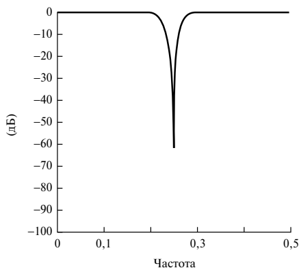
Рис. 7.14. Характеристика фильтра (нормированная шкала частот)
