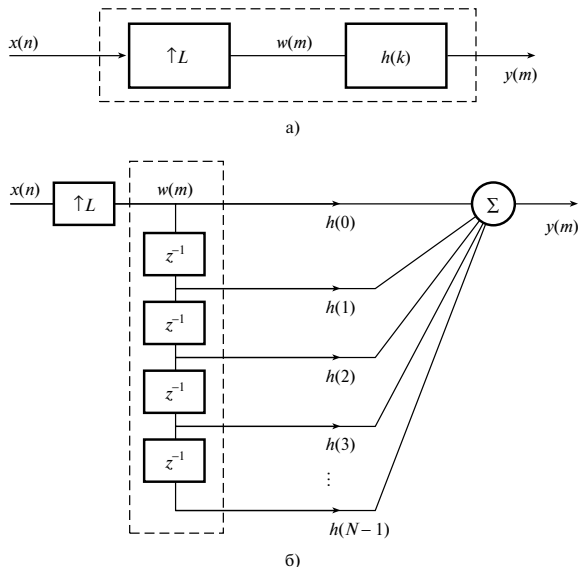
Рис. 9.16. Блок-схема интерполятора (панель а); функциональная схема интерполятора (панель б)
