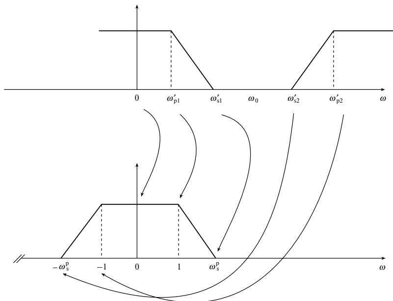
Рис. 8.16. Связь частот денормированного режекторного фильтра и фильтра нижних частот, используемого при разработке как прототип
