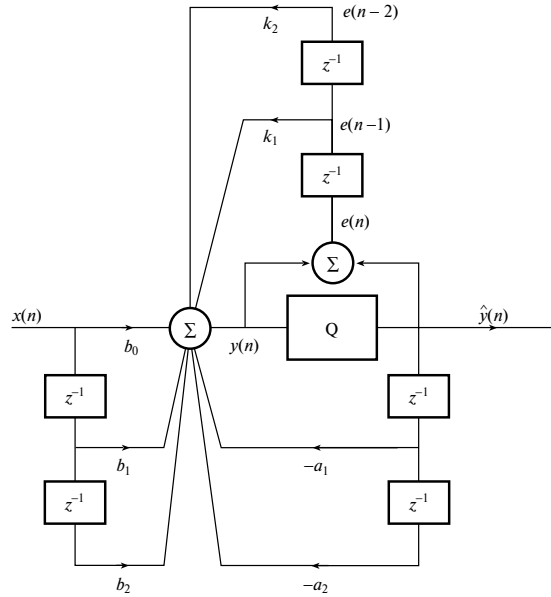
Рис. 13.23. Схема снижения шума второго порядка
