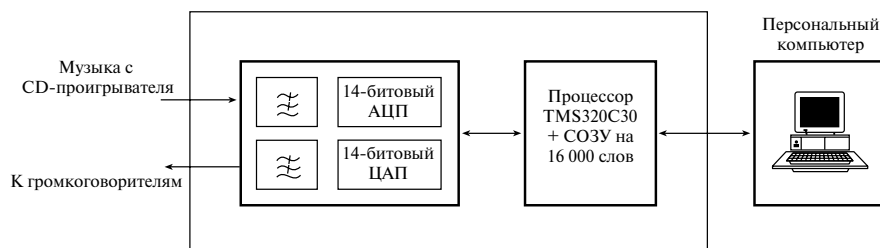
Рис. 14.19. Упрощенная блок-схема демонстрационного модуля TMS320C30
