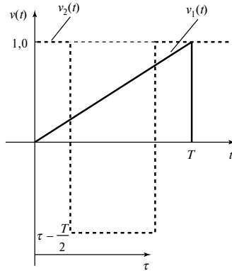
Рис. 5.8. Сегменты v_2(t) для T/2 \leq \tau \leq T
