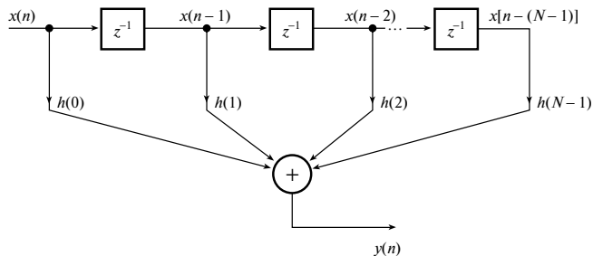
Рис. 7.28. Трансверсальная структура фильтра
