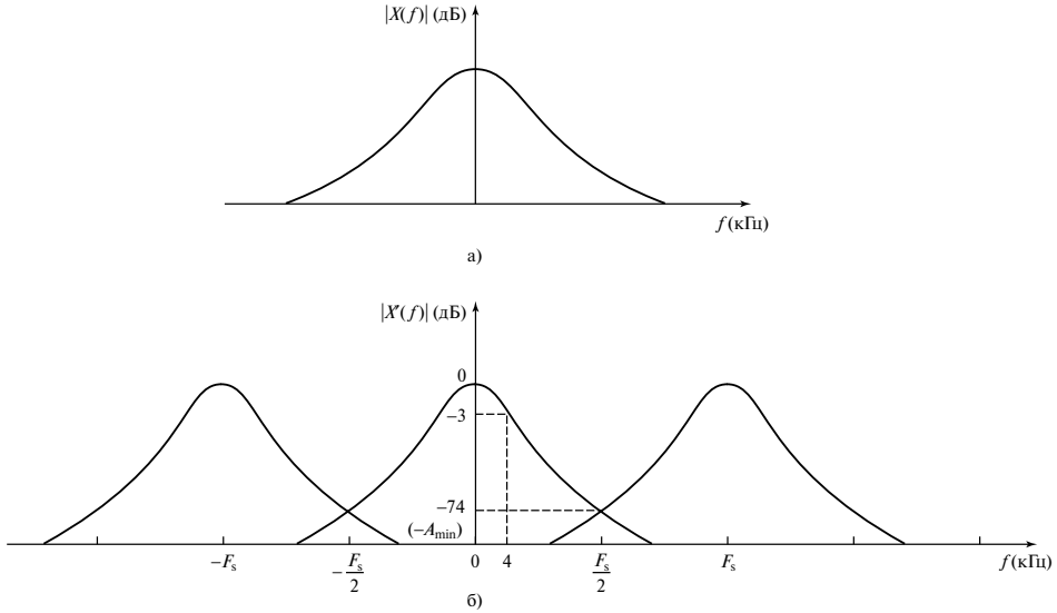
Рис. 2.14. Спектр сигнала: а) на выходе аналогового фильтра; б) после дискретизации (пример 2.3)
