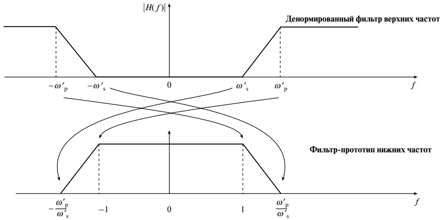
Рис. 8.14. Связь частот денормированного ФВЧ и ФНЧ-прототипа
