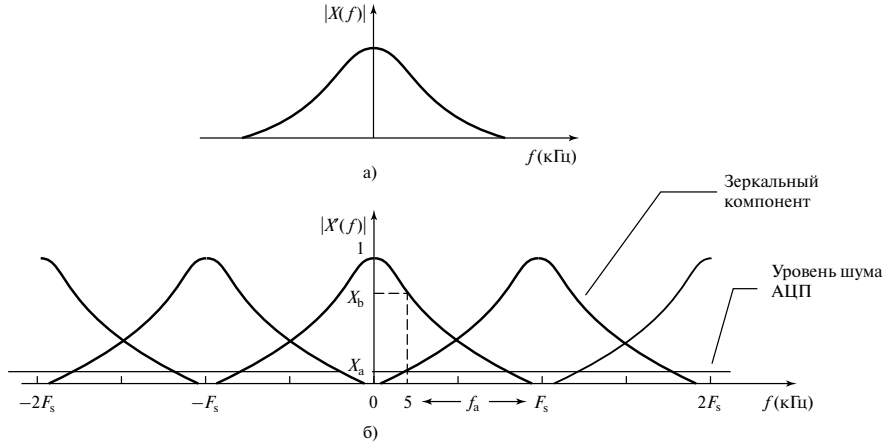
Рис. 2.15. Спектр дискретного сигнала, на котором показано искажение, вызванное наложением и квантованием АЦП (пример 2.4)
