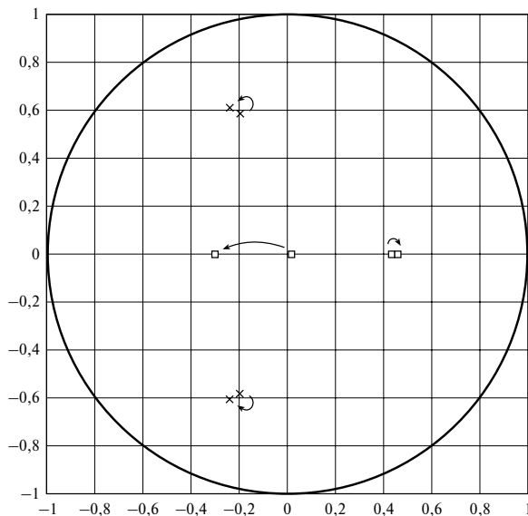
Рис. 8.22. Сравнение графиков нулей и полюсов фильтров, полученных путем согласованного z -преобразования и усредненного согласованного/билинейного z -преобразования. Стрелочками указано движение полюсов/нулей при переходе от первого фильтра ко второму
