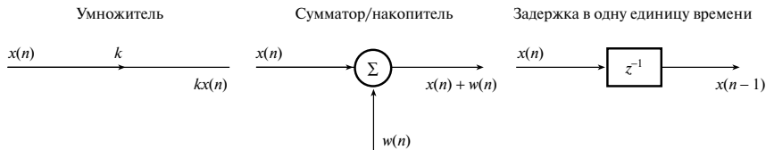
Рис. 8.23. Основные элементы структуры фильтра
