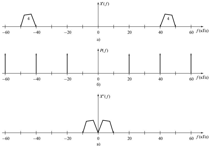
Рис. 2.19. Выход полосового фильтра (панель а ); функция дискретизации (панель б ); выход устройства дискретизации (панель в ) (пример 2.6)
