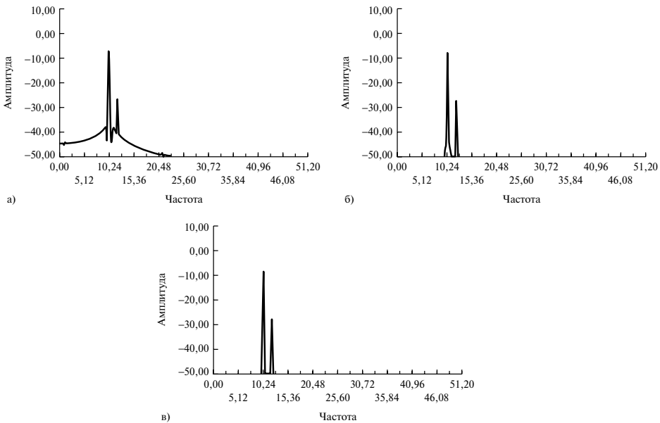
Рис. 11.14. Амплитудный спектр двух синусоид, вычисленный с использованием соответствующих функций Кайзера–Бесселя, представленных на рис. 11.13: а) \alpha = 2, 0 ; б) \alpha = 3, 0 ; в) \alpha = 4, 0
