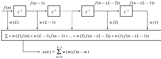
Рис. 5.24. Трансверсальный фильтр w(n) для слепой свертки
