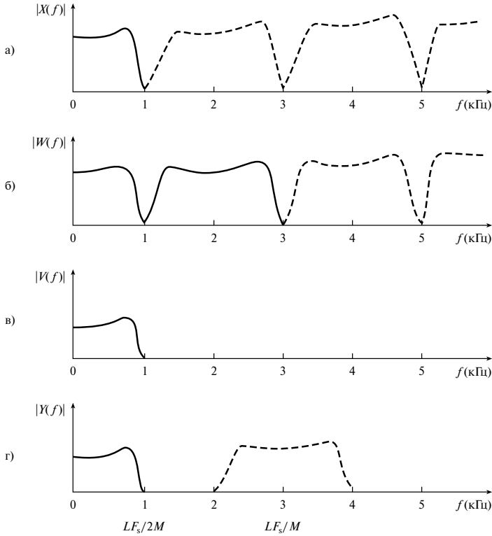
Рис. 9.6. Спектральная интерпретация увеличения частоты дискретизации с 2 кГц в 3/2 раза. Вначале скорость передачи сигнала увеличивается в 3 раза до 6 кГц (панель а); после ограничения по полосе для устранения наложения (панель в) скорость передачи сигнала уменьшается в 2 раза до 3 кГц
