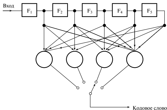
Рис. 5.39. Сверточный кодер
