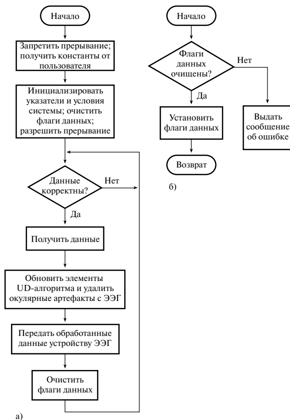
Рис. 14.14. Программное обеспечение системы устранения окулярных артефактов: а) основная программа; б) служебная программа прерывания
