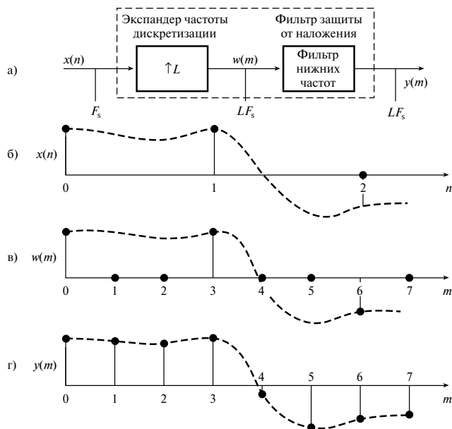
Рис. 9.3. Иллюстрация интерполяции с шагом L = 3 во временной области. Обратите внимание на то, что для каждой выборки x(n) получаются три выходные выборки y(m)
