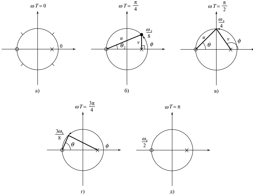
Рис. 4.10. Оценка частотной характеристики с помощью геометрического метода и диаграмма нулей и полюсов
