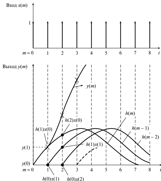
Рис. 5.19. Поданная на вход импульсная последовательность и характеристика системы, полученная из отдельных импульсных откликов
