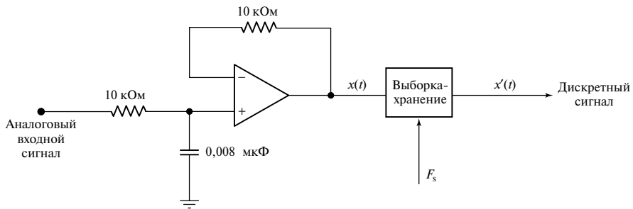
Рис. 2.10. Устройство предварительной обработки в простой системе сбора данных. Простой активный фильтр ограничивает полосу частот сигнала перед дискретизацией с частотой F_s
