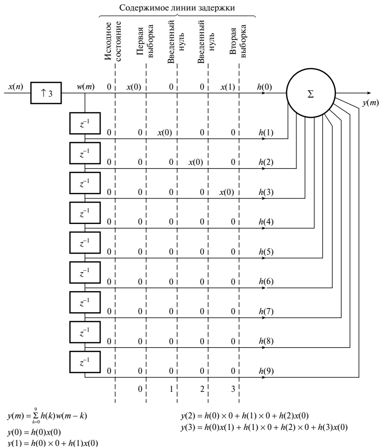
Рис. 9.17. Иллюстрация процесса интерполяции для простого случая L = 3
