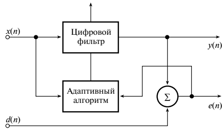
Рис. 12.37. Общая структура адаптивного фильтра: пара входов и пара выходов
