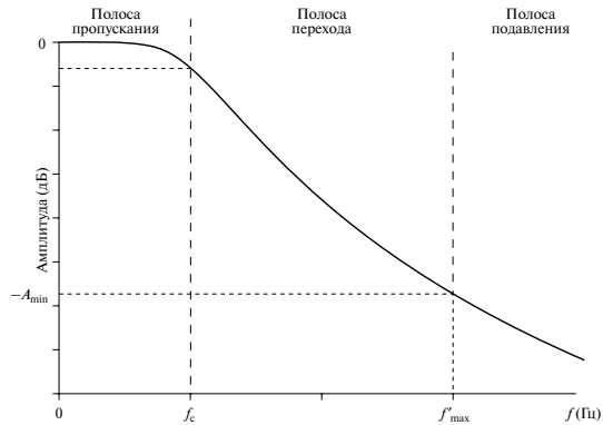
Рис. 2.13. Типичная амплитудно-частотная характеристика реального фильтра защиты от наложения спектров
