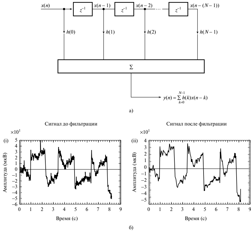
Рис. 1.4. Блок-схема трансверсального фильтра. Здесь h(k), k = 0, 1, \dots, N-1 — коэффициенты фильтра, а каждый квадрат с z^{-1} обозначает задержку на один интервал дискретизации (панель а); цифровая низкочастотная фильтрация биомедицинского сигнала с целью устранения шума (панель б)
