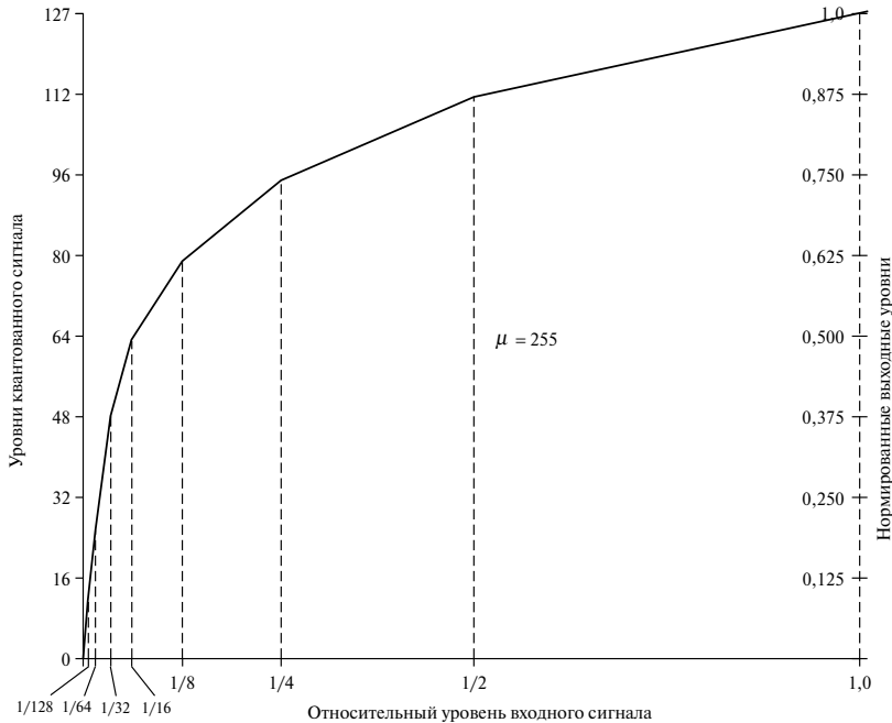
Рис. 2.27. Характеристики компандирования для \mu -характеристики с \mu = 255 ([ITU, 1998]). Характеристики подчиняются уравнению F(x) = \text{sgn}(x) \frac{\ln(1+\mu|x|)}{\ln(1+\mu)} , где \mu = 255 , x — нормированный входной сигнал, \text{sgn} — его знак, а F(x) — сжатый выходной сигнал
