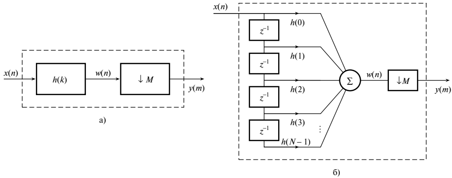
Рис. 9.13. Простая блок-схема дециматора (панель а); функциональная схема прохождения сигнала через дециматор (панель б)
