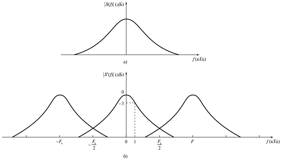
Рис. 2.29. Спектр входного сигнала: а) до дискретизации; б) после дискретизации
