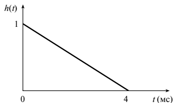
Рис. 5.40. Импульсная характеристика системы (задача 5.12)
