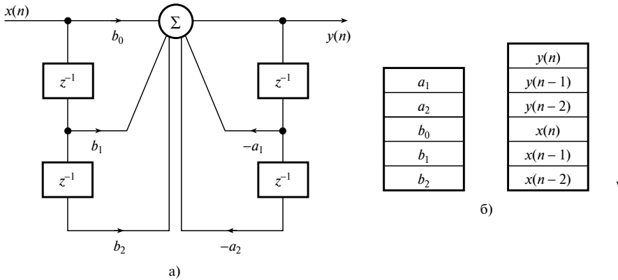
Рис. 12.28. Реализация звена второго порядка в прямой форме: а) диаграмма реализации; б) память для хранения данных и коэффициентов
