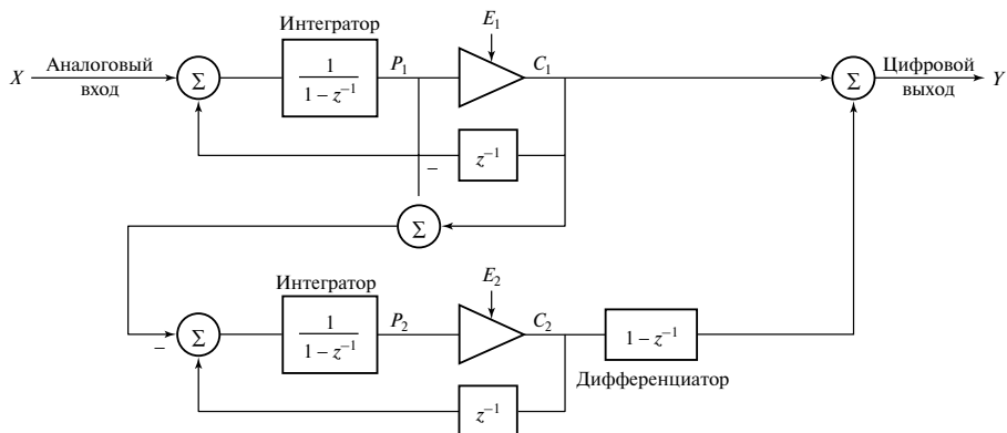
Рис. 2.54. Результат преобразования Y(z) на выходе сигма-дельта-модулятора второго порядка задается как Y(z) = X(z) + E_2(z)(1 - z^{-1})^2
