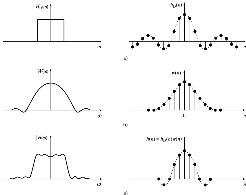
Рис. 7.6. Иллюстрация определения коэффициентов фильтра h(n) с помощью метода взвешивания
