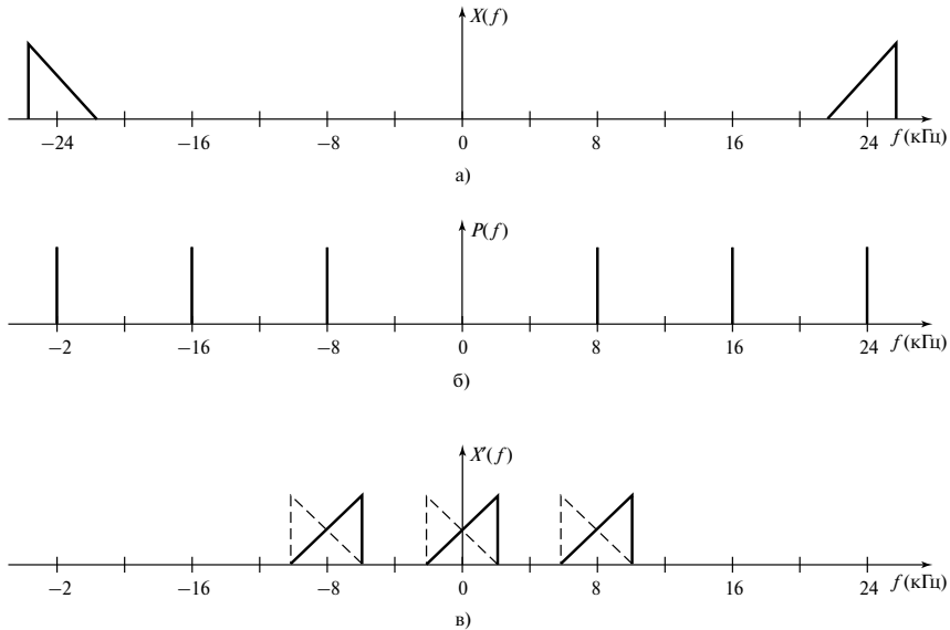
Рис. 2.24. Спектр дискретного сигнала ( n = f_H/B = 6,5 ) (пример 2.7, вариант 3)
