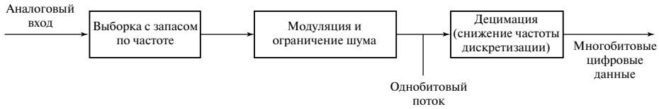
Рис. 2.31. Принципы (однобитового) аналого-цифрового преобразования с запасом по частоте
