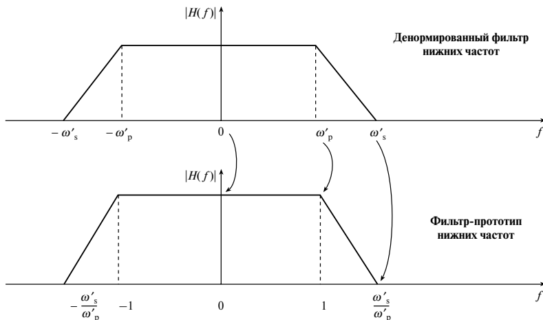
Рис. 8.13. Связь между частотами денормированного ФНЧ и ФНЧ-прототипа
