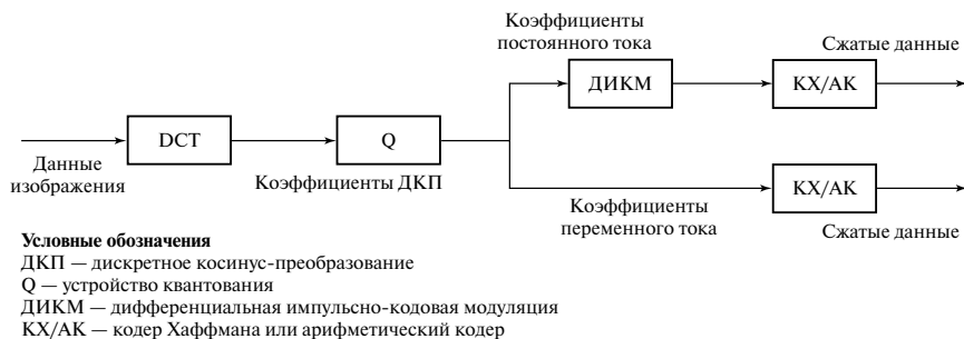
Рис. 3.16. Сжатие данных в стандарте JPEG
