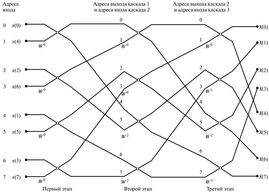
Рис. 12.33. Двоичное БПФ с постоянной геометрией, где вычисления выполняются без замещения ячеек памяти. Обратите внимание на то, что для каждой “бабочки” расстояние между входами и выходами одинаковое
