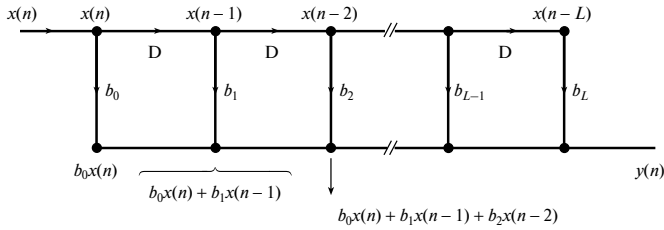
Рис. 5.38. Представление нерекурсивного фильтра в диаграммной форме
