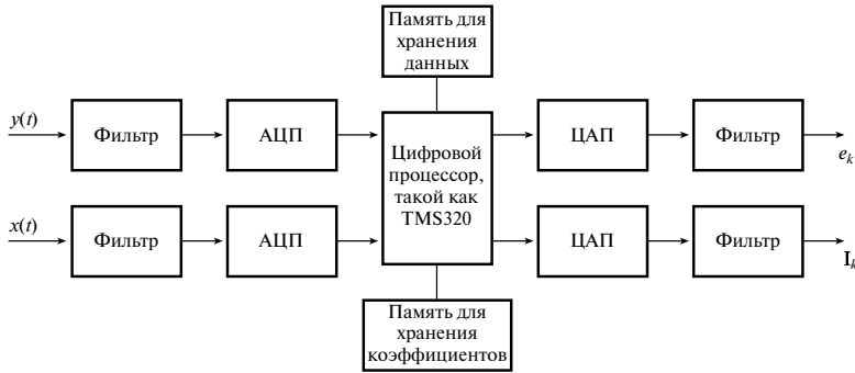
Рис. 10.10. Аппаратная реализация адаптивной фильтрации реального времени по схеме наименьших квадратов
