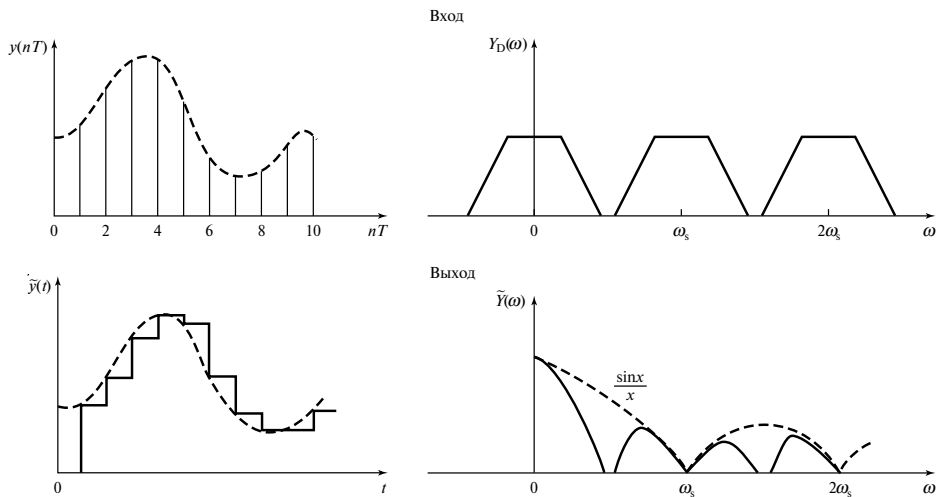
Рис. 2.40. Входной и выходной сигналы ЦАП в частотных и временных координатах. Заметим, что изменение характеристики по закону \sin x/x можно представить гипотетическим фильтром нижних частот
