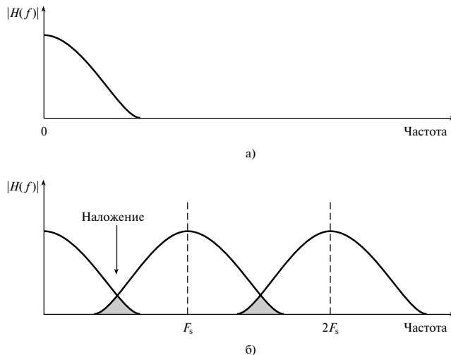
Рис. 8.8. Спектр аналогового фильтра (панель а ); спектр эквивалентного цифрового фильтра, полученного методом инвариантного преобразования импульсной характеристики, на котором виден эффект наложения (панель б )
