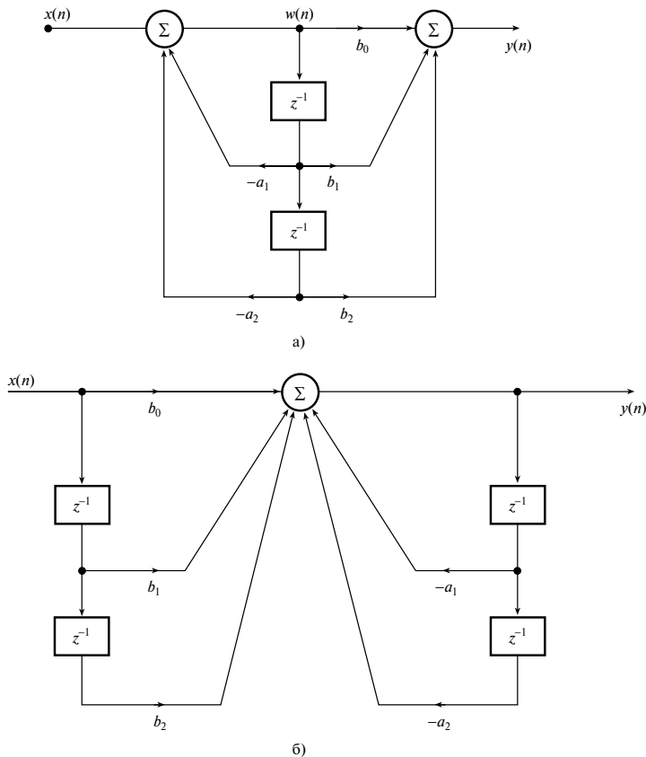
Рис. 8.25. Стандартные блоки структуры реализации БИХ-фильтров: а) каноническое звено второго порядка; б) звено второго порядка в прямой форме
