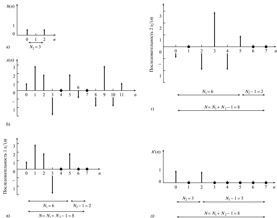
Рис. 5.30. Свертка методом наложения-сложения
