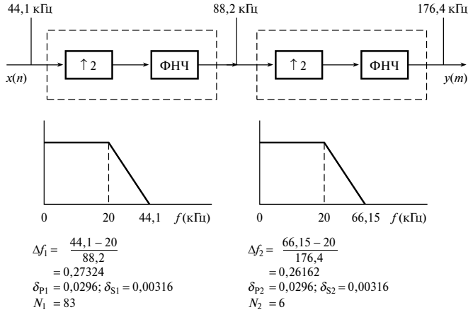
Рис. 9.27. Двухкаскадный интерполятор из примера 9.5
