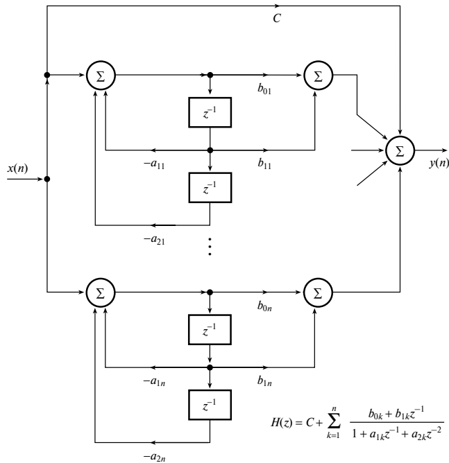
Рис. 8.28. Параллельная реализация
