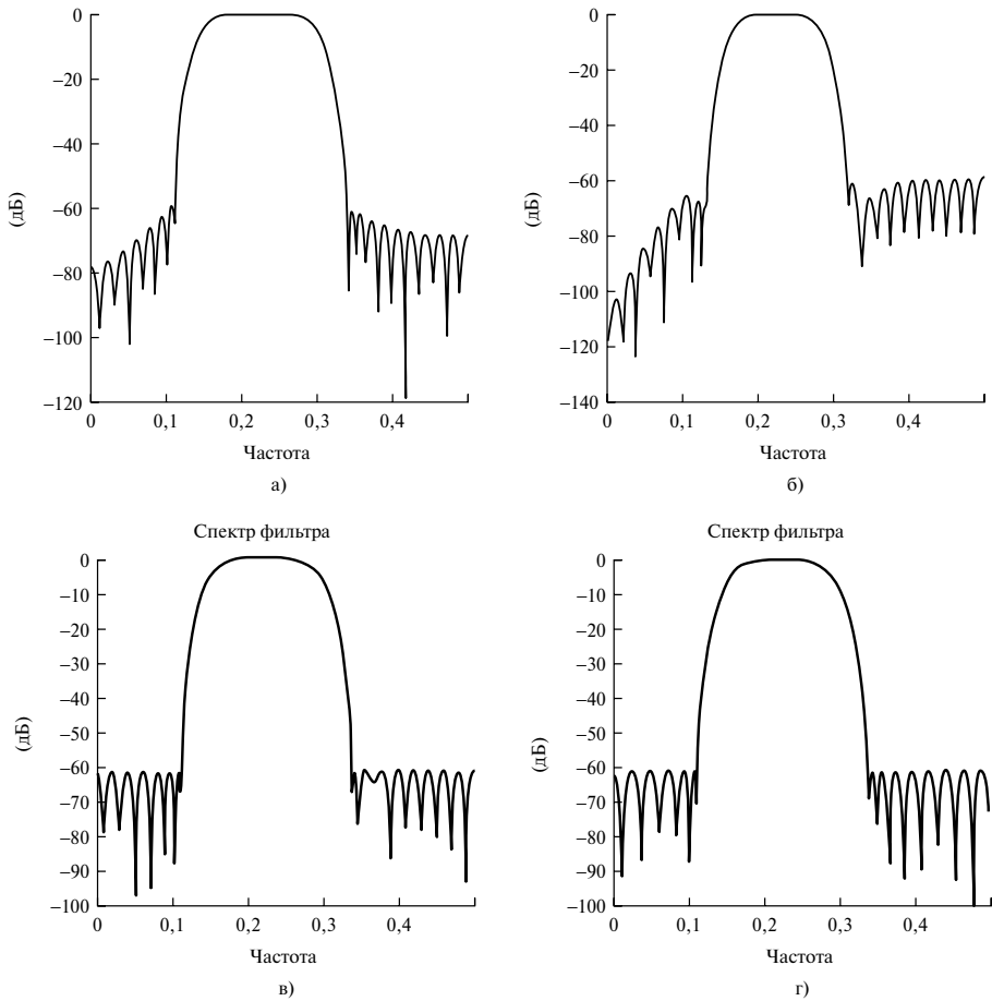
Рис. 7.25. Сравнение частотных характеристик фильтров, полученных с использованием метода взвешивания, метода частотной выборки и оптимального метода: а) характеристика фильтра, полученного с помощью функции Кайзера (фильтры 1 и 2); б) характеристика фильтра, полученного с помощью частотной выборки (фильтры 1 и 2); в) характеристика фильтра, полученного с помощью оптимального метода (фильтр 1); г) характеристика фильтра, полученного с помощью оптимального метода (фильтр 2)
