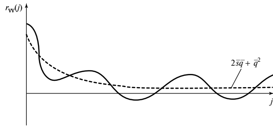
Рис. 5.11. Автокорреляционная функция зашумленного сигнала
