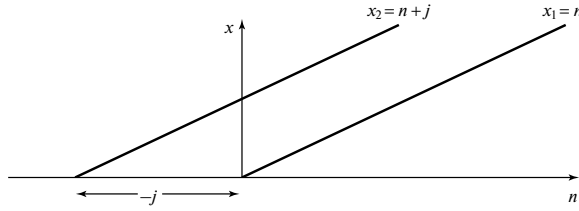
Рис. 5.2. Сигнал x_2 = x_1 + j , смещенный на j промежутков времени влево от сигнала x_1
