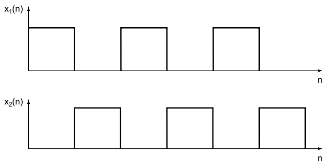
Рис. 5.1. Сигналы со 100%-ной корреляцией, идущие не в фазе, — при нулевой задержке корреляция равна нулю
