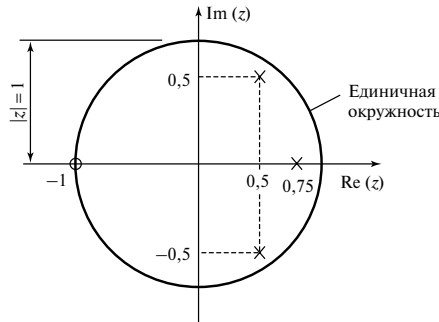
Рис. 4.6. Описание z -преобразования в виде диаграммы нулей и полюсов: X — полюс; O — нуль
