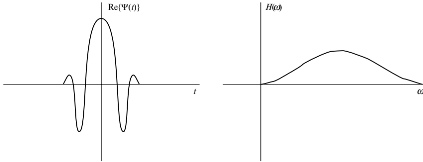
Рис. 3.9. Модифицированная гауссова, или морлетовская, материнская вейвлетная функция \Psi(t) и ее Фурье-образ H(\omega)
