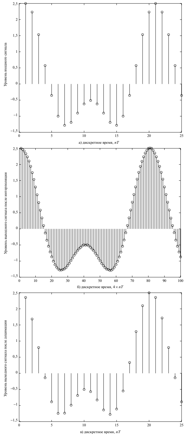
Рис. 9Б.1. Входной сигнал (панель а). Иллюстрация интерполяции с шагом 4 (панель б). Иллюстрация децимации с шагом 4 (панель в)
