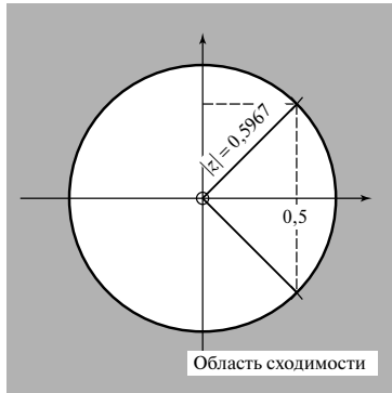
Рис. 4.4. Контур интегрирования, показывающий область сходимости (пример 4.8)
