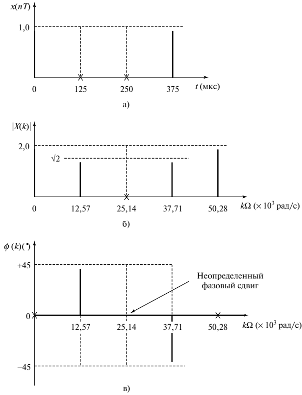
Рис. 3.3. График зависимости x(nT) от t (панель а), график зависимости |X(k)| от k (панель б); график зависимости \phi(k) от k (панель в)
