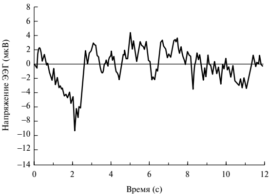
Рис. 11.18. Сигнал CNV пациента с болезнью Хантингтона после предварительной обработки и усреднения
