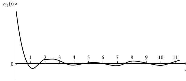
Рис. 5.5. Автокорреляционная функция случайного сигнала
