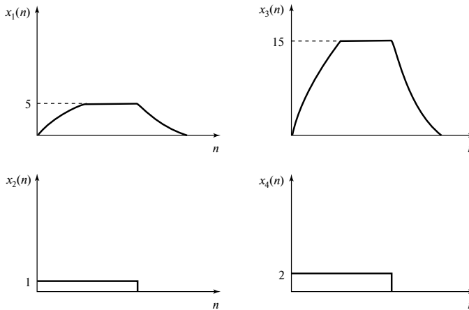
Рис. 5.4. Пары сигналов \{x_1(n), x_2(n)\} и \{x_3(n), x_4(n)\} различных амплитуд, но с равными взаимными корреляциями
