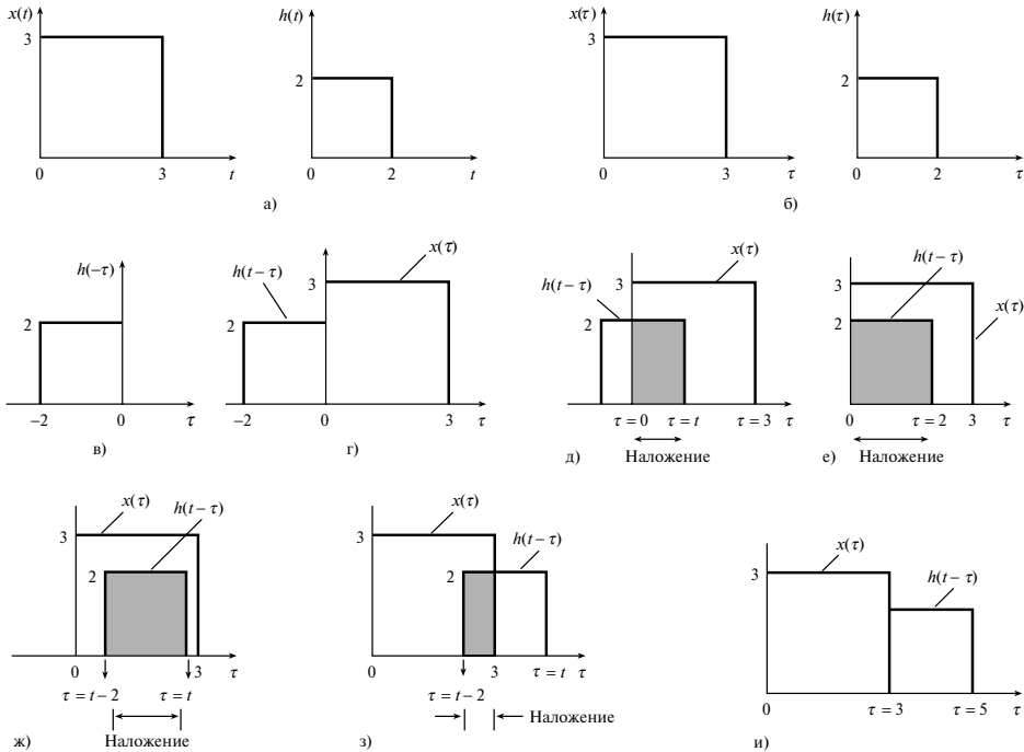
Рис. 5.21. Аналитическая свертка: а) сигналы x(t) и h(t) ; б) x(\tau) и h(\tau) ; в) h(-\tau) ; г) h(t-\tau) и x(\tau) ; t < 0 , сигнал h(t-\tau) не накладывается на x(\tau) ; д) h(t-\tau) и x(\tau) ; 0 < t \leq 2 , первое частичное наложение h(t-\tau) и x(\tau) ; е) h(t-\tau) и x(\tau) ; t = 2 , конец первого частичного наложения; ж) h(t-\tau) и x(\tau) ; 2 \leq t \leq 3 , полное наложение h(t-\tau) и x(\tau) ; з) h(t-\tau) и x(\tau) ; 3 \leq t \leq 5 , второе частичное наложение h(t-\tau) и x(\tau) ; и) h(t-\tau) и x(\tau) ; t > 5 , наложения h(t-\tau) и x(\tau) нет
