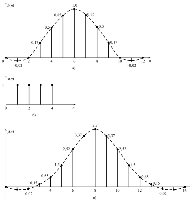
Рис. 1.1. Пример свертки двух последовательностей, y(n) — это свертка h(n) и x(n) . Если рассматривать h(n) как импульсную характеристику системы, то y(n) — это выход системы при входе x(n) . Значения y(n) были получены непосредственно из уравнения (1.1)
