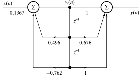
Рис. 4.18. Функциональная схема системы дискретного времени из задачи 4.13
