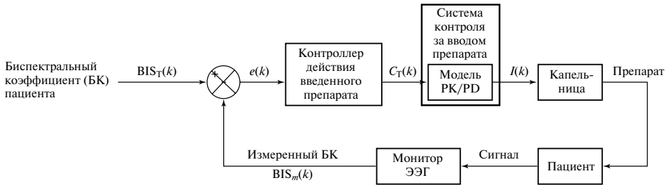
Рис. 1.25. Основанная на ЦОС анестетическая система с регулированием по замкнутому циклу
