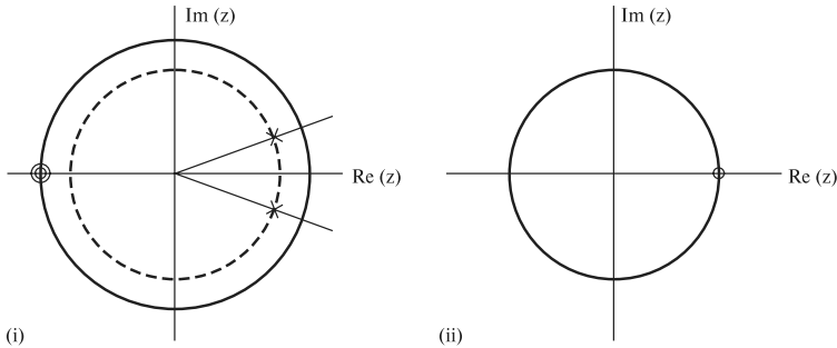
а) диаграмма нулей и полюсов (i) фильтра, (ii) сети с обратной связью по ошибке при k = 1
