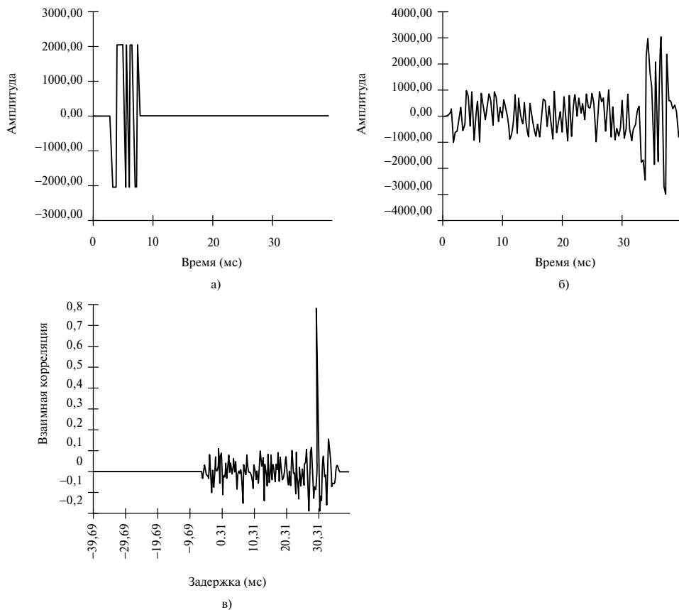
Рис. 1.3. Взаимная корреляция случайного сигнала x(t) с задержанной зашумленной версией того же сигнала y(t) . Задержка между двумя сигналами равна времени от начала отсчета до времени появления максимума их взаимной корреляции на панели в
