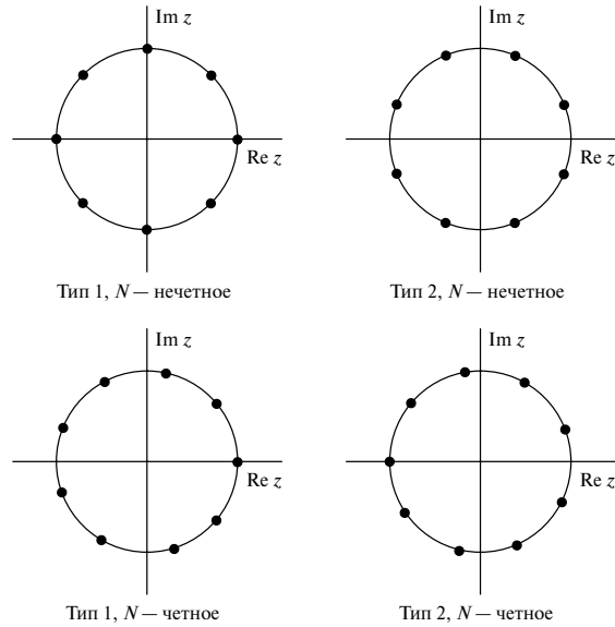
Рис. 7.17. Четыре возможные структуры выборки для двух типов фильтров (изображены на комплексной плоскости)
