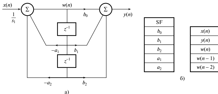
Рис. 12.27. Каноническое звено второго порядка: а) диаграмма реализации; б) память для хранения данных и коэффициентов
