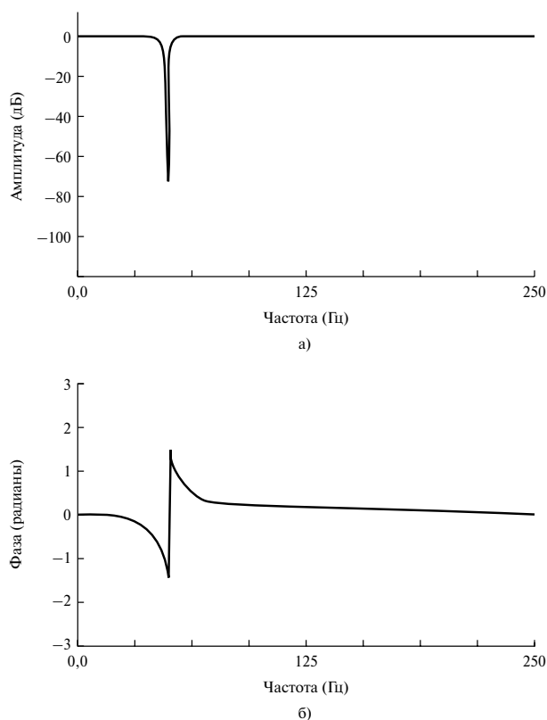
Рис. 4В.1. Амплитудно-частотная характеристика БИХ-системы из примера 4В.1 при непосредственной оценке (панель а ). Фазовая характеристика БИХ-системы из примера 4В.1 при непосредственной оценке (панель б )
