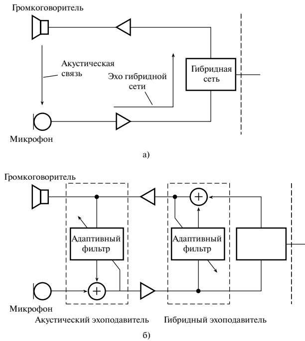
Рис. 10.19. Громкоговорящий телефон (панель а); подавление в громкоговорящем телефоне акустического эха и эха гибридной сети (панель б)
