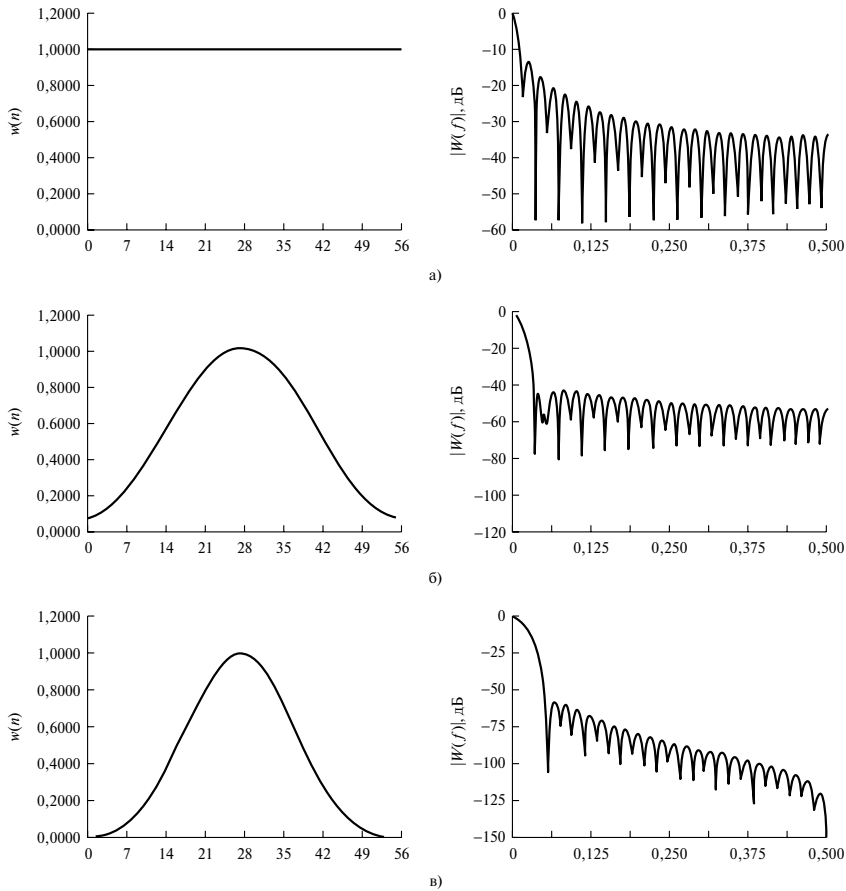
Рис. 7.7. Сравнение характеристик распространенных весовых функций во временной и частотной областях: а) прямоугольная функция; б) функция Хэмминга; в) функция Блэкмена
