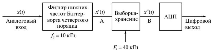
Рис. 2.8. Устройство предварительной обработки данных системы ЦОС реального времени
