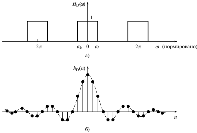
Рис. 7.4. Идеальная частотная характеристика фильтра нижних частот (панель а). Импульсная характеристика идеального фильтра нижних частот (панель б)
