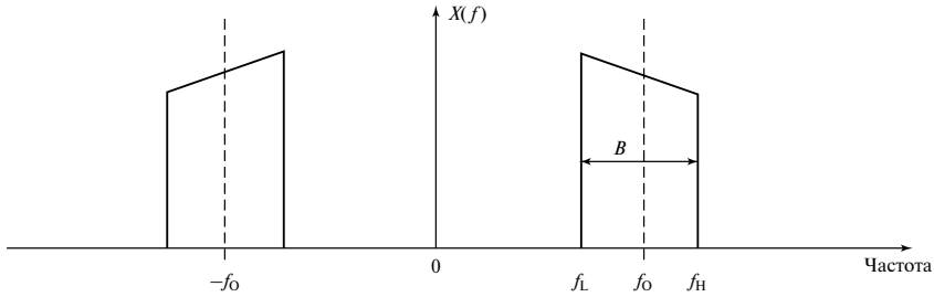
Рис. 2.17. Полосовой сигнал
