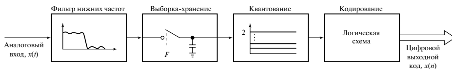
Рис. 2.2. Графическое представление процесса преобразования аналогового сигнала в цифровой
