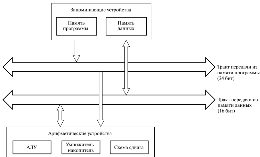
Рис. 12.18. Упрощенная архитектура процессора ЦОС с фиксированной запятой второго поколения (Analog Devices ADSP2100)
