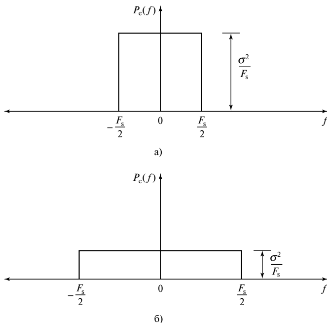
Рис. 2.30. Спектральная плотность мощности шума квантования: а) для преобразования с частотой Найквиста; б) для выборки с запасом по частоте. (Общая мощность шума одинакова в обоих случаях, но при выборке с запасом по частоте мощность шума распределяется по намного большему частотному диапазону, что приводит к снижению уровня мощности шума в полосе)
