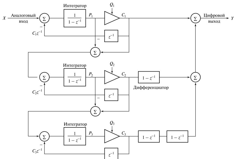
Рис. 2.35. Модель сигма-дельта-модулятора MASH третьего порядка на z -плоскости
