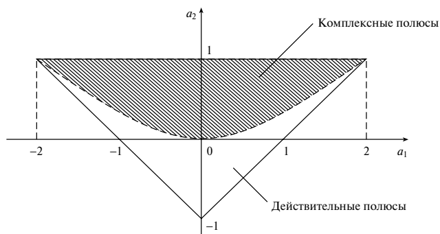
Рис. 13.5. Треугольник устойчивости, показывающий значения коэффициентов фильтра a_1 и a_2 , при которых фильтр устойчив
