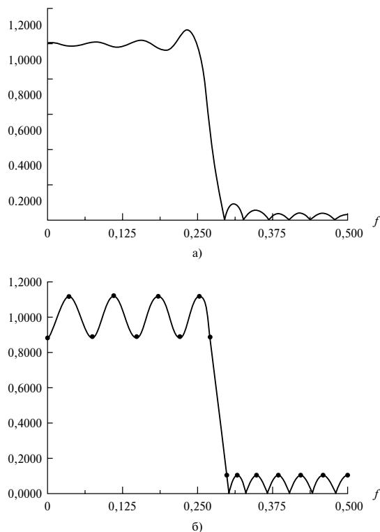
Рис. 7.10. Сравнение частотных характеристик: а) фильтра, полученного методом вырезания, б) оптимального фильтра. На панели а колебания характеристики больше на границе полосы; а на панели б колебания имеют равные амплитуды (полосы равных колебаний) в полосе пропускания и подавления
