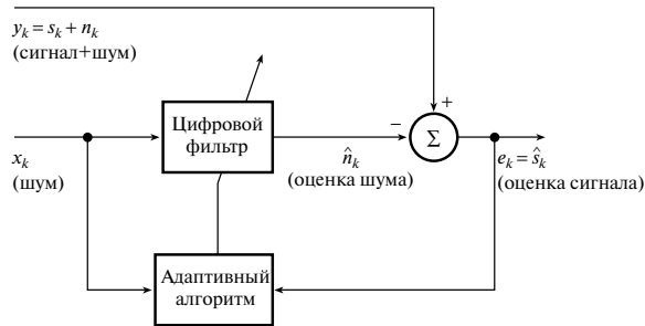
Рис. 10.2. Блок-схема адаптивного фильтра-шумоподавителя
