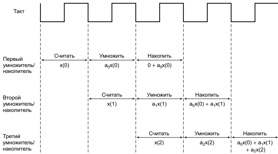
Рис. 12.9. Временная диаграмма блока умножителя-накопителя с конвейерной обработкой. При заполненном конвейере операция в блоке завершается каждый такт (200 нс)
