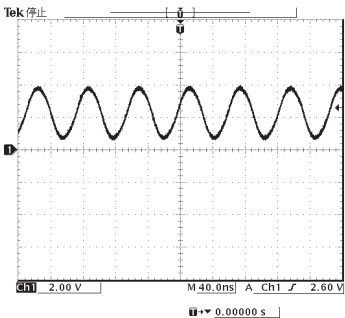
POINT A XL601 (Pin 13 of IC602)
