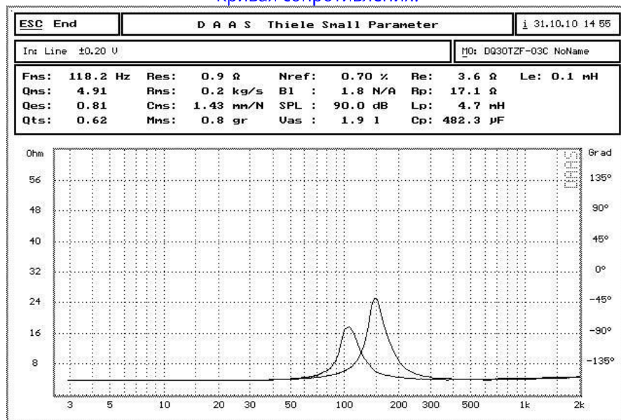
Кривая сопротивления:
