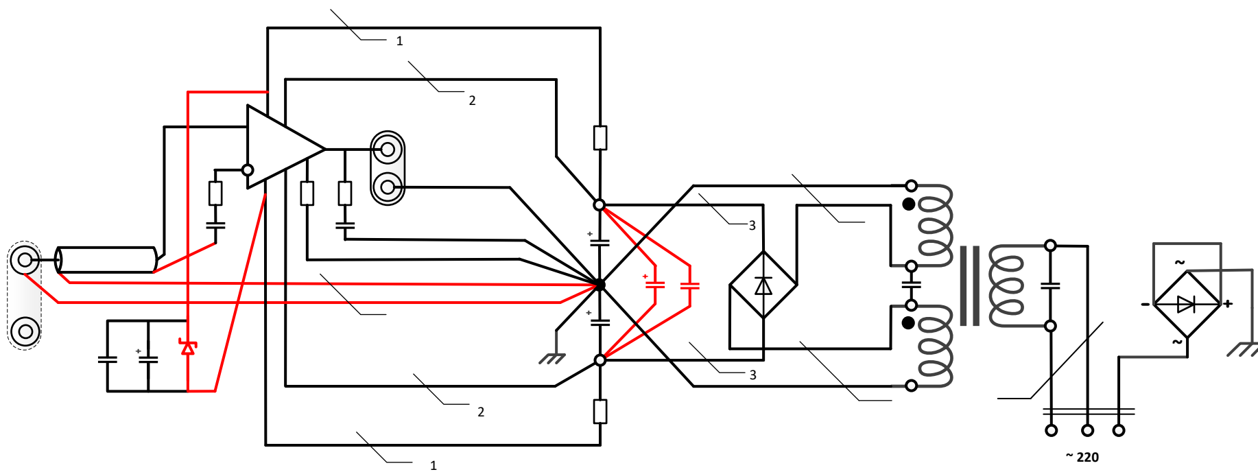
Схема разводки земли и питания УМЗЧ
