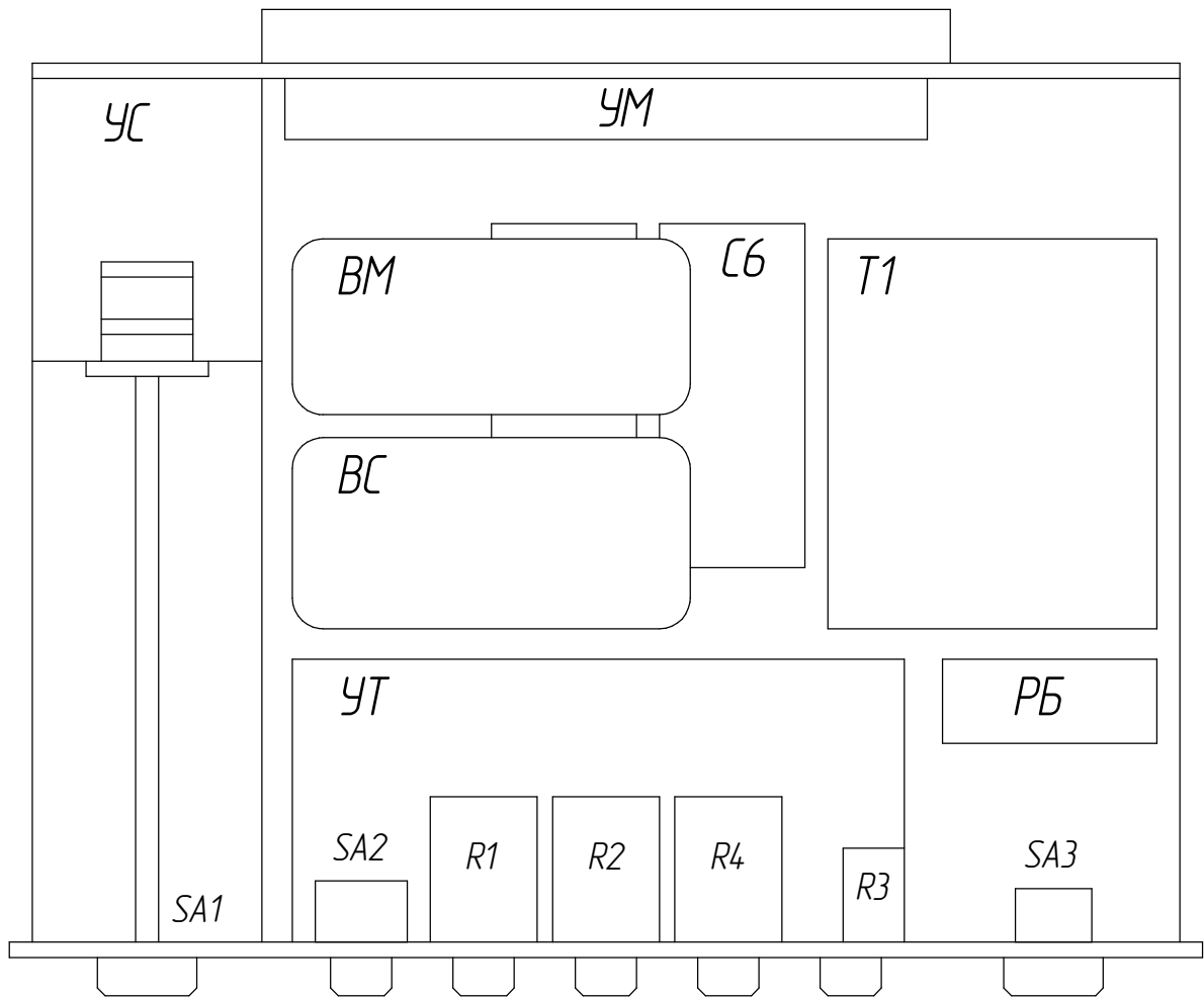
Расположение основных элементов и плат
