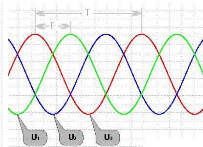
Осциллограммы фазовых напряжений обмоток U_1, U_2, U_3 – напряжения обмоток; T – период сигнала (360 градусов); F – фаза смещения (120 градусов).
