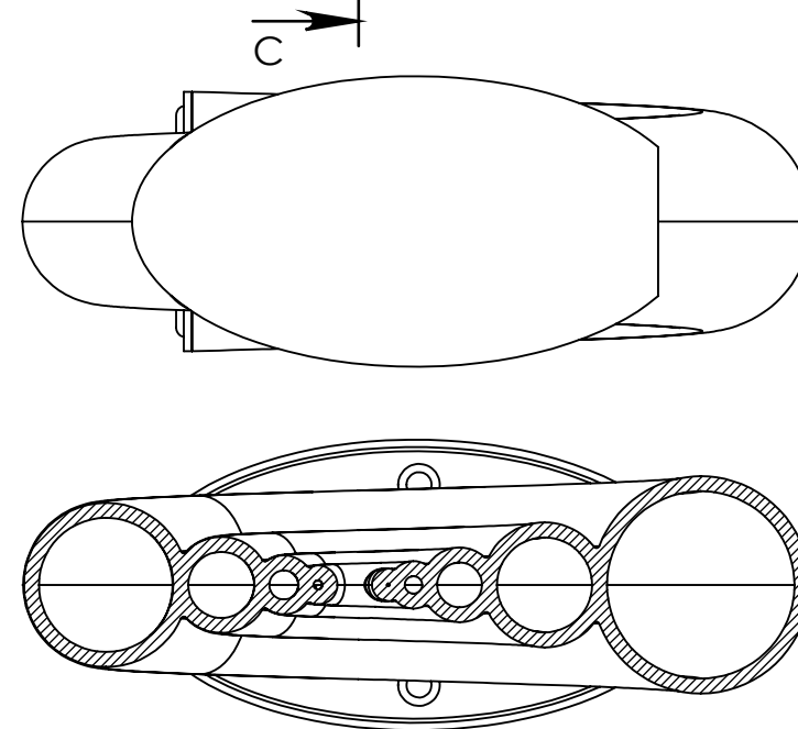
B-B SCALE 1 : 10
