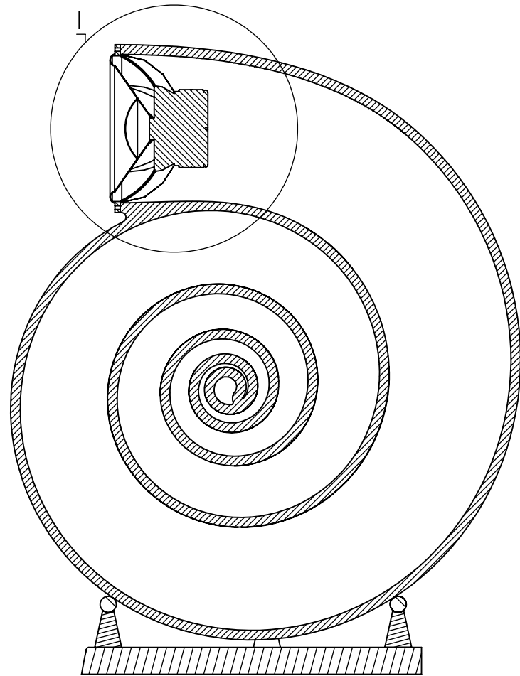
A-A SCALE 1 : 10
