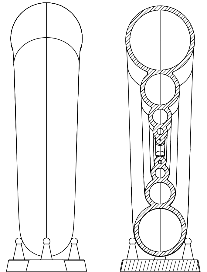
C-C SCALE 1 : 10
