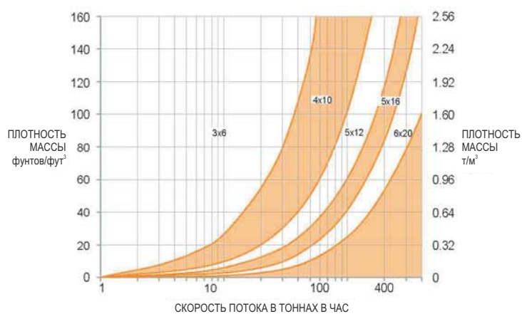
Производительность вертикального потоконаправителя подачи
