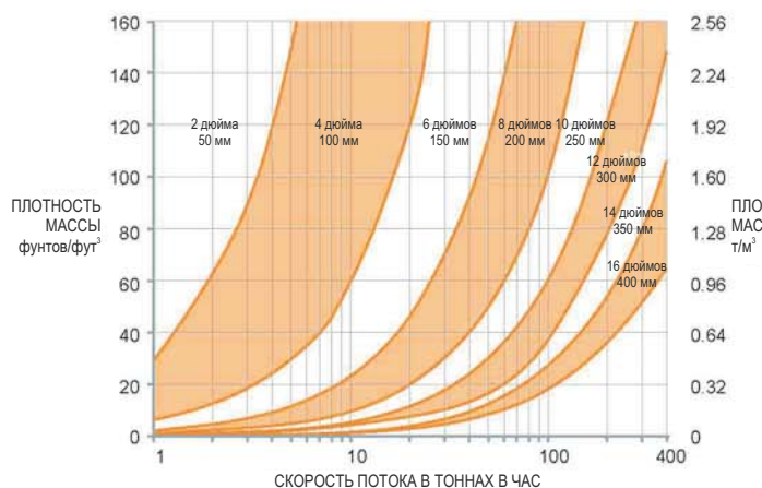
Производительность кругового потоконаправителя подачи
