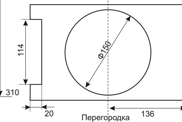
Задняя панель верхняя часть
