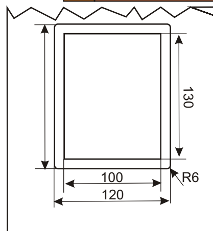
Задняя панель вырез под площадку терминала
