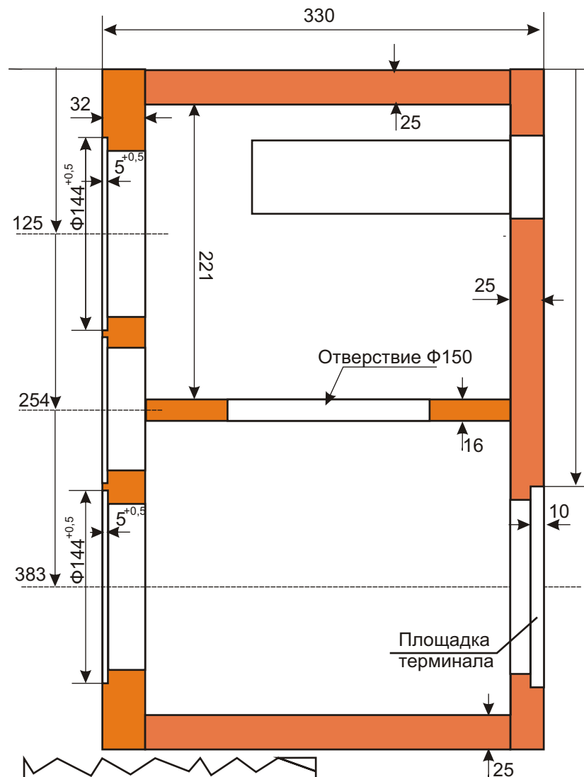
Задняя панель верхняя часть
