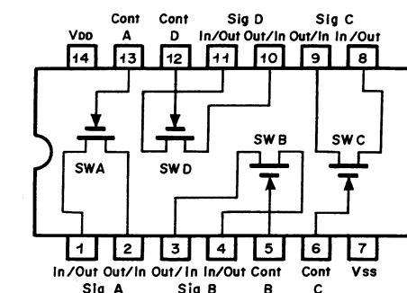
Fig. 13.6 Bilateral Switch C-MOS IC MSM4066RS
