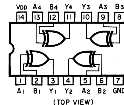
Fig. 13.9 Exclusive OR Gate C-MOS IC \mu PD4030BC
