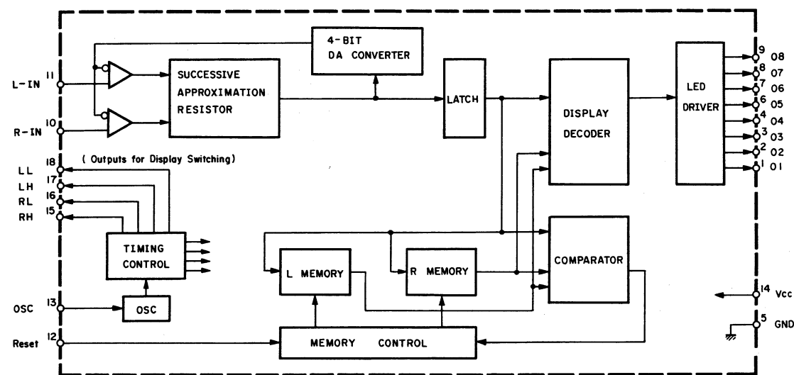
Fig. 13.11 Level Meter Control IC MSL9350RS
