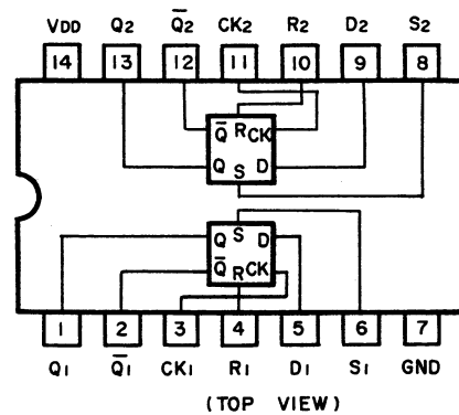
Fig. 13.10 D-Type Flip-Flop C-MOS IC TC4013BP
