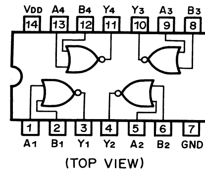
Fig. 13.7 NOR Gate C-MOS IC \mu PD4001BC
