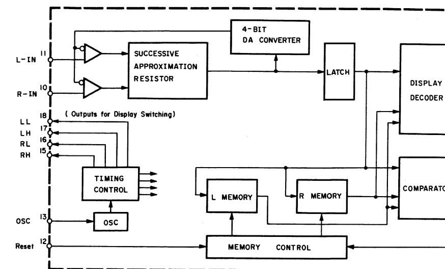
Fig. 13.11 Level Meter Control IC MSL9350RS
