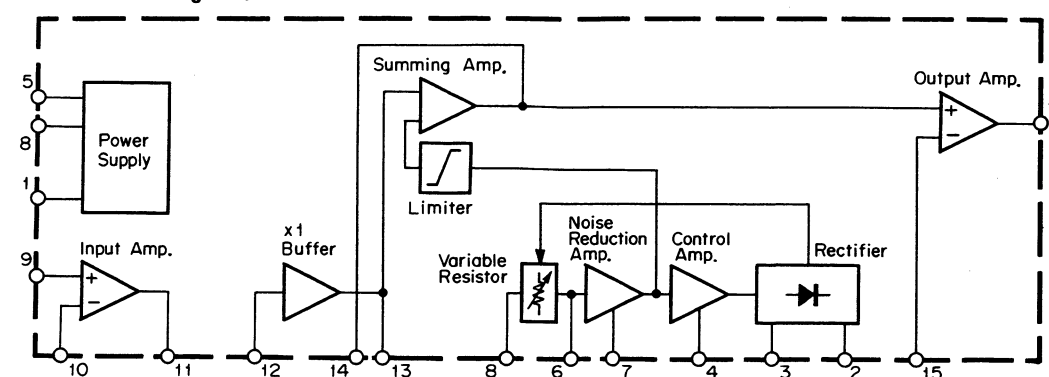
Fig. 13.4 Dolby NR IC \mu A7300PC, LA2730
