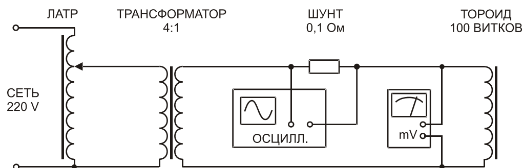
Рис. 1. Схема измерения.
