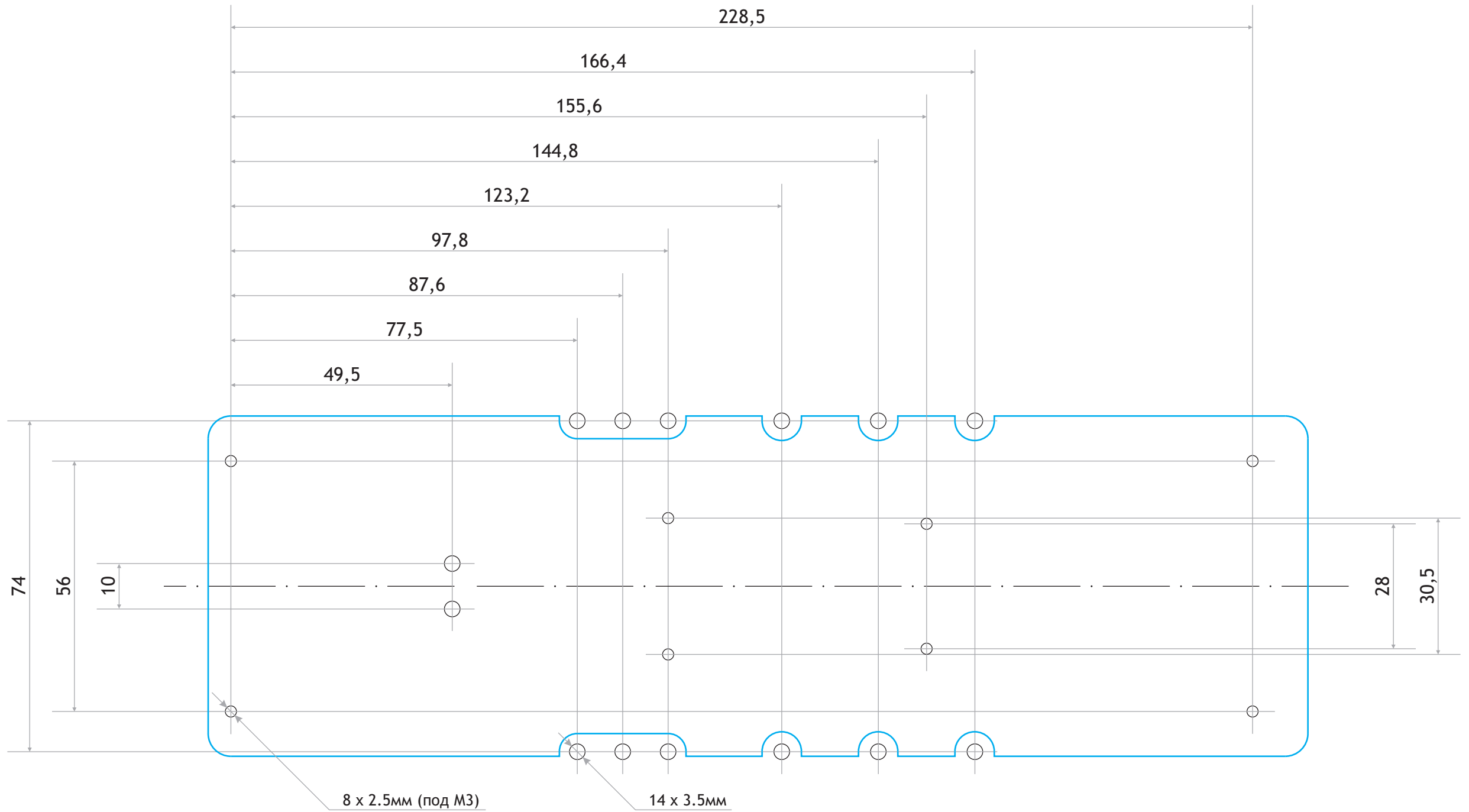
Разметка радиатора (WP тк II v1.21 PCB) by ~D'Evil~
