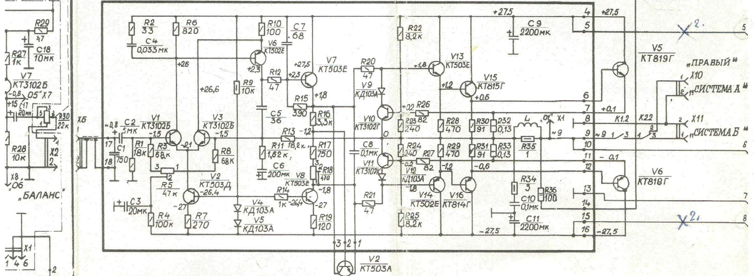
А7 Усилитель оконечный
