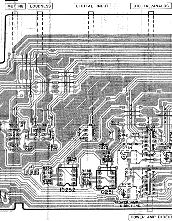
G SWITCH P.C.B.
