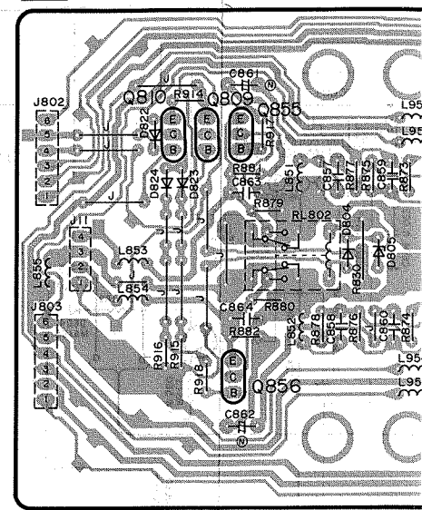
C AUDIO (DIGITAL) AMP P.C.B.
