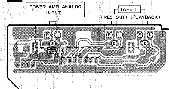
G SWITCH P.C.B.
