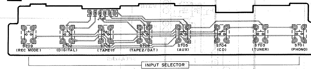
I INPUT SELECT SWITCH P.C.B.
