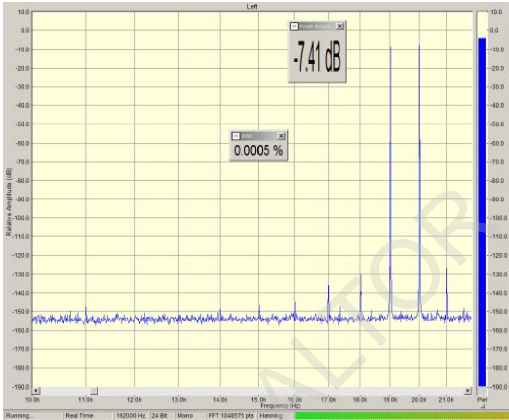
IMD 19/20kHz -7dB/-7dB 44.1kHz SPDIF
