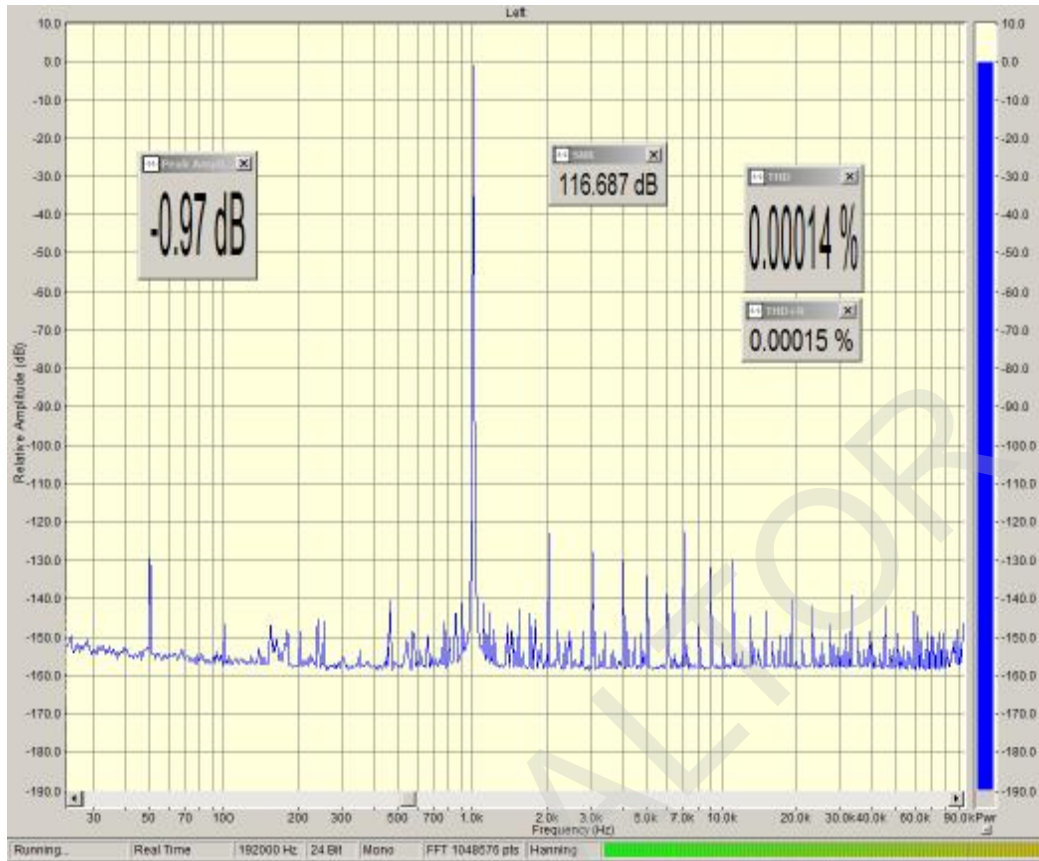
THD 1kHz 0dB 384kHz USB
