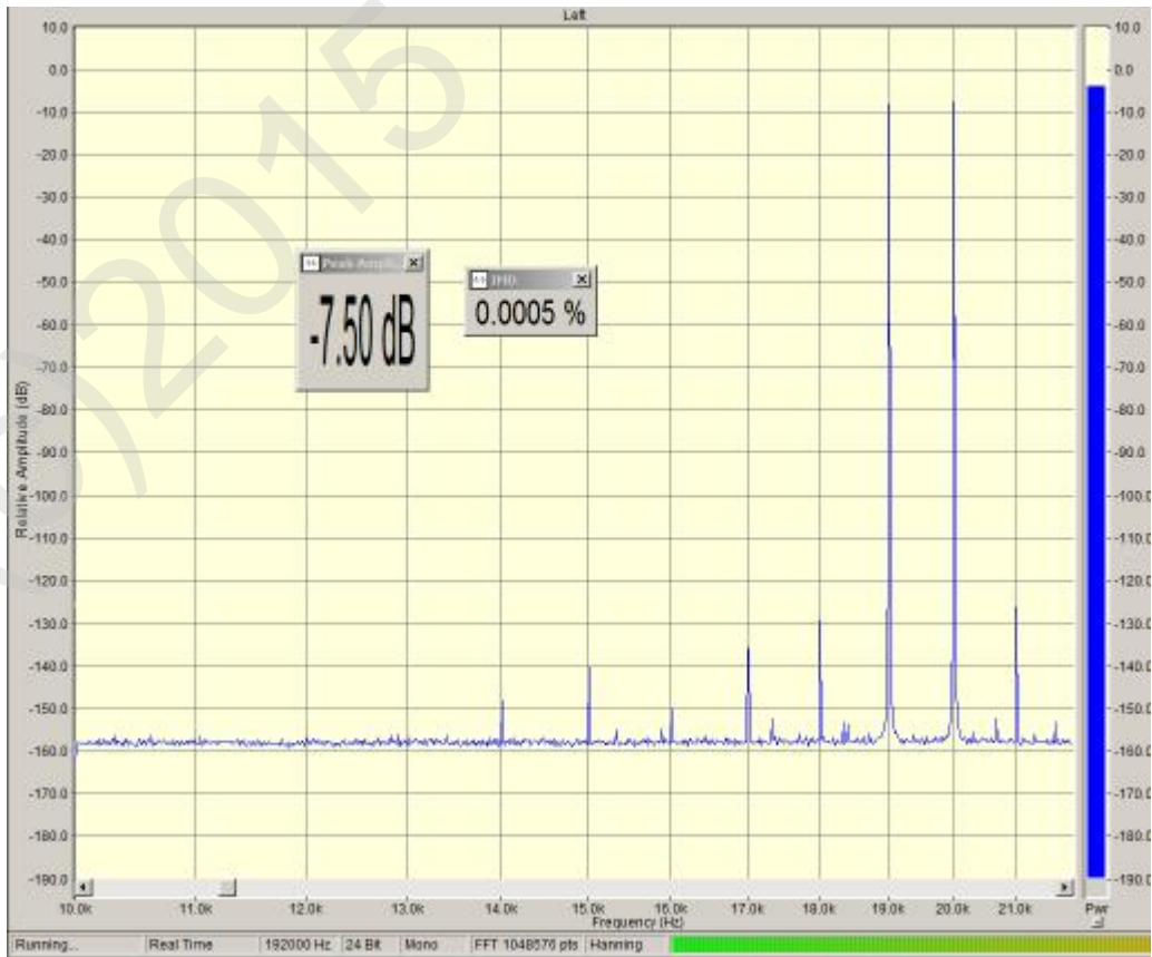
IMD 19/20kHz -7dB/-7dB 44.1kHz USB
