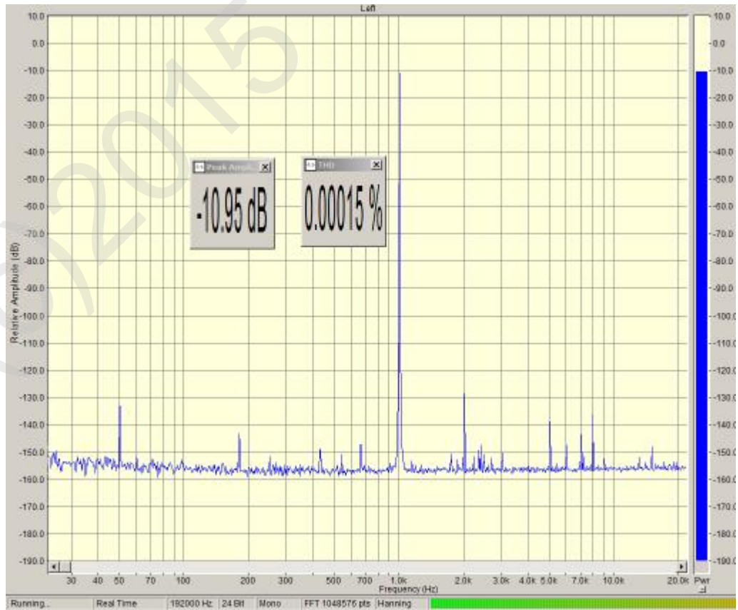
THD 1kHz -10dB 44.1kHz SPDIF
