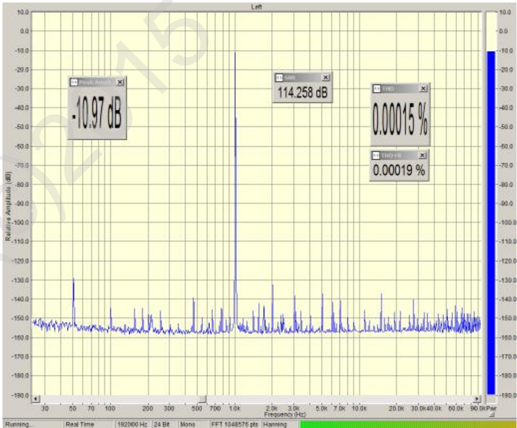
THD 1kHz -10dB 384kHz USB
