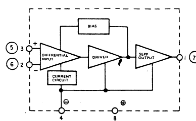
M54565P (Mitsubishi)
