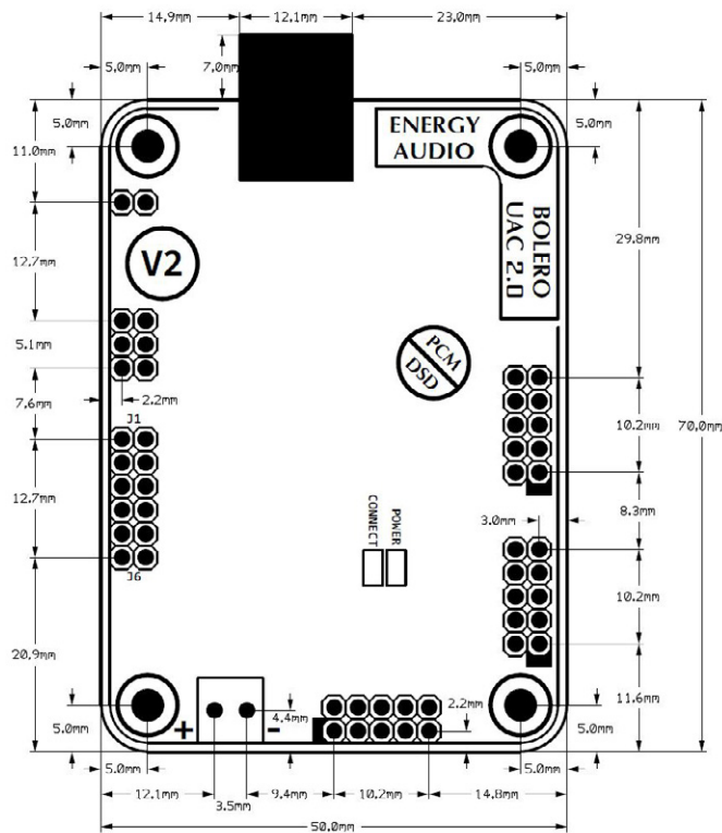
Вид сверху.
