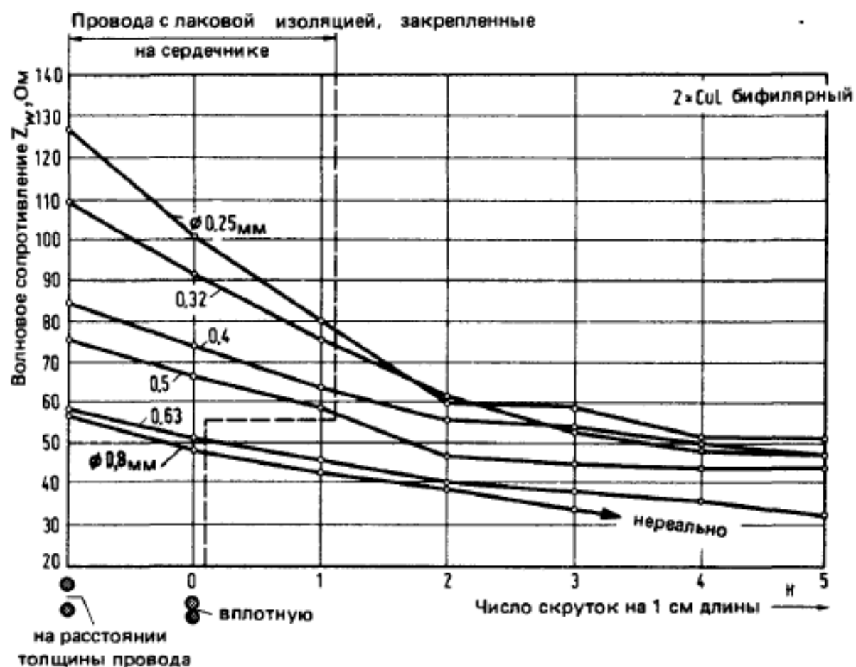
Рис. 6.3 Зависимость импеданса (волнового сопротивления) двухпроводной линии от толщины проводов и их взаимного расположения.
