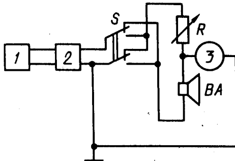
1 — генератор ГНИ; 2 — усилитель мощности У1; 3 — электронный вольтметр; R — магазин сопротивлений; BA — контролируемый громкоговоритель; S — переключатель
