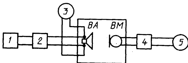
1 – генератор ГНИ; 2 – усилитель мощности У1; 3 – электронный вольтметр; 4 – микрофонный усилитель УМ; 5 – измеритель нелинейных искажений ИНИ; ВА – контролируемый громкоговоритель; ВМ – измерительный микрофон
