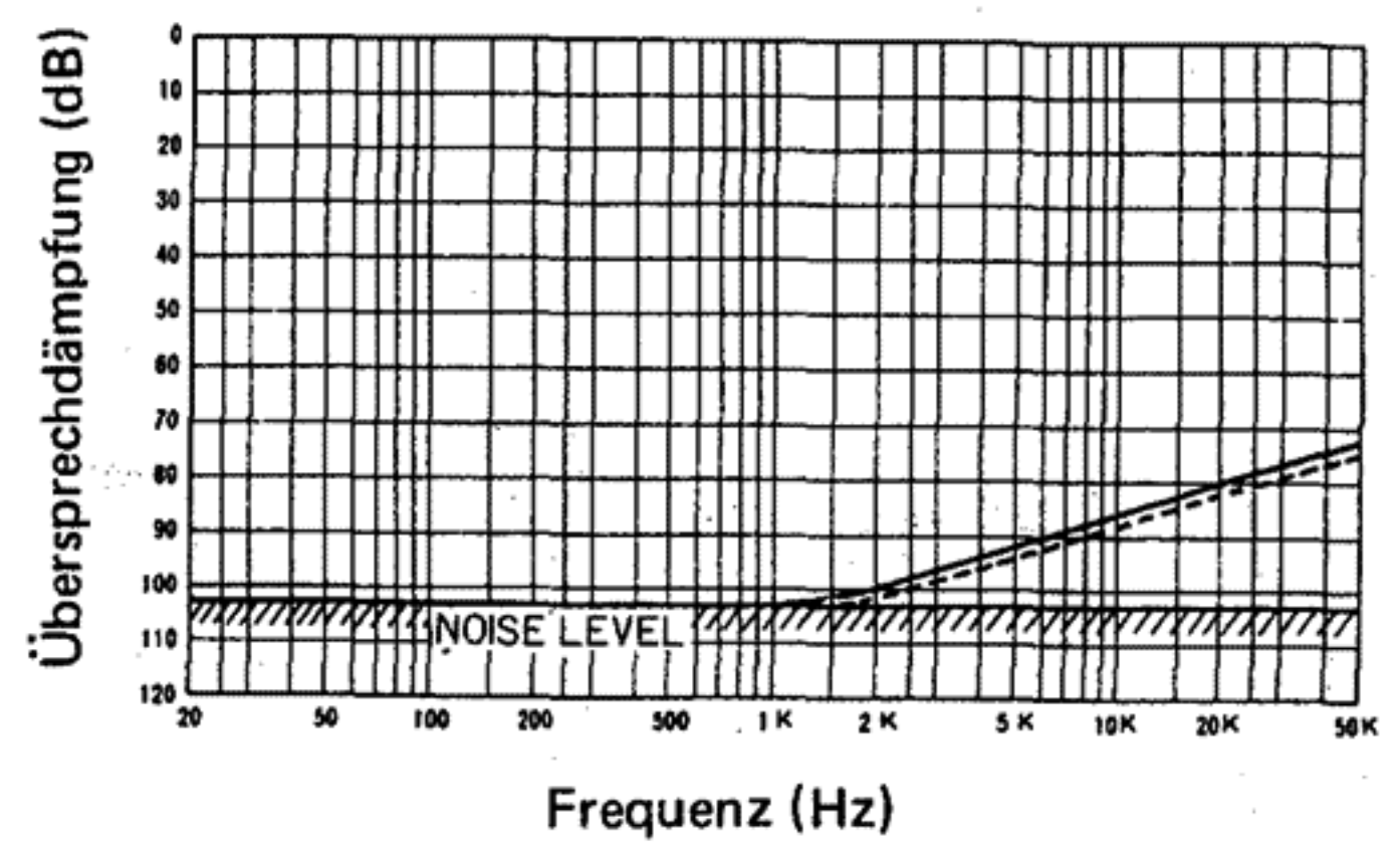
Übersprechdämpfung in Abhängigkeit von der Frequenz.
