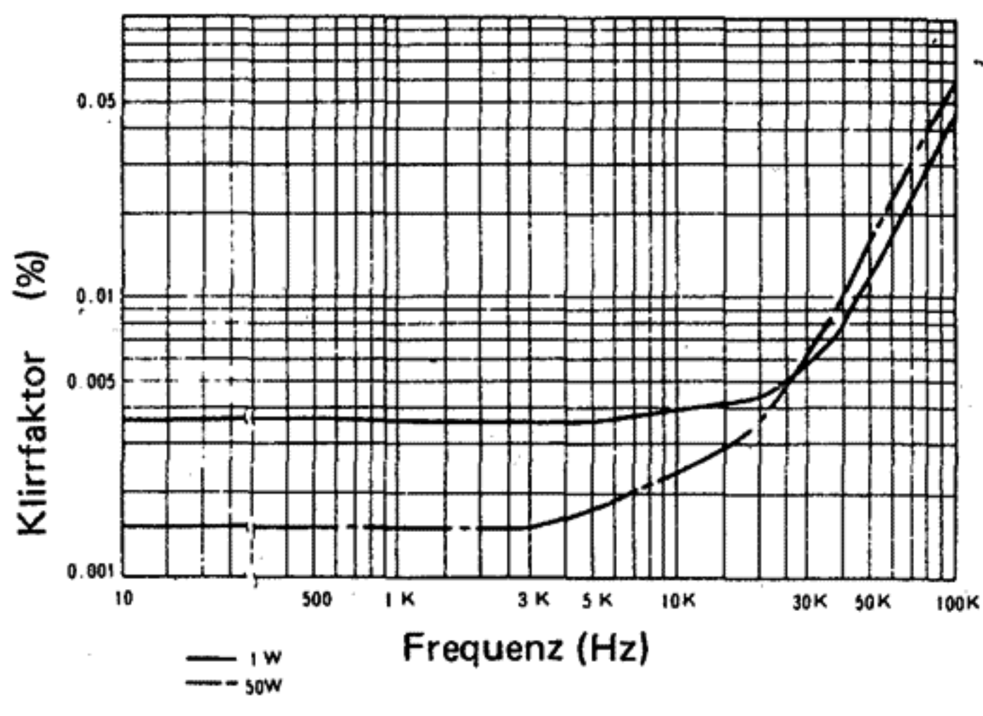
klirr in Abhängigkeit von der Frequenz (8 Ohm, beide Kanäle ausgesteuert)
