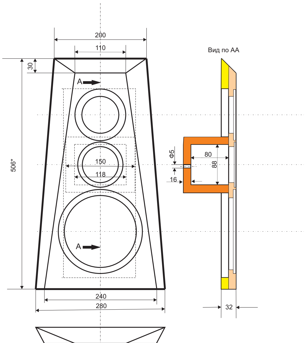
Передняя панель в сборе. МДФ16мм.
