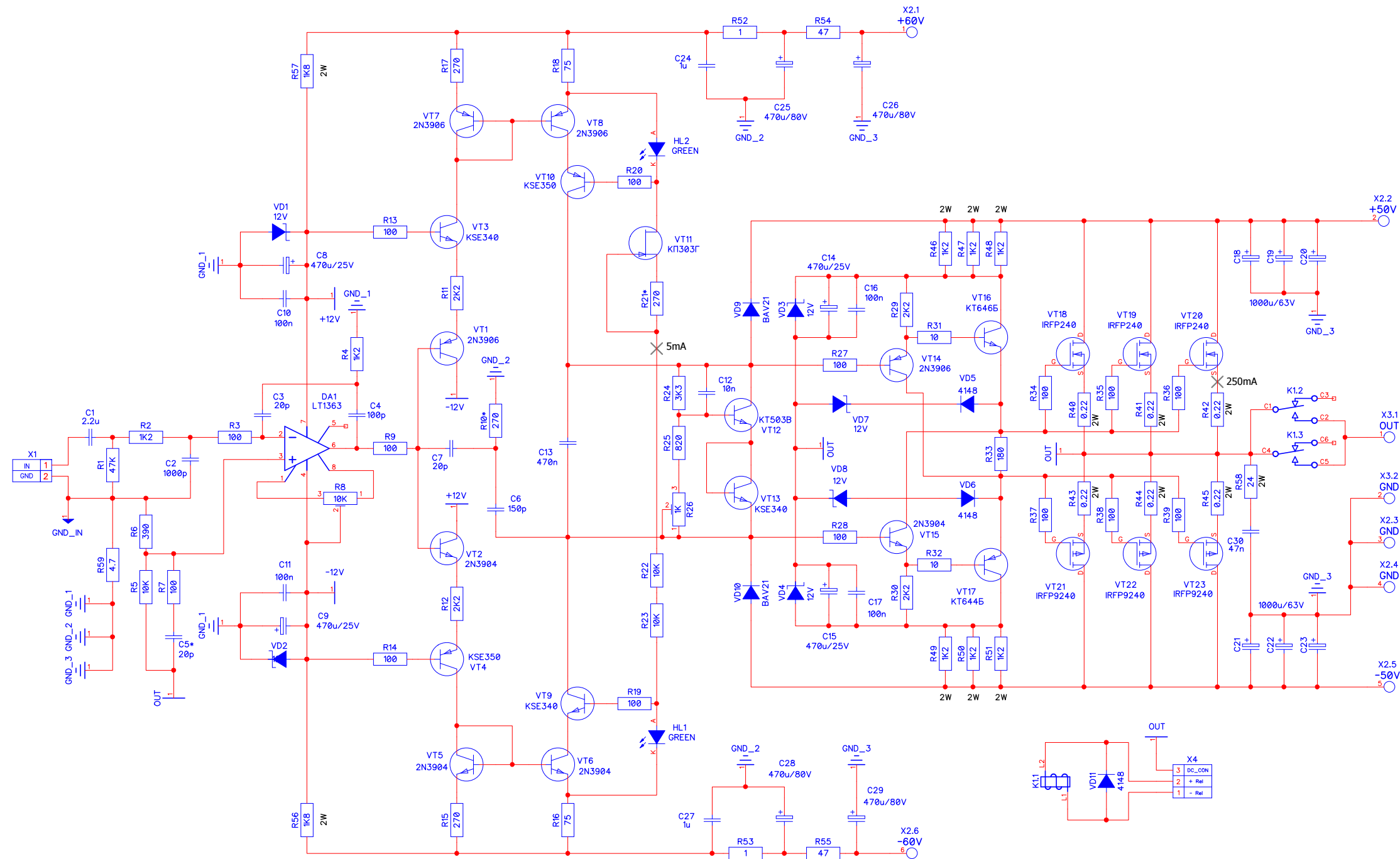
Рис.1 Схема усилителя мощности
