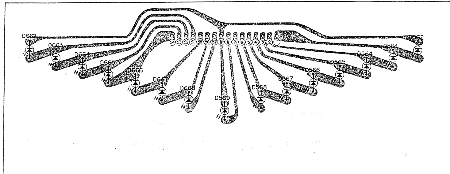
Anzeige-Leiterplatte
