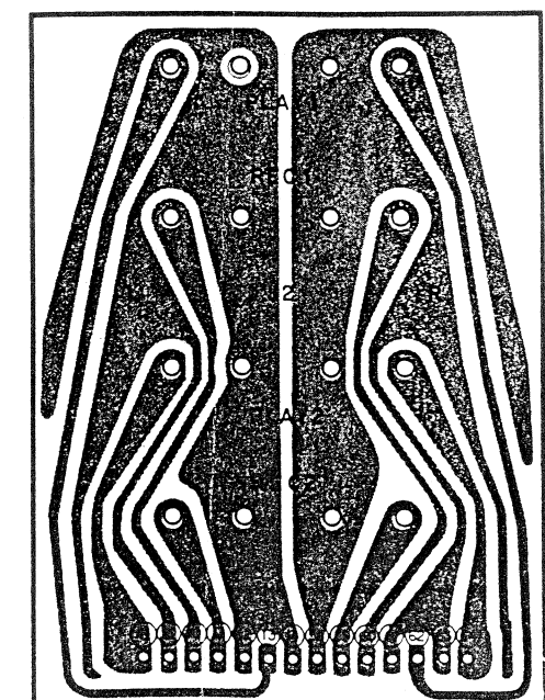
Tonbandgerät-Leiterplatte
