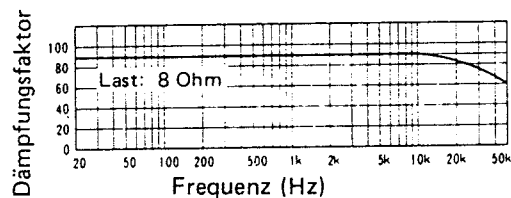
Dämpfungsfaktor
