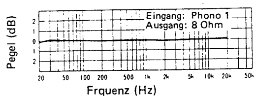
Abweichung von der RIAA-Entzerrungskurve
