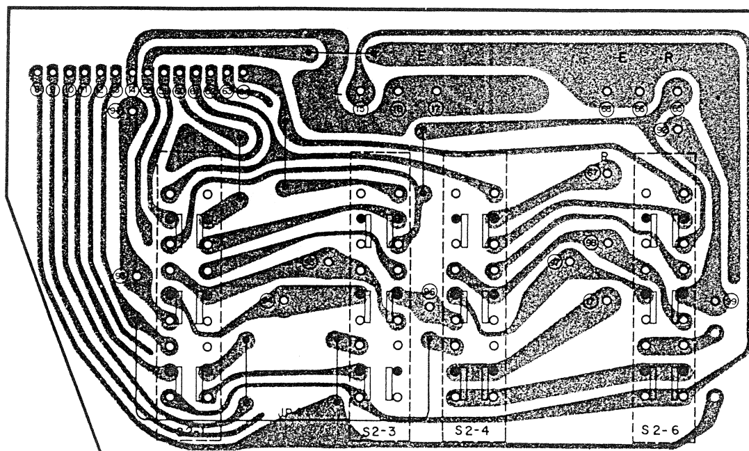
Kopierschaltungs-Leiterplatte
