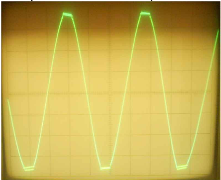
Ограничения выходного напряжения.
