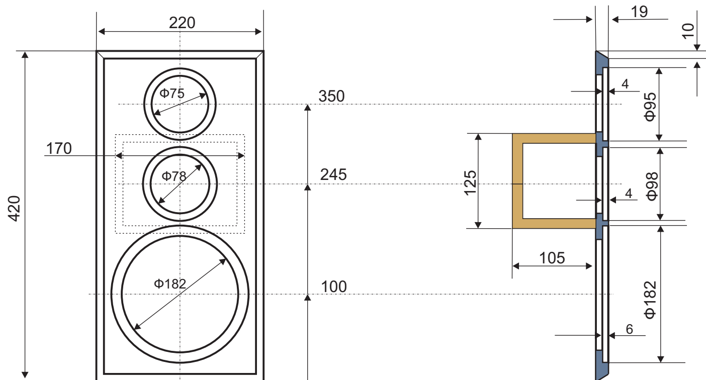
Передняя панель, МДФ 19 мм.
