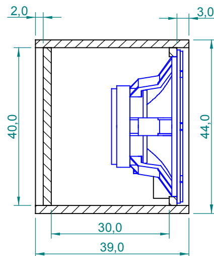
Corte A-A
