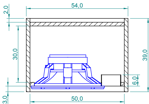
Corte B-B
