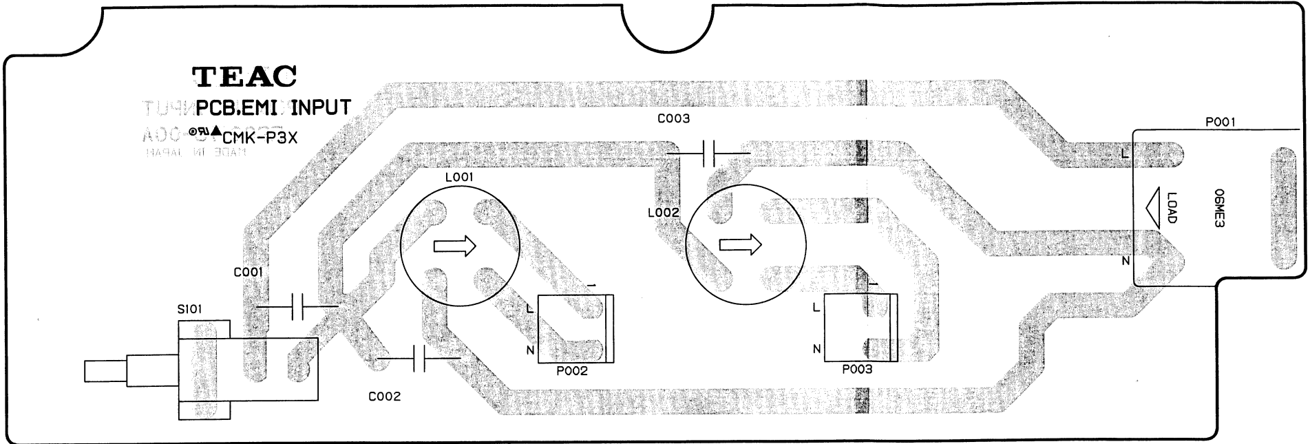
EMI INPUT PCB
