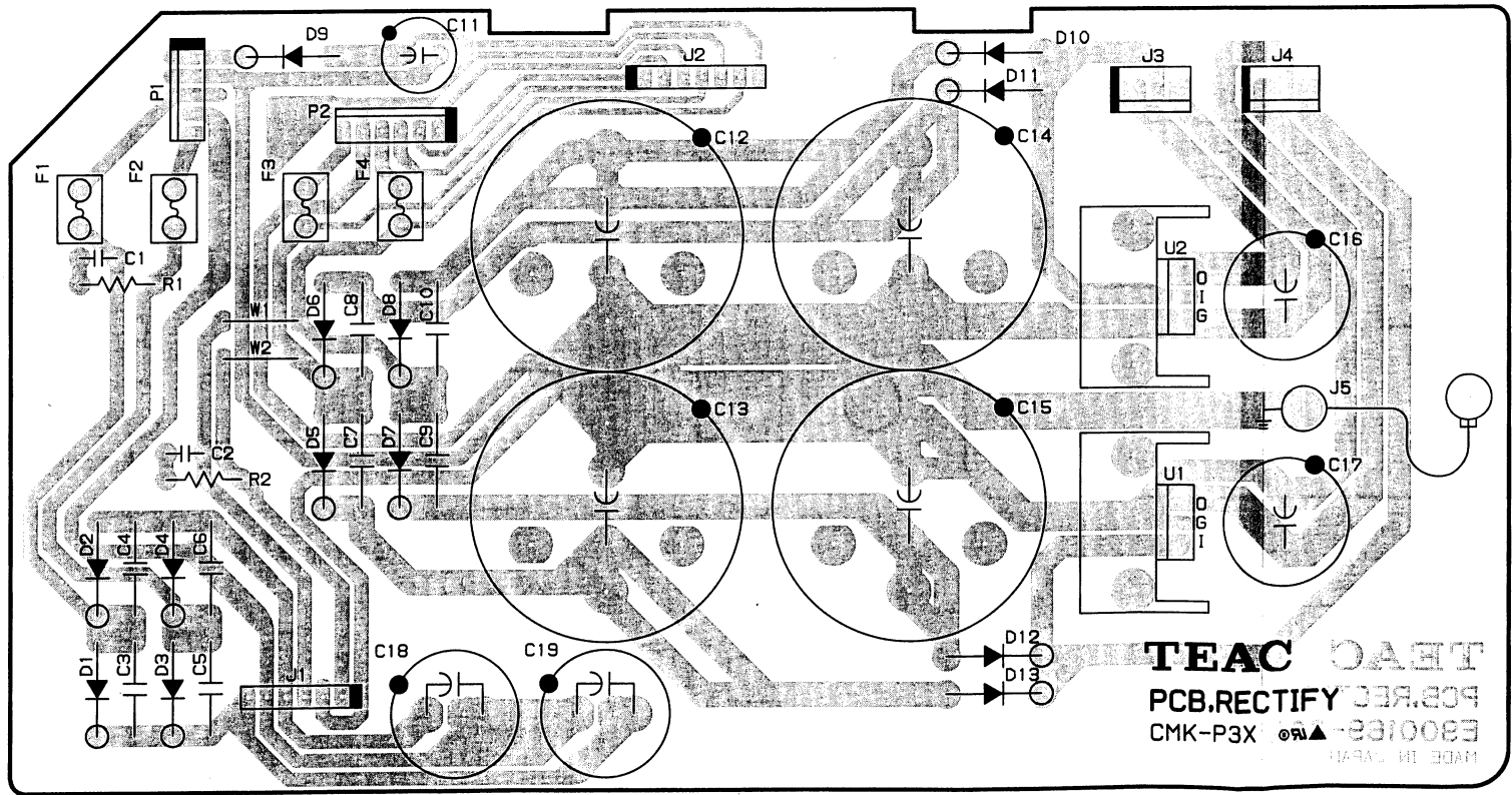
RECTIFY PCB
